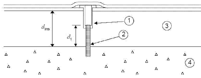
1 : kunststof kap – 2 : verzonken bevestiging – 3 : isolatielaag – 4 : dakplaat
