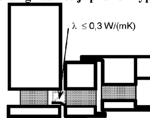
Aansluiting raamstijl-profiel Type C2
