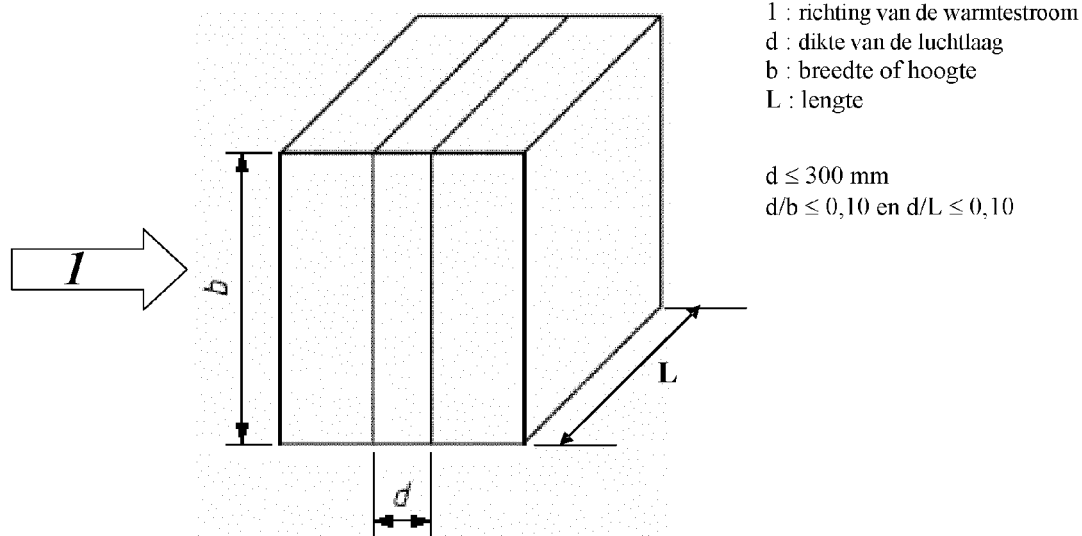
Figuur 1 – Gewone luchtlaag
