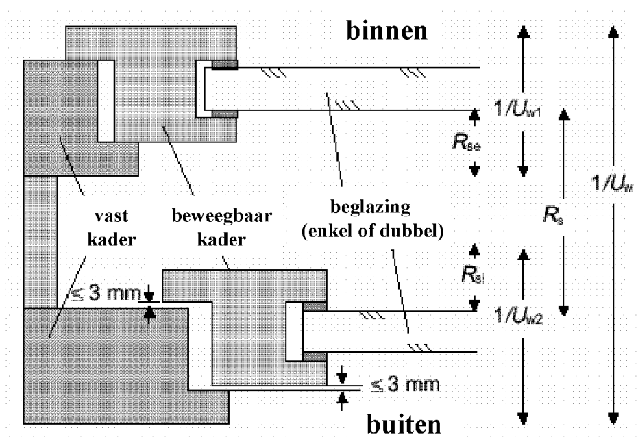
Figuur 14 – Illustratie van een dubbelraam
