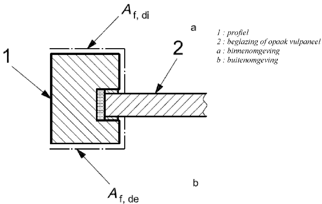
Figuur 11 – Ontwikkelde oppervlakte van raamprofielen
