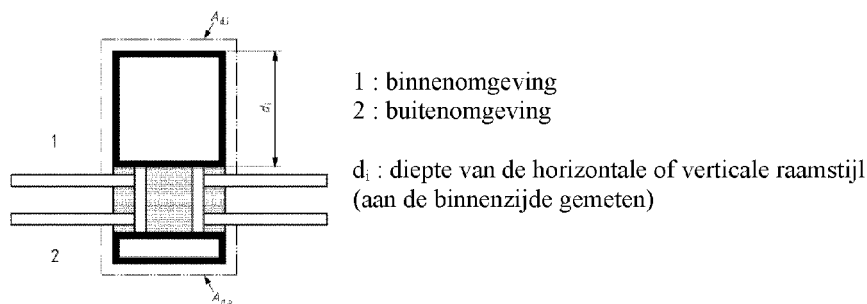
Figuur E.2 – Interne diepte van raamstijlen
