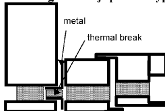
Aansluiting raamstijl-profiel Type A
