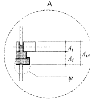
Doorsnede A
