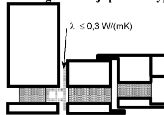
Aansluiting raamstijl-profiel Type B
