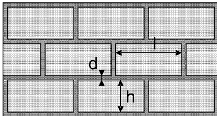
Figuur G.1 – Parameters voor de bepaling van de mortelfractie van metselwerk
