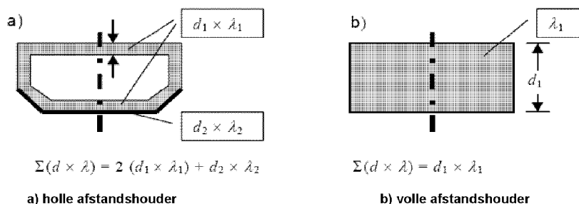
Figuur E.1 – Voorbeelden van de bepaling van het criterium van thermisch verbeterde afstandshouder
