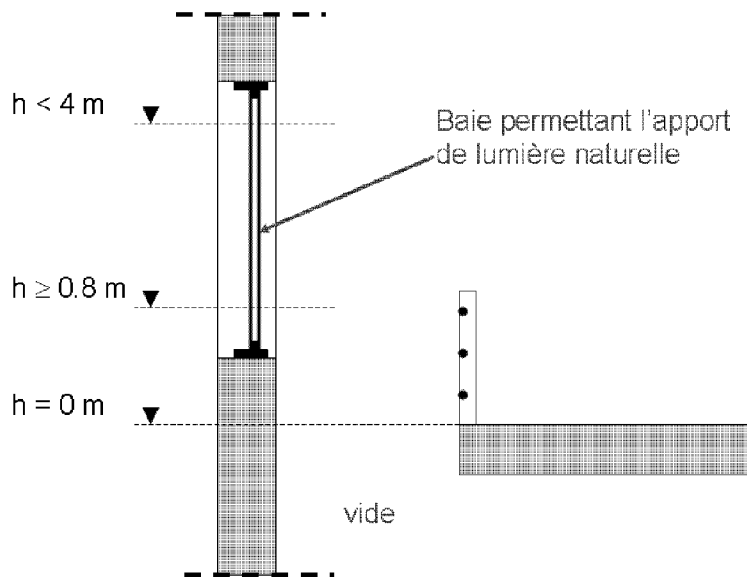
Figuur 1 Projectie van de bovenkant van de vloer op de gevel (bv. bij vides) en begrenzing van de te beschouwen minimale en maximale hoogte van de (equivalente) verticale daglichtopening
