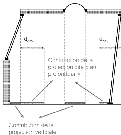
Figuur 2 Bijdragen van de verticale projectie en de diepteprojectie
