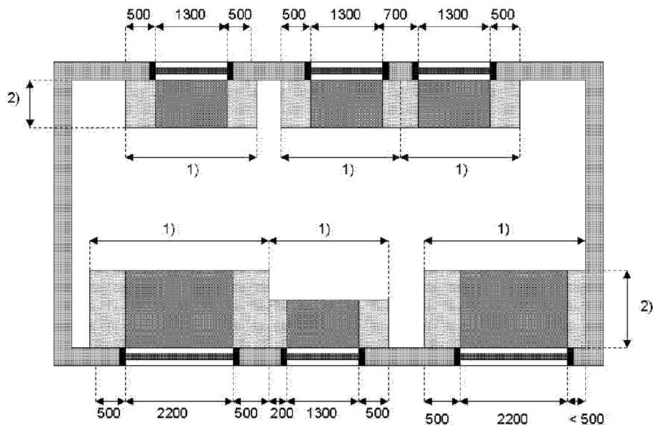
Figuur 3 Deel van de gebruiksoppervlakte achter transparante en niet-transparante geveldelen, dat behoort tot het daglichtdeel
