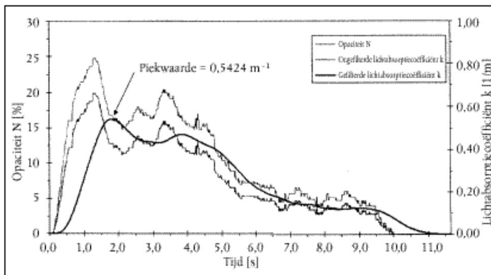
Figuur B Verloop van de gemeten opaciteit N, de ongefilterde lichtabsorptiecoëfficiënt k en de gefilterde lichtabsorptiecoëfficiënt k
