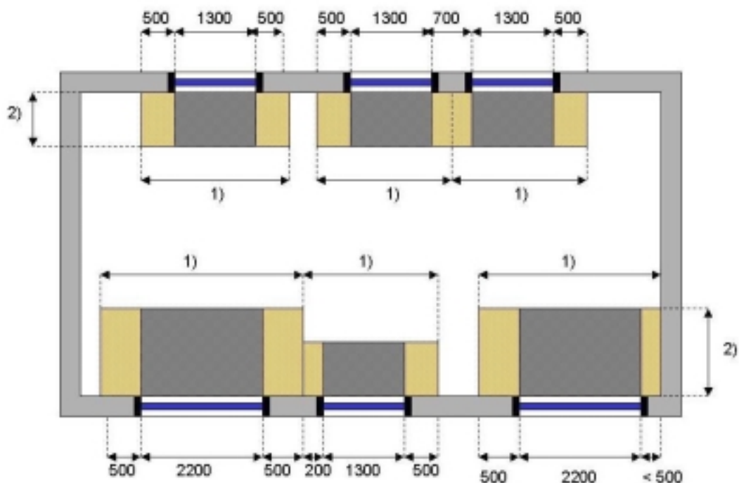
Figuur [6]: Deel van de gebruiksoppervlakte achter transparante en niet-transparante geveldelen dat behoort tot het daglichtdeel
