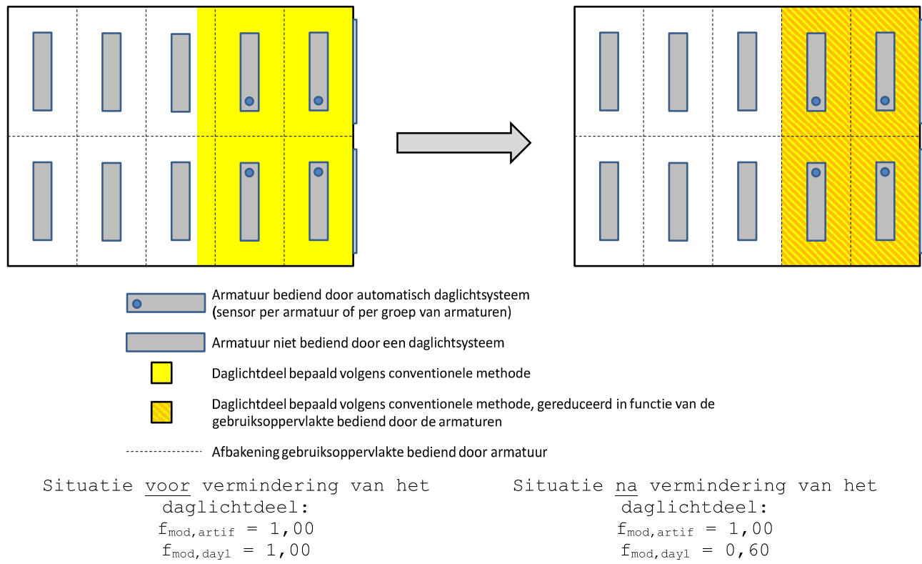
Figuur [3]: Configuratie waarbij niet alle ingerekende armaturen worden bediend door eenzelfde daglichtsysteem – de daglichtoppervlakte ligt deels buiten de gebruiksoppervlakte die bediend wordt door het systeem
