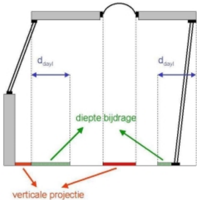
Figuur [5]: Bijdragen van de verticale projectie en van de diepteprojectie
