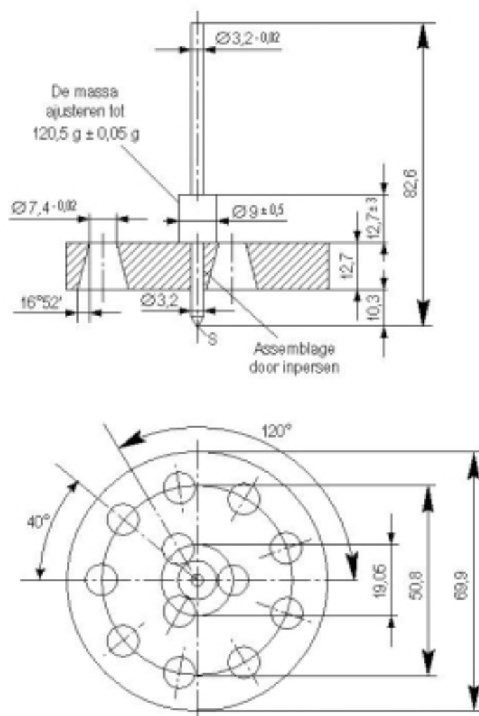
Figuur 1 - Penetrometer
