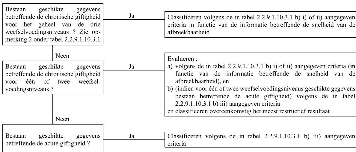
Afbeelding 2.2.9.1.10.3.1 : Categorieën voor de stoffen die gevaarlijk zijn (op lange termijn) voor het aquatisch milieu
