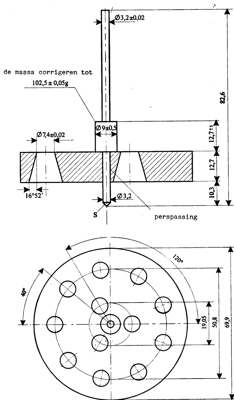
Figuur 1 Penetrometer
