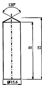
Fig. 2: Cilindervormige bronzen zuiger; afmetingen in mm
