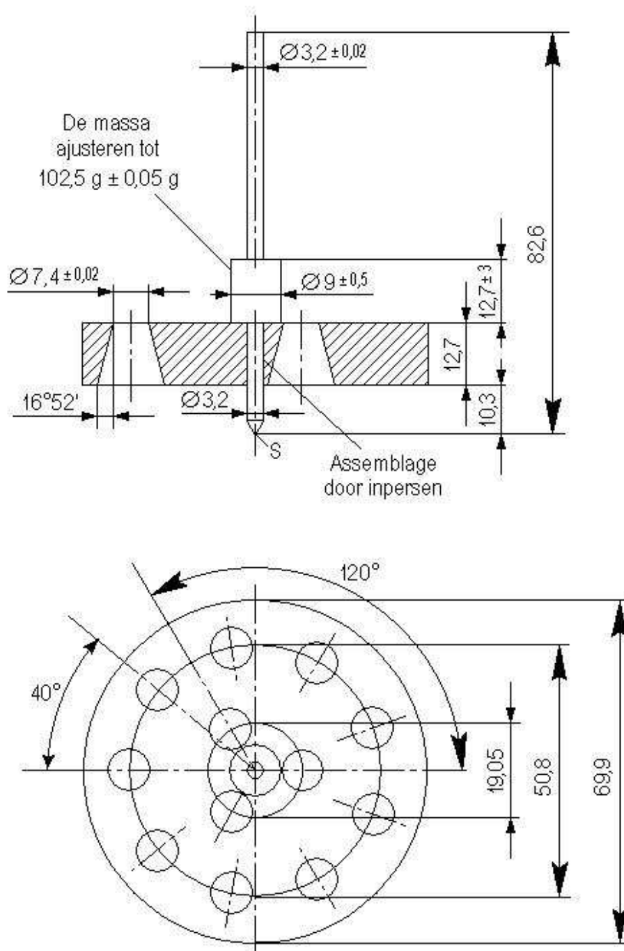
Figuur 1 - Penetrometer
