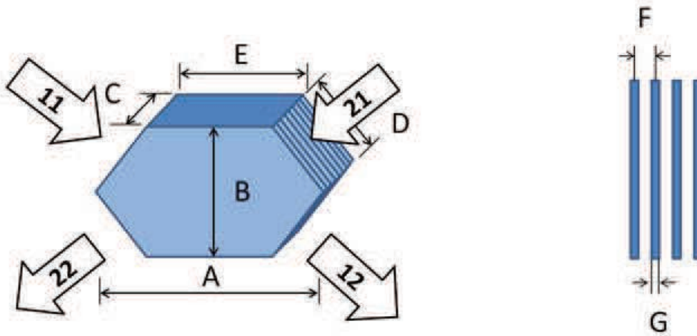
Figuur [6]: Tegenstroomwarmtewisselaar
