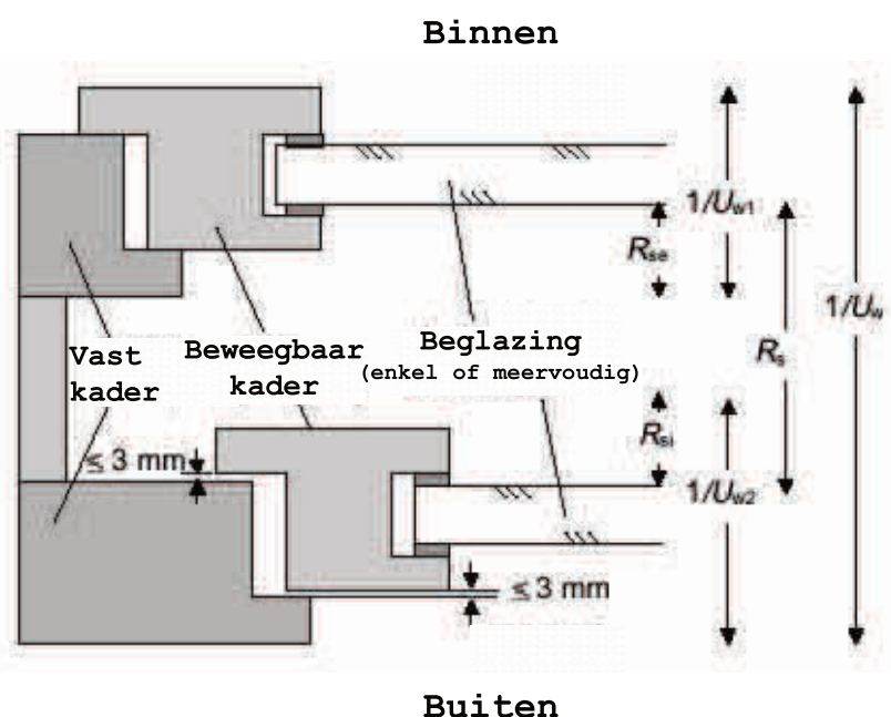
Figuur [16]: Illustratie van een dubbelraam
