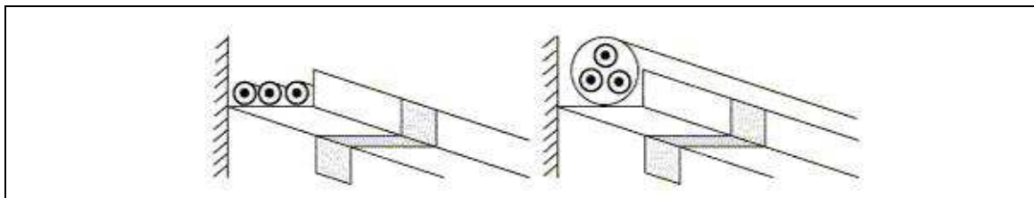
Figuur 5.9. Plaatsingswijzen van elektrische leidingen – Kabelrekken
