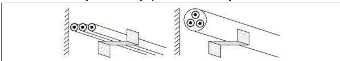
Figuur 5.10. Plaatsingswijzen van elektrische leidingen – Haken
