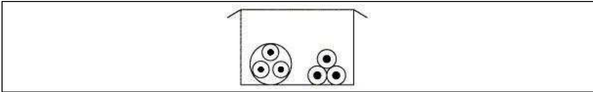
Figuur 5.34. Plaatsingswijzen van elektrische leidingen – Kabelbaan
