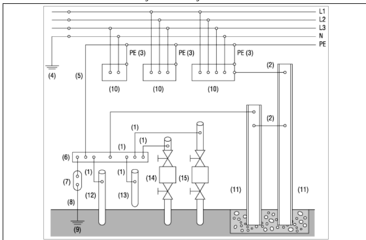
Figuur 2.11. Aardingsinstallatie
