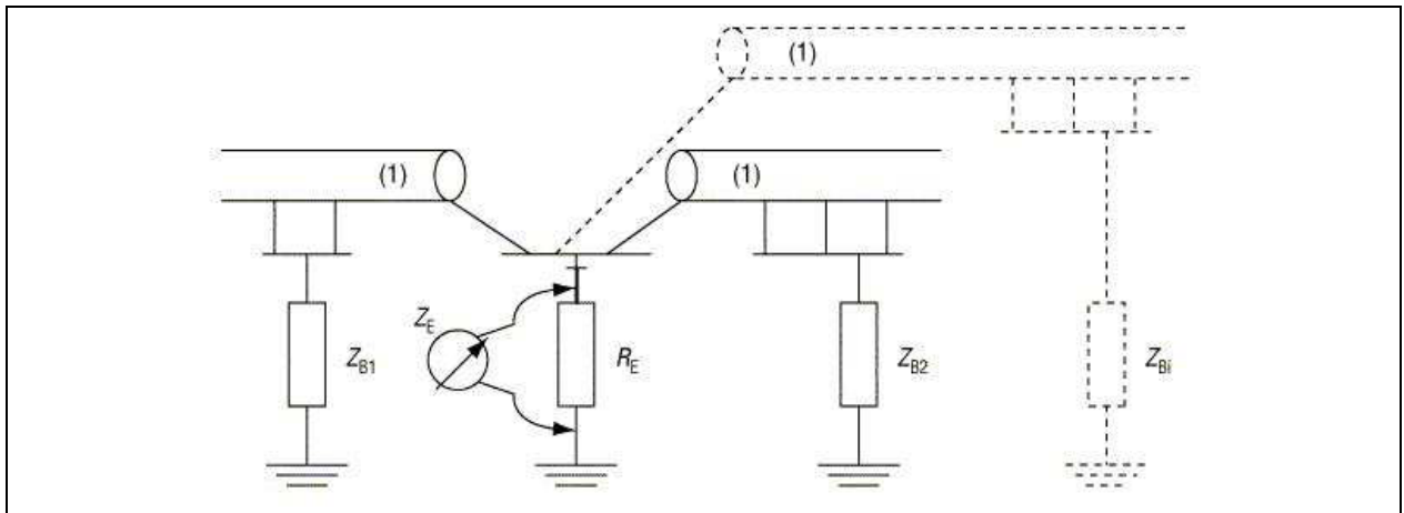
Figuur 2.14. Aardingsimpedantie Z_E
