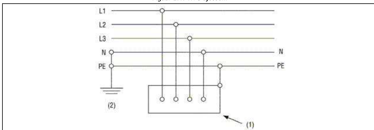
Figuur 2.1. TN-S-systeem
