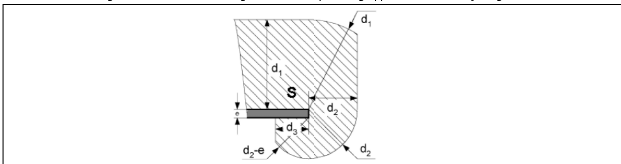
Figuur 2.6. Genaakbaarheidsgabarit: het verplaatsingsoppervlak is natuurlijk begrensd
