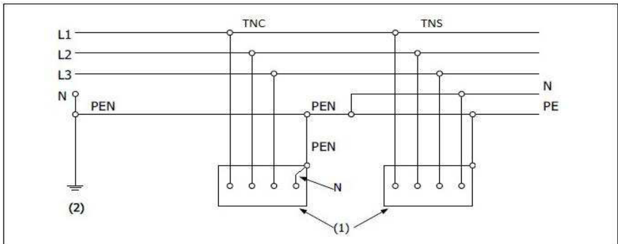
Figuur 2.3. TN-C-S-systeem
