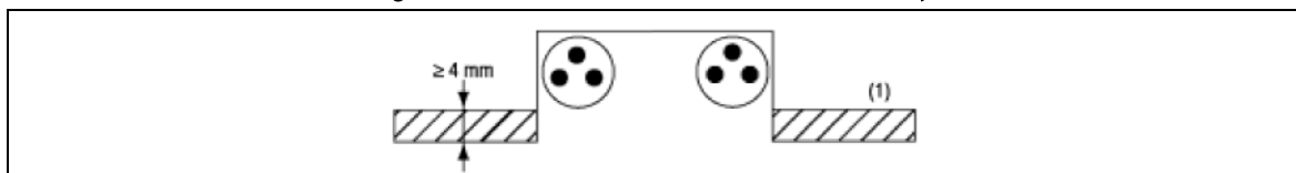
Figuur 5.42. Schematische doorsnede van een sleuf
