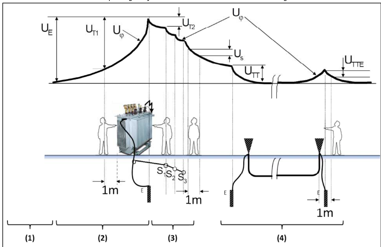
Figuur 2.12. Voorbeeld van verandering van aardbodemschijf en van spanningen bij het vloeien van stroom in de aardverbindingen
