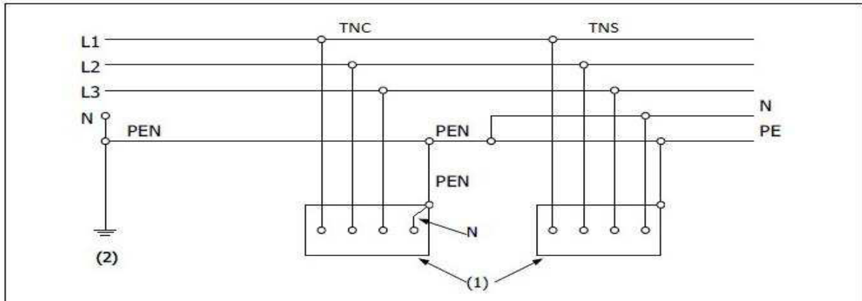
Figuur 3.1. TN-C-S-net
