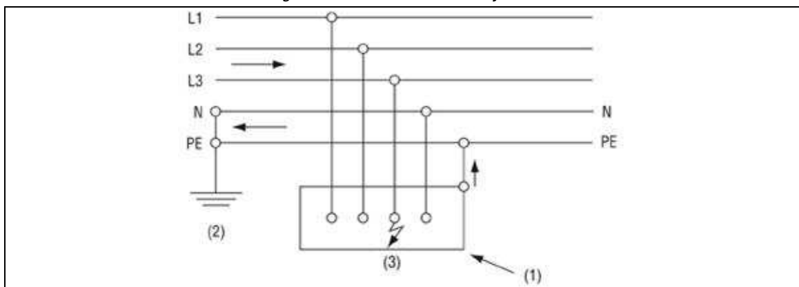
Figuur 4.3. Foutlus in een TN-S-systeem
