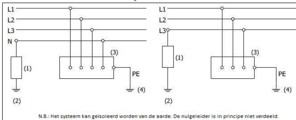
Figuur 3.3. IT-net
