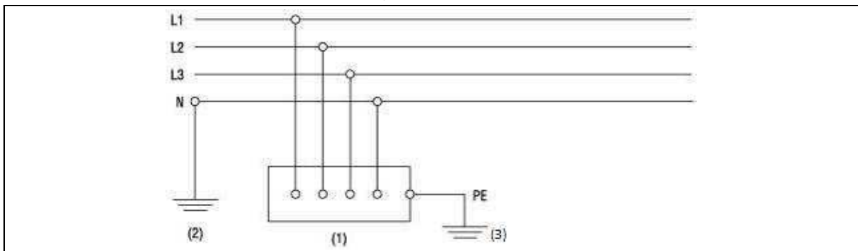
Figuur 3.2. TT-net
