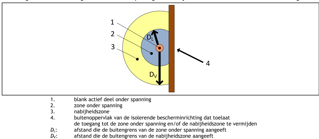
Figuur 2.29. Voorstelling van de zone onder spanning en de nabijheidszone met isolerende bescherming
