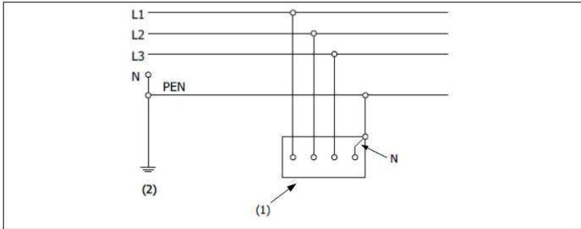
Figuur 2.2. TN-C-systeem
