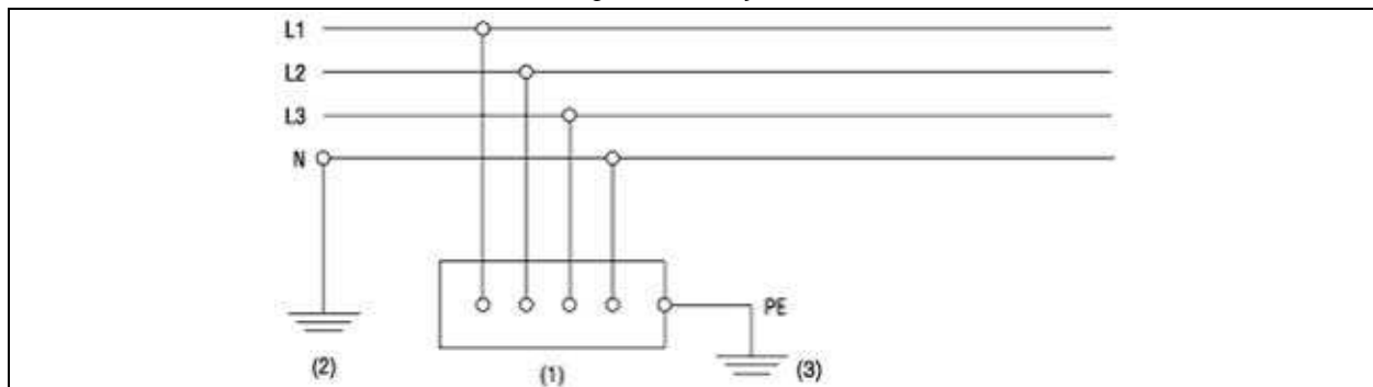
Figuur 2.4. TT-systeem
