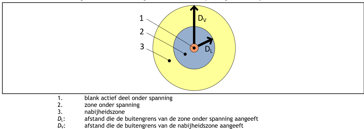
Figuur 2.29. Voorstelling van de zone onder spanning en de nabijheidszone met isolerende bescherming
