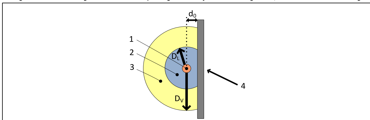
Figuur 2.30. Voorstelling van de zone onder spanning en de nabijheidszone met geaarde, metalen bescherming
