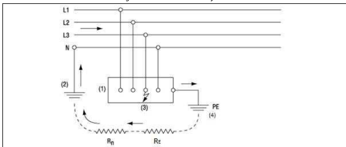
Figuur 4.6. Foutlus in een TT-systeem
