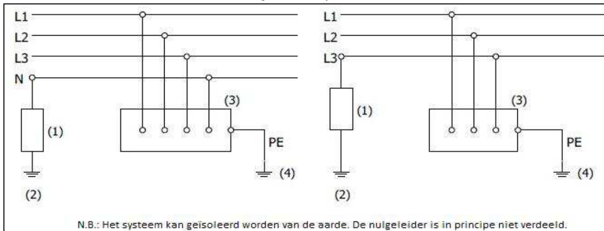
Figuur 2.5. IT-systeem
