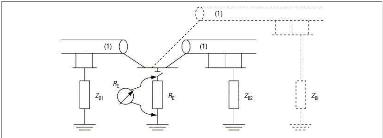
Figuur 2.13. Aardingsweerstand R_E
