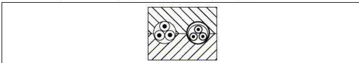
Figuur 5.20. Plaatsingswijzen van elektrische leidingen – Geprefabriceerde blokken
