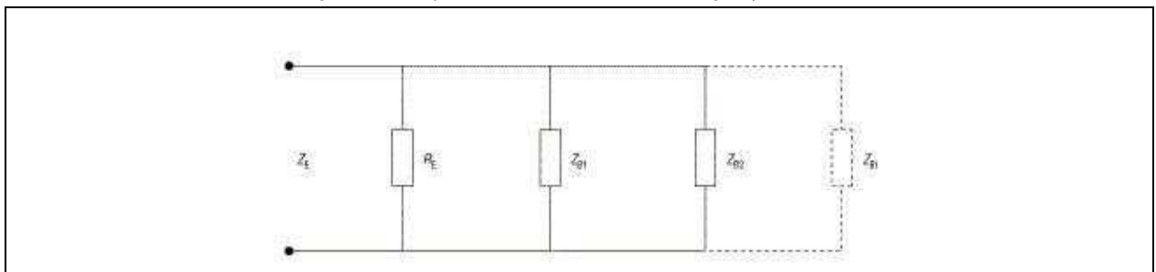
Figuur 2.15. Equivalent schema van de aardingsimpedantie Z_E
