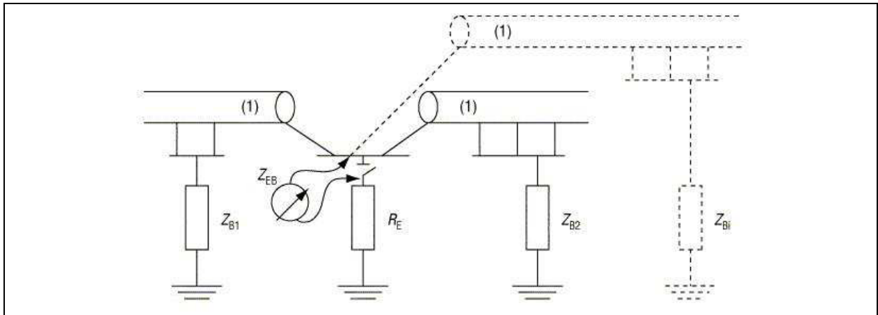
Figuur 2.16. Lusimpedantie van een aardverbinding Z_{EB}
