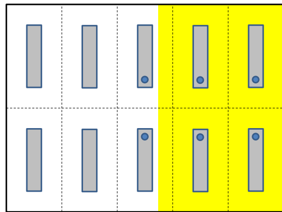
Figuur [2]: Configuratie waarbij niet alle armaturen worden bediend door eenzelfde dimsysteem - de daglichtoppervlakte ligt volledig binnen de gebruiksovervlakte die bediend wordt door het systeem
