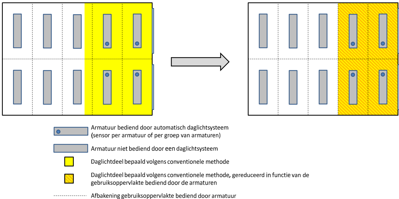
Figuur [3]: Configuratie waarbij niet alle armaturen worden bediend door eenzelfde dimsysteem - de daglichtoppervlakte ligt deels buiten de gebruiksovervlakte die bediend wordt door het systeem
