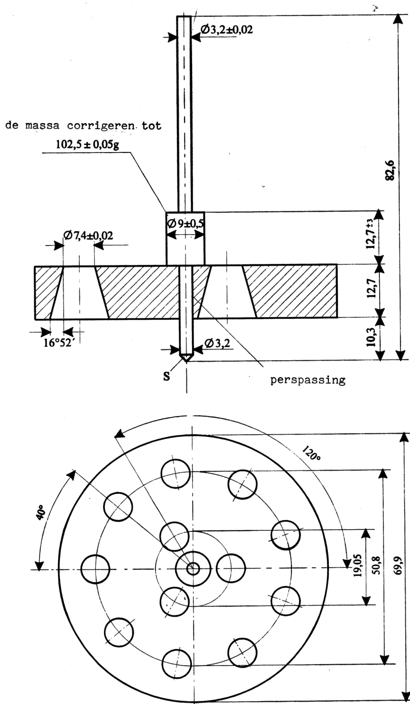
Figuur 1 Penetrometer
