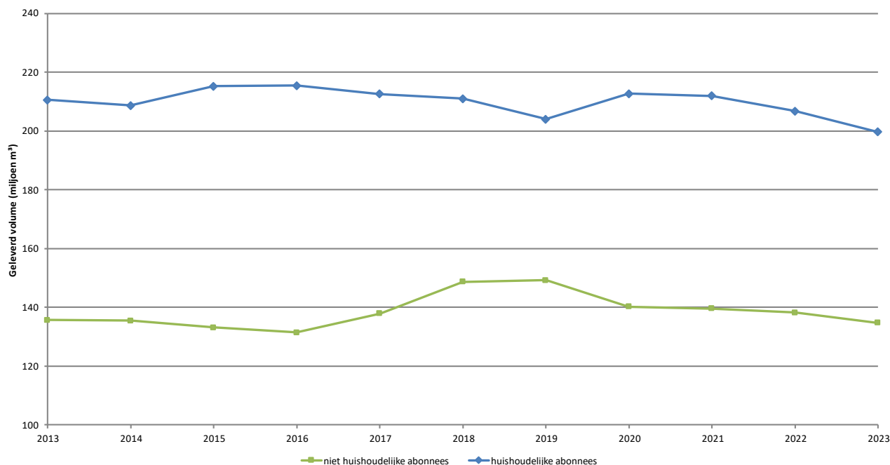
figuur 11: Evolutie van het geleverde drinkwater verdeeld over het huishoudelijk en niet-huishoudelijk verbruik in miljoen m³ voor de periode 2013- 2023.
