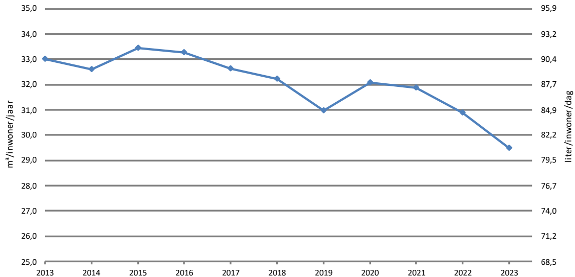
figuur 13: Evolutie het volume geleverd aan huishoudelijke abonnees in Vlaanderen uitgedrukt per inwoner tussen 2013 en 2023 in m 3 /inwoner/jaar (linkeras) en liter/inwoner/dag (rechteras)
