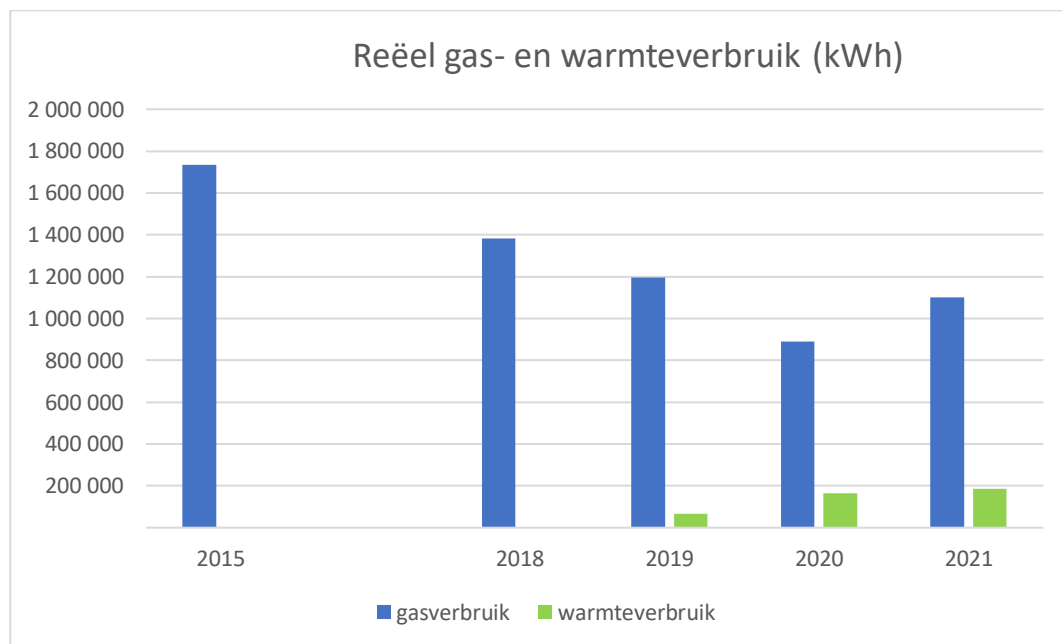
Figuur 4: Totale reële gasverbruik in kWh
