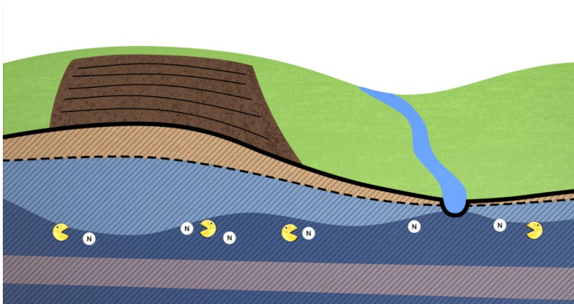
Figuur 91 Nitraatafbraak in de reductiezone met behulp van micro-organismen
