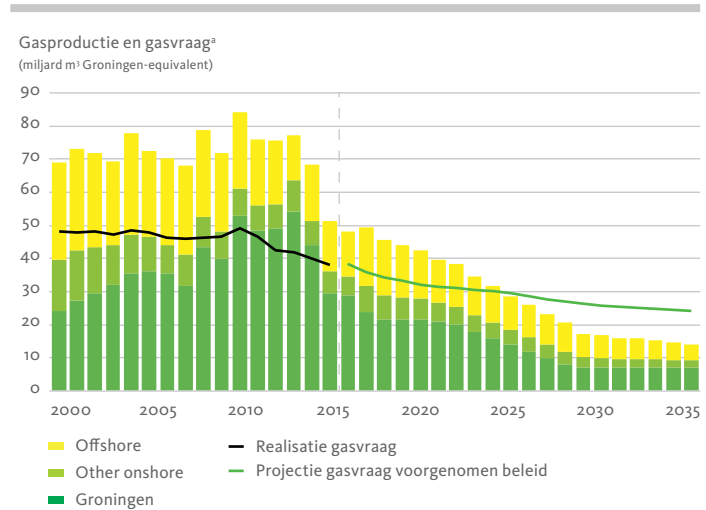
Figuur 4.9 Nederlandse gasproductie en gasvraag a . Bron: TNO 2016.
