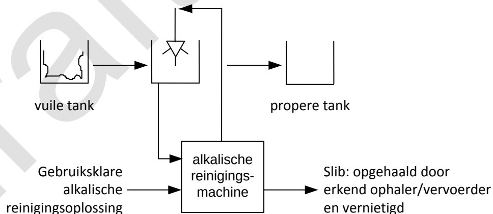
Figuur 17. Alkalische reiniging van draagbare mengtanks met recyclage van het bezinkingsresidu.
