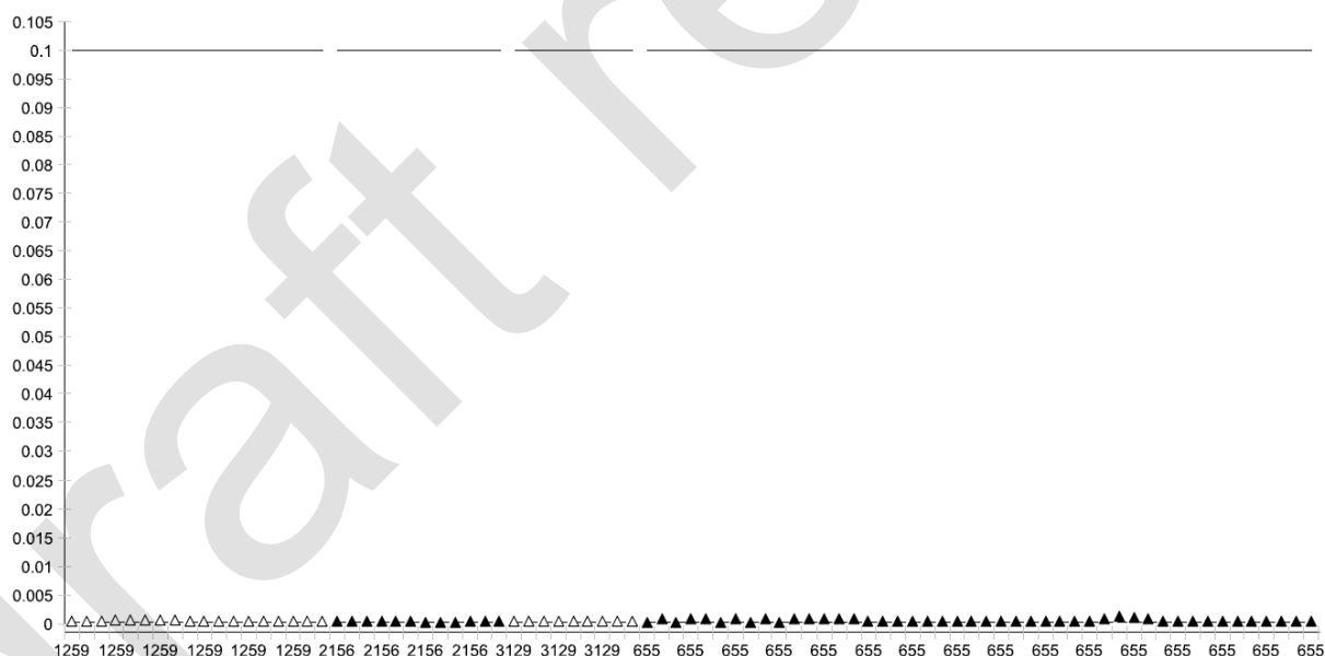
Figuur II.12. Hg (mg/l) lozingsgegevens op riool van coatings- en inktproducenten (VMM, 2012). De bedrijven (ID-nummer) worden met afwisselend zwart-wit symbolen aangeduid. sectorale norm = 0,1 mg/l; indelingscriterium GS = 0,0003 mg/l.
