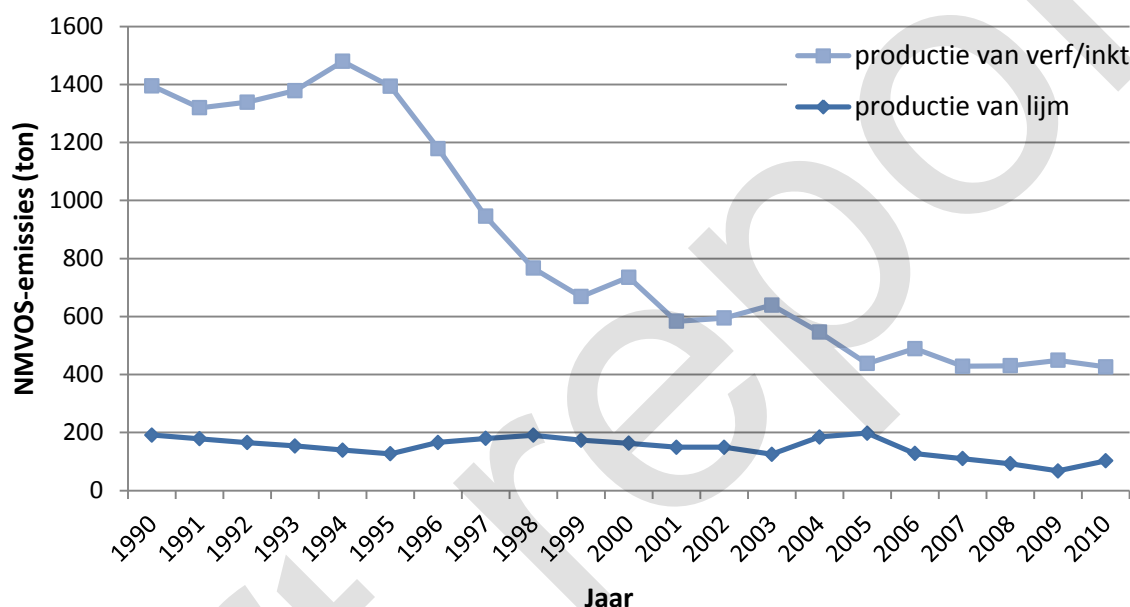
Figuur 24. Emissies voor niet-methaan vluchtige organische stoffen (NMVOS) bij de productie van verf, drukinkt en lijm in Vlaanderen volgens de VMM.
