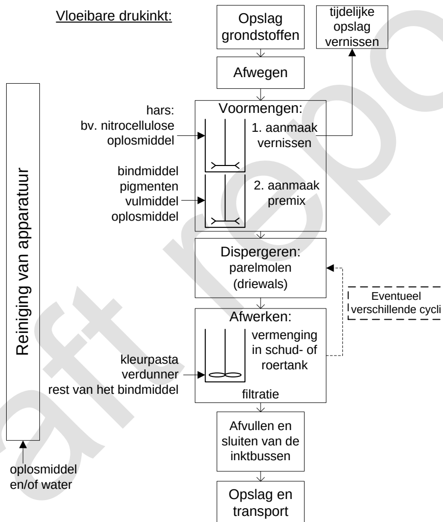
Figuur 20. Productie van drukinkten.
