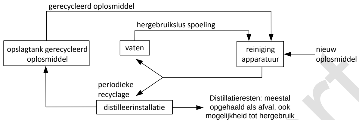
Figuur 18. Hergebruik van oplosmiddelen d.m.v. destillatie.
