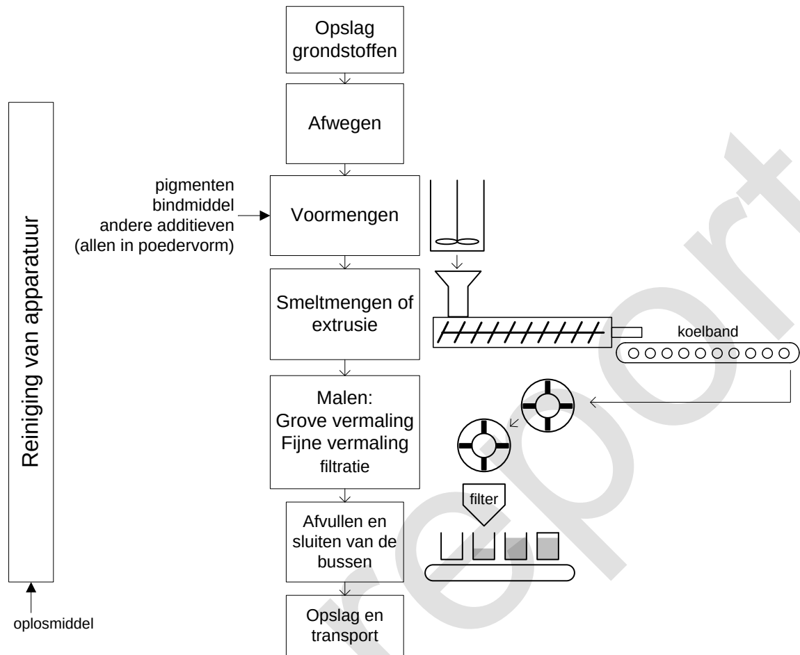
Figuur 19. Productie van poederverven.
