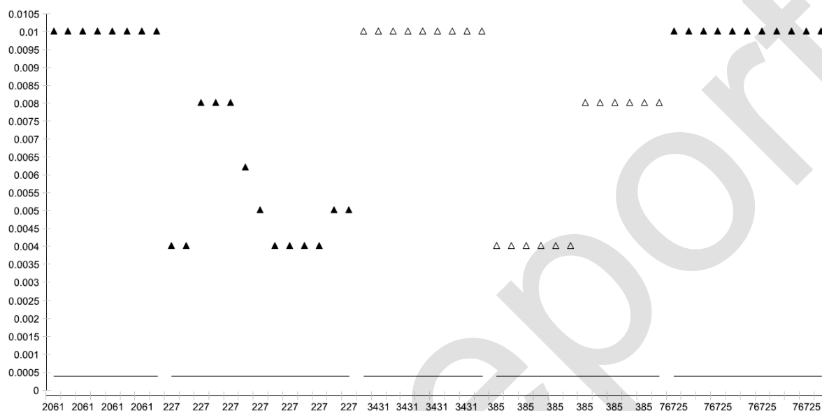
Figuur II.1. Ag (mg/l) lozingsgegevens op oppervlaktewater van coatings- en inktproducenten (VMM, 2012). De bedrijven (ID-nummer) worden met afwisselend zwart-wit symbolen aangeduid. indelingscriterium GS = 0,0004 mg/l; Rapportagegrens = .0,01 mg/l.
