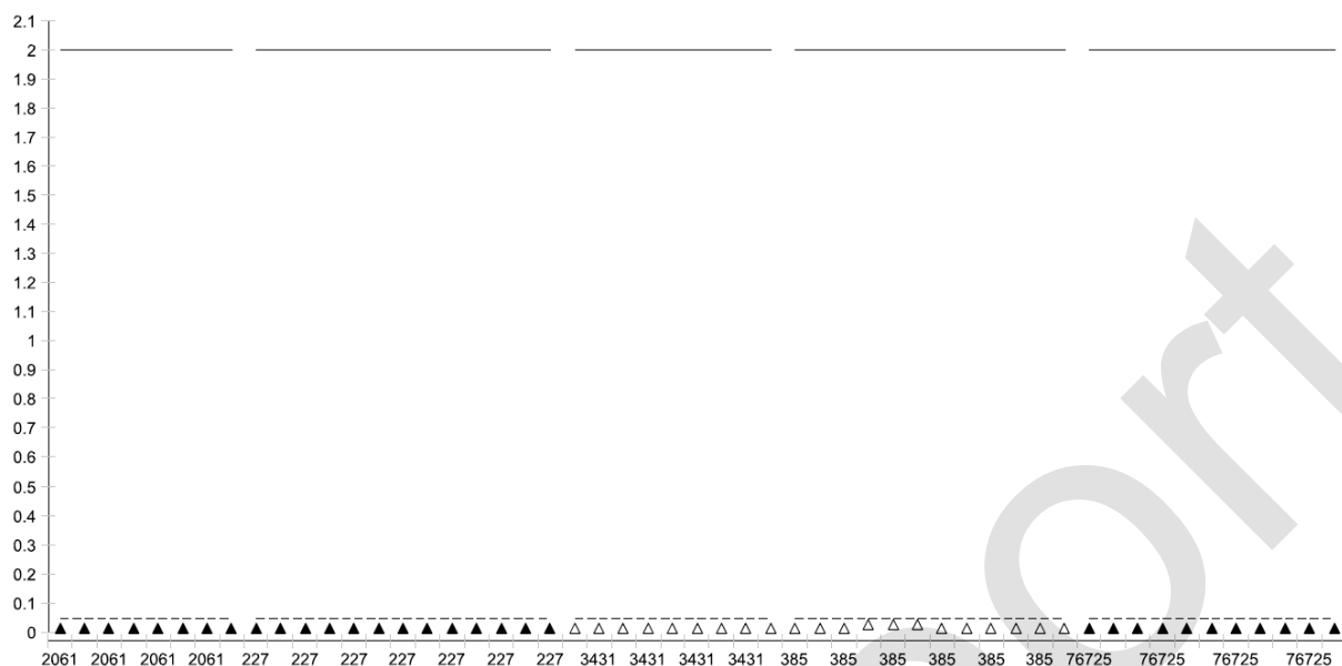
Figuur II.7. Cr (mg/l) lozingsgegevens op oppervlaktewater van coatings- en inktproducenten (VMM, 2012). De bedrijven (ID-nummer) worden met afwisselend zwart-wit symbolen aangeduid. sectorale norm = 2,0 mg/l; indelingscriterium GS = 0,05 mg/l.
