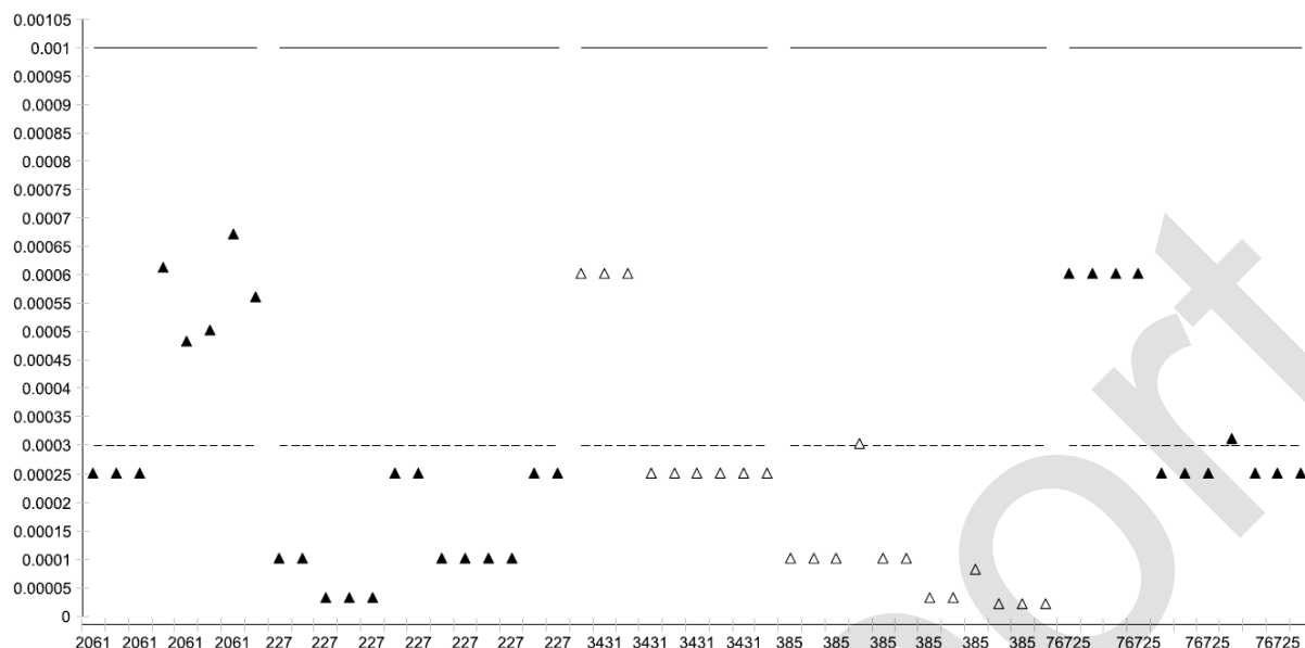
Figuur II.11. Hg (mg/l) lozingsgegevens op oppervlaktewater van coatings- en inktproducenten (VMM, 2012). De bedrijven (ID-nummer) worden met afwisselend zwart-wit symbolen aangeduid. sectorale norm = 0,001 mg/l; indelingscriterium GS = 0,0003 mg/l.
