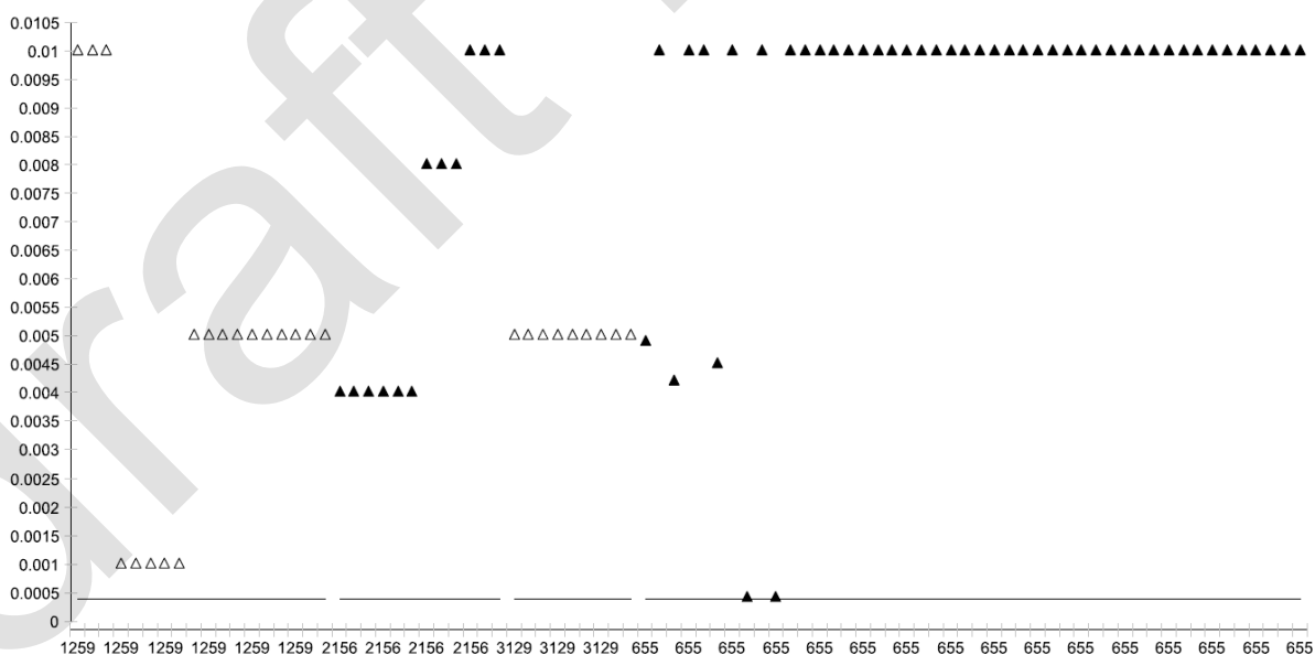
Figuur II.2. Ag (mg/l) lozingsgegevens op riool van coatings- en inktproducenten (VMM, 2012). De bedrijven (ID-nummer) worden met afwisselend zwart-wit symbolen aangeduid. indelingscriterium GS = 0,0004 mg/l; Rapportagegrens = .0,01 mg/l.
