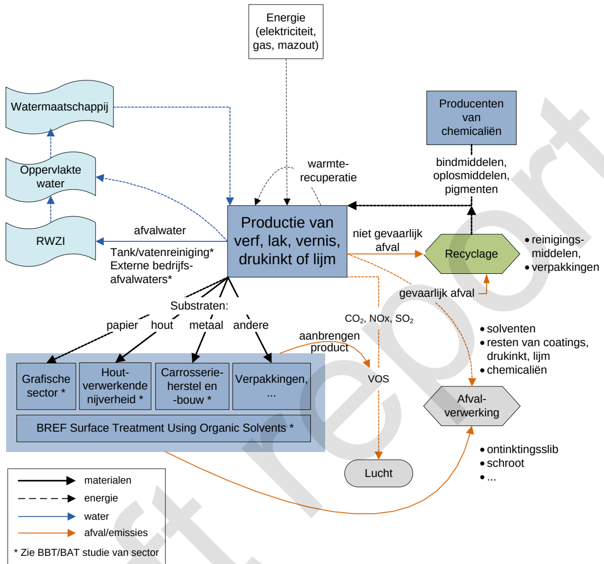
Figuur 26. Energie- en materiaalstromen in de productketen
