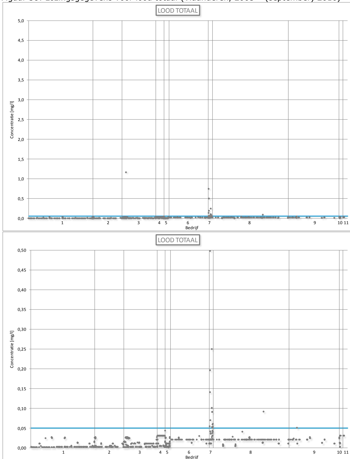
Figuur 38: Lozingsgegevens voor lood totaal (Vlaanderen, 2005 – (september) 2010)
