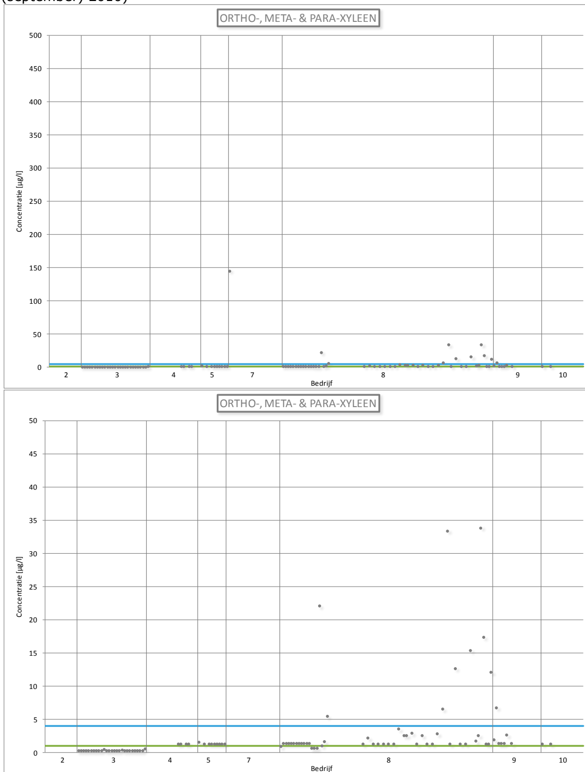
Figuur 70: Lozingsgegevens voor ortho-, meta- & para-xyleen (Vlaanderen, 2005 – (september) 2010)
