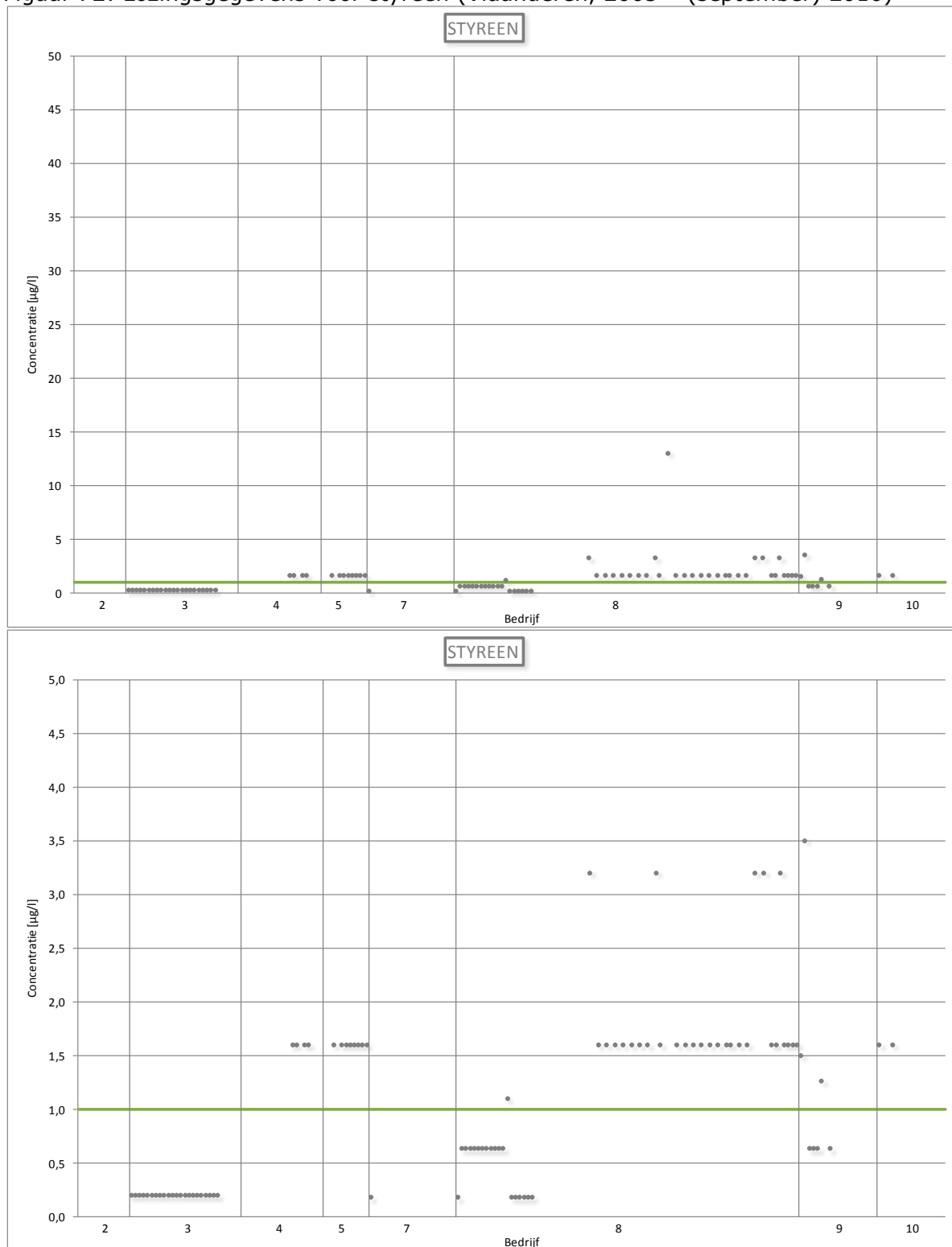
Figuur 72: Lozingsgegevens voor styreen (Vlaanderen, 2005 – (september) 2010)
