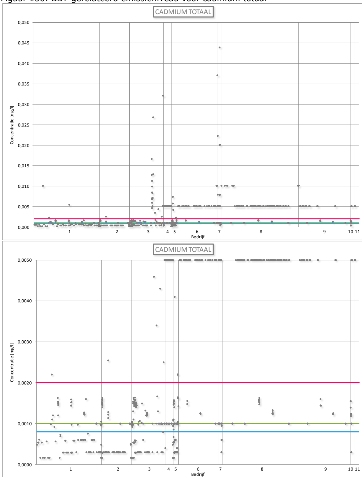
Figuur 136: BBT-gerelateerd emissieniveau voor cadmium totaal
