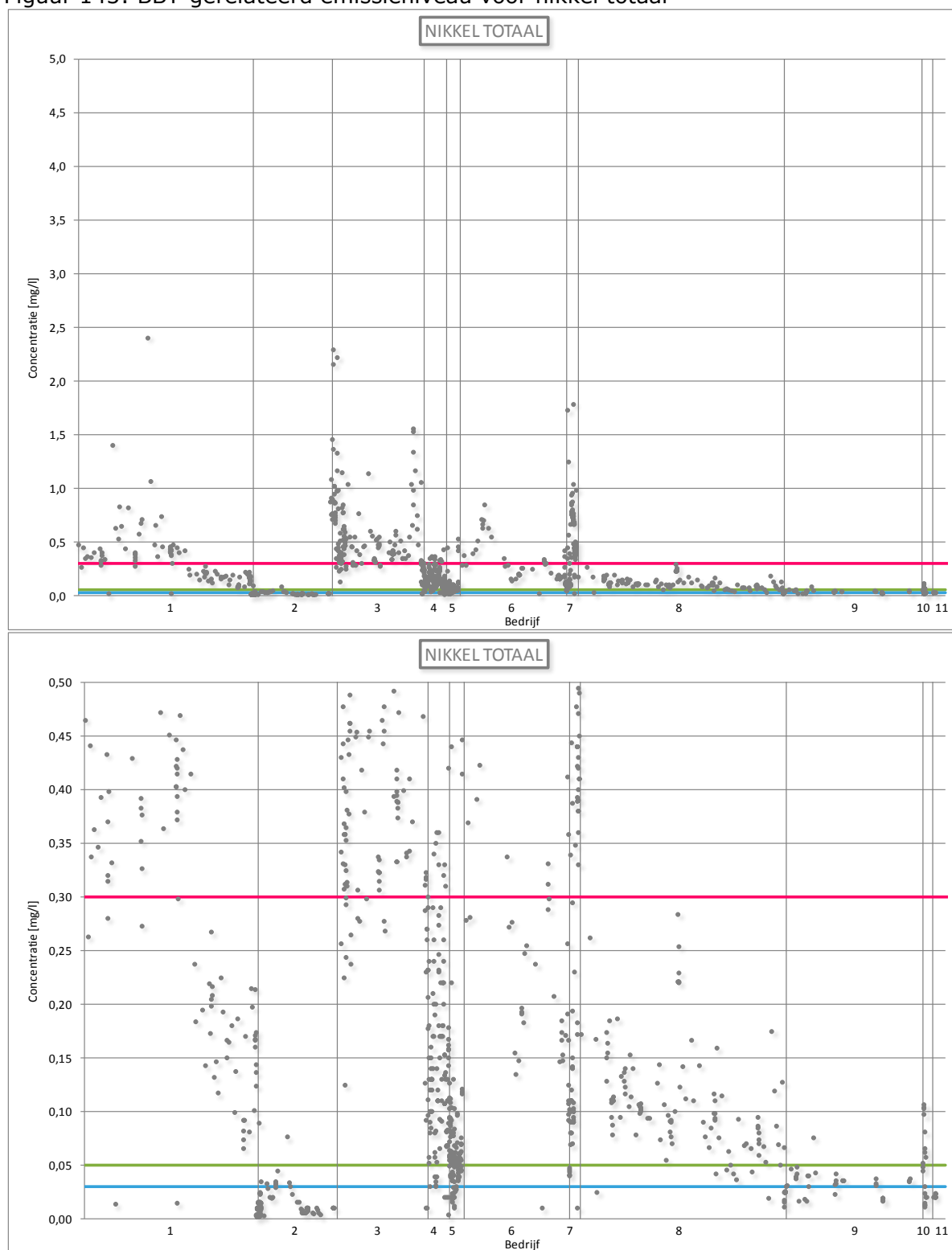
Figuur 143: BBT-gerelateerd emissieniveau voor nikkel totaal
