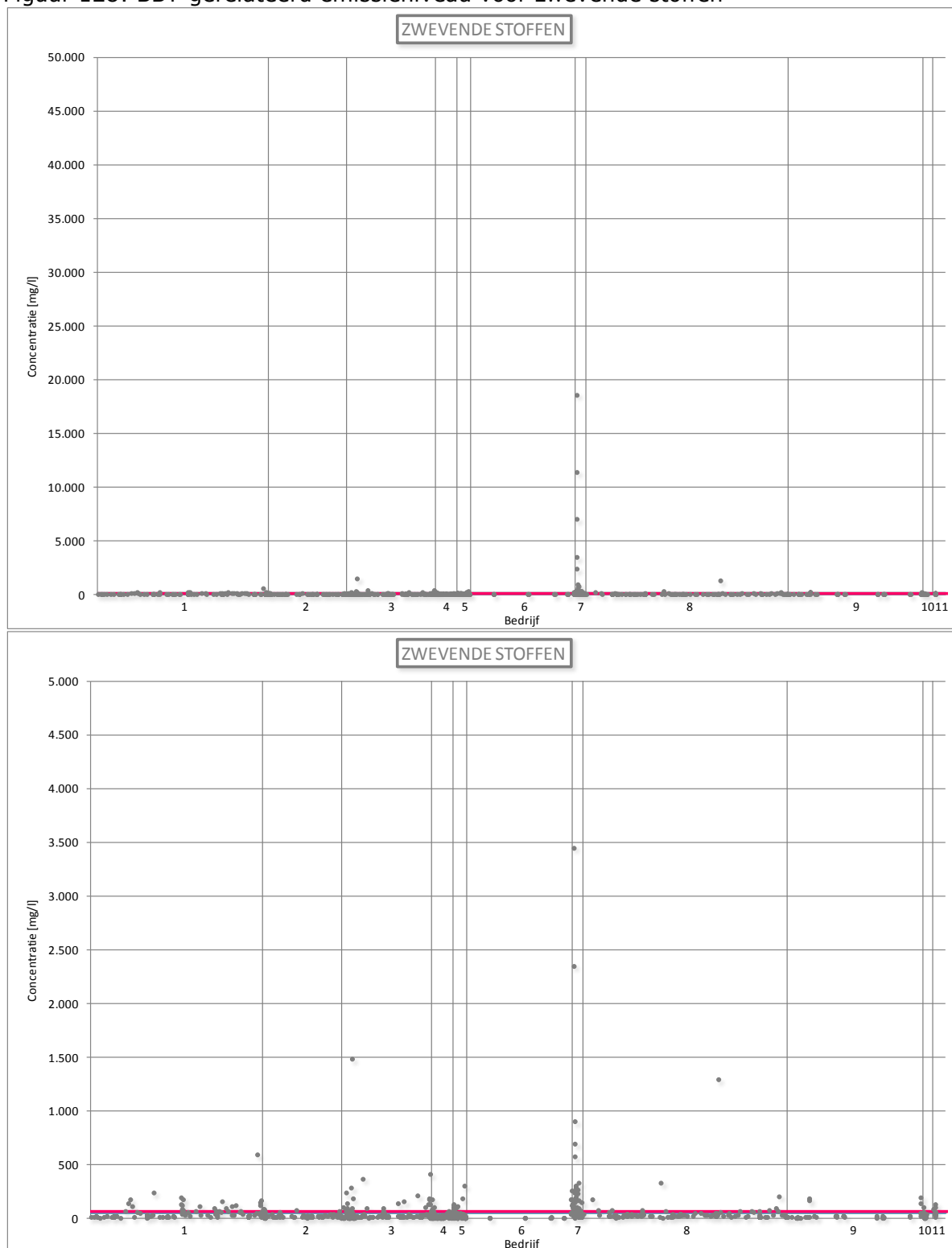
Figuur 128: BBT-gerelateerd emissieniveau voor zwevende stoffen
