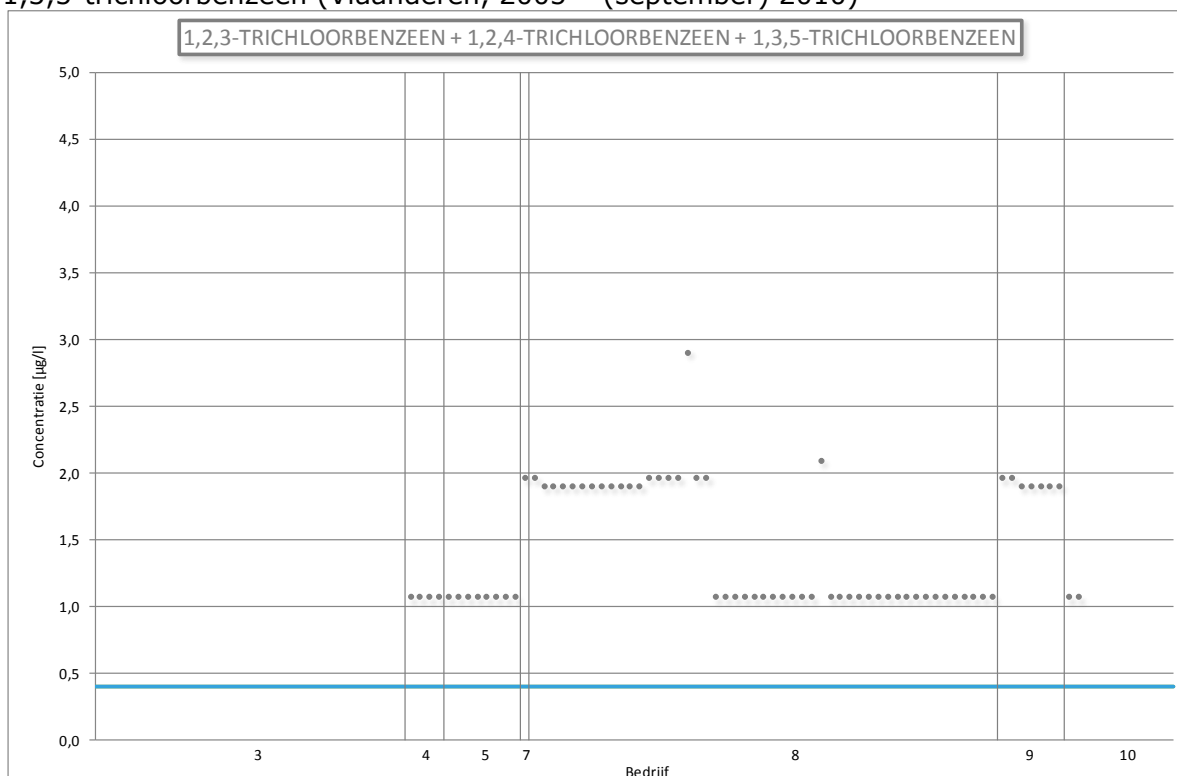
Figuur 111: Lozingsgegevens voor 1,2,3-trichloorbenzeen + 1,2,4-trichloorbenzeen + 1,3,5-trichloorbenzeen (Vlaanderen, 2005 – (september) 2010)
