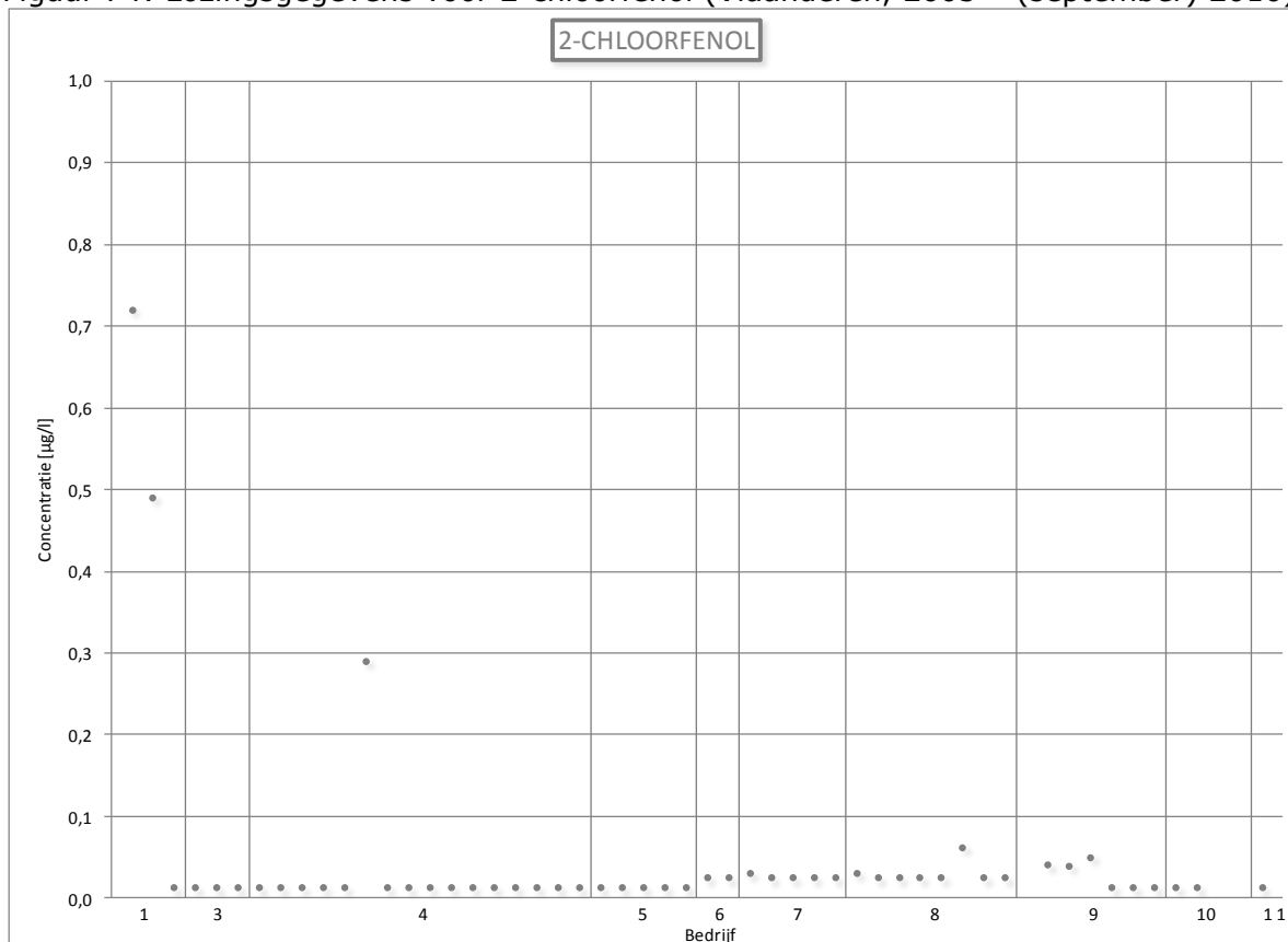
Figuur 74: Lozingsgegevens voor 2-chloorfenol (Vlaanderen, 2005 – (september) 2010)
