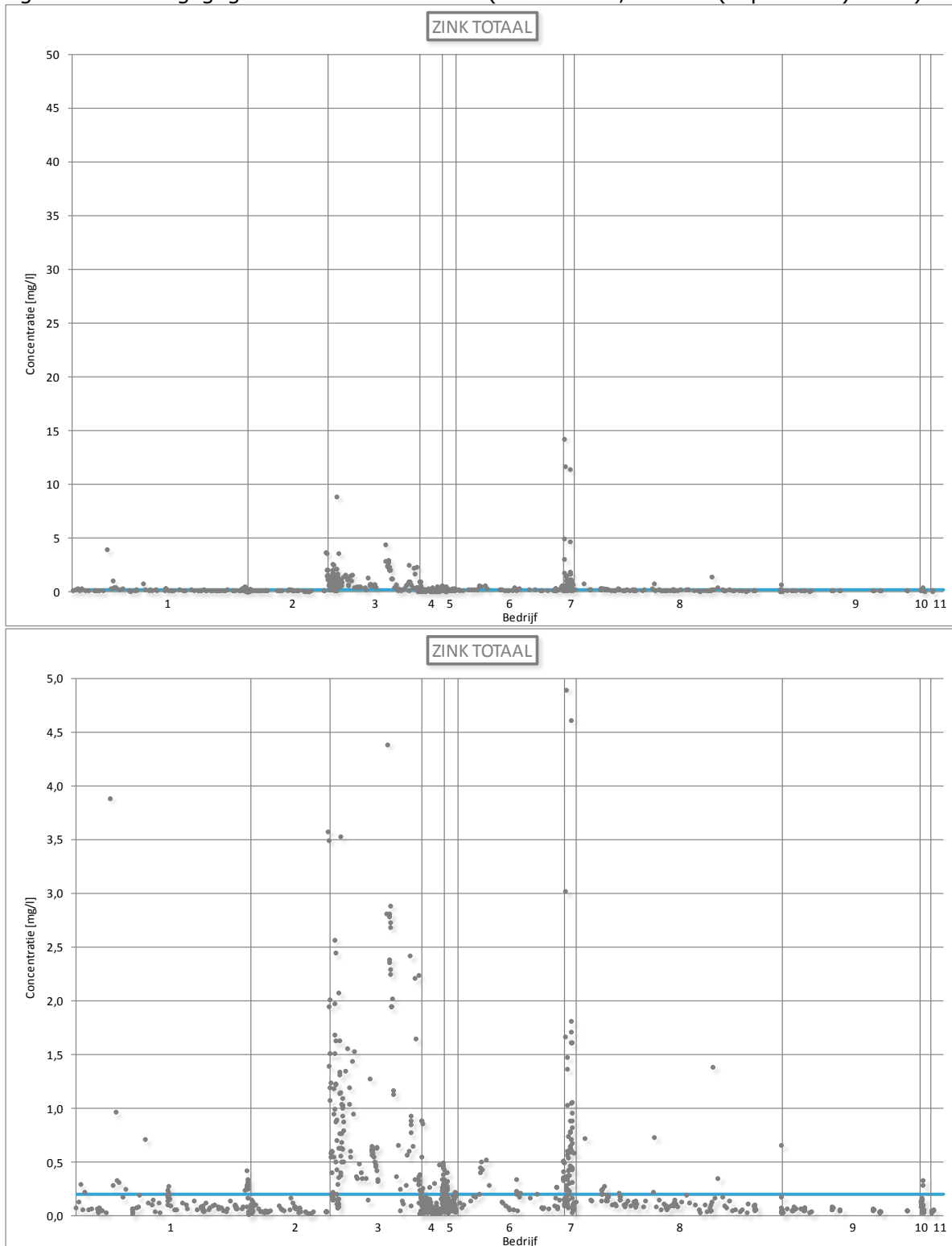
Figuur 44: Lozingsgegevens voor zink totaal (Vlaanderen, 2005 – (september) 2010)
