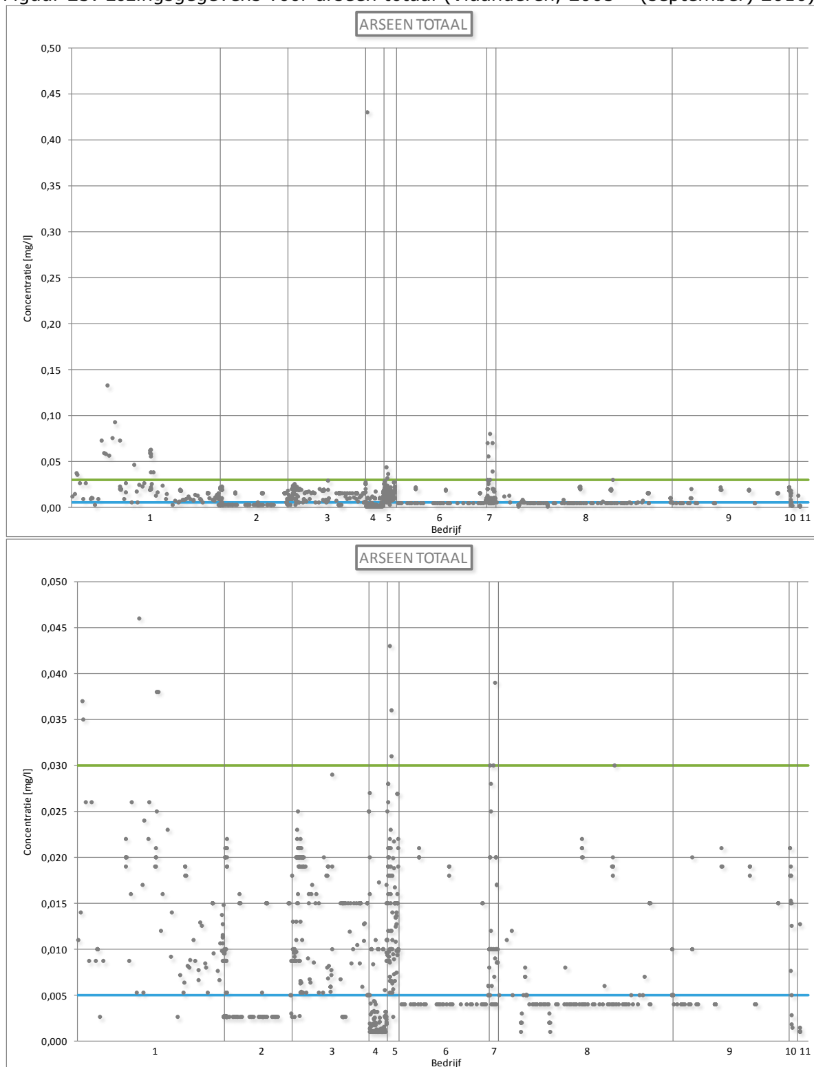
Figuur 25: Lozingsgegevens voor arseen totaal (Vlaanderen, 2005 – (september) 2010)
