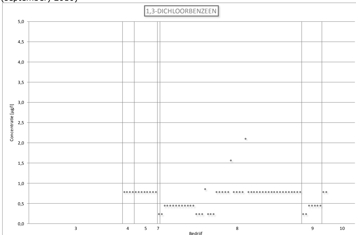
Figuur 105: Lozingsgegevens voor 1,3-dichloorbenzeen (Vlaanderen, 2005 – (september) 2010)
