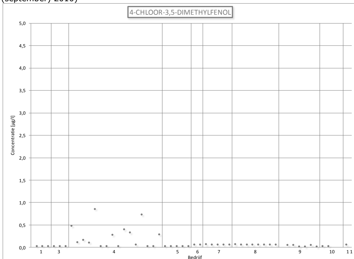
Figuur 81: Lozingsgegevens voor 4-chloor-3,5-dimethylfenol (Vlaanderen, 2005 – (september) 2010)
