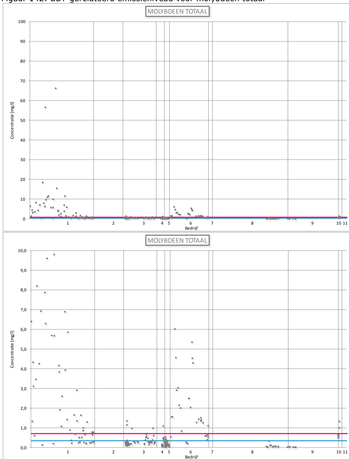
Figuur 142: BBT-gerelateerd emissieniveau voor molybdeen totaal
