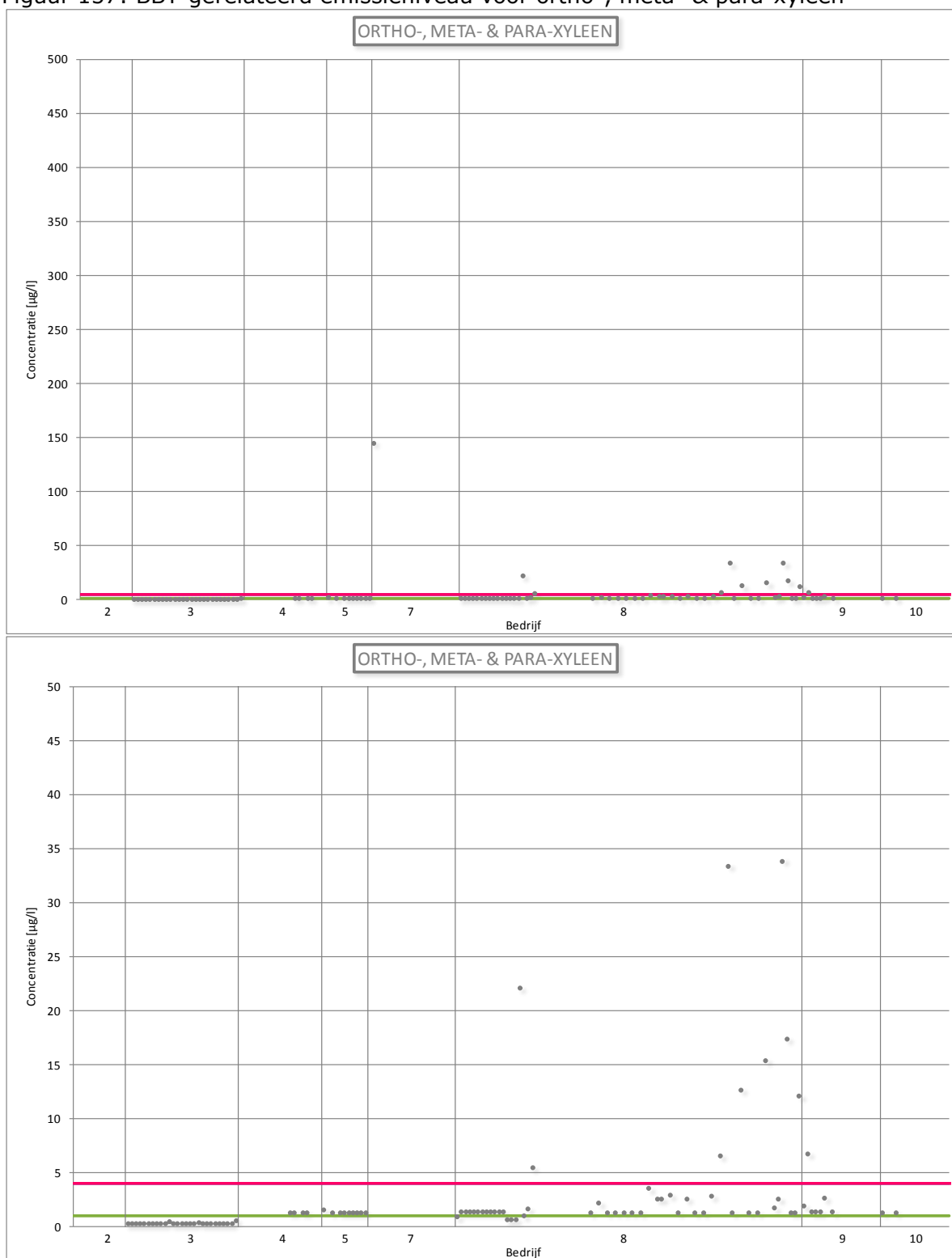
Figuur 157: BBT-gerelateerd emissieniveau voor ortho-, meta- & para-xyleen
