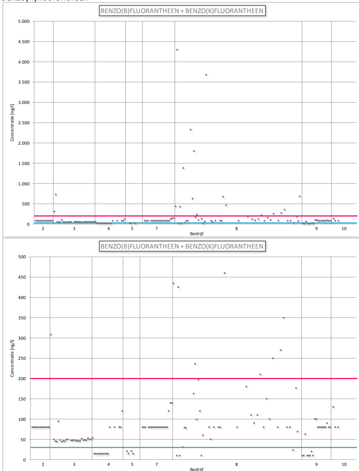
Figuur 152: BBT-gerelateerd emissieniveau voor benzo(b)fluorantheen & benzo(k)fluorantheen
