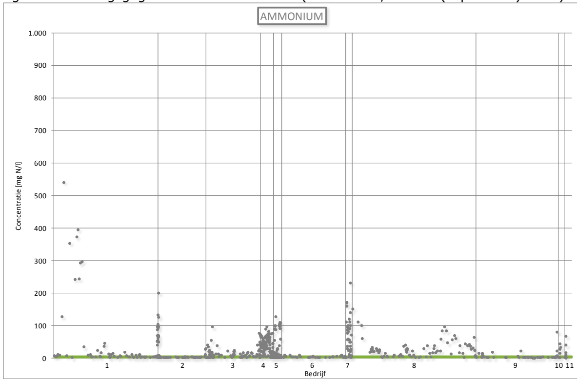
Figuur 14: Lozingsgegevens voor ammonium (Vlaanderen, 2005 – (september) 2010)
