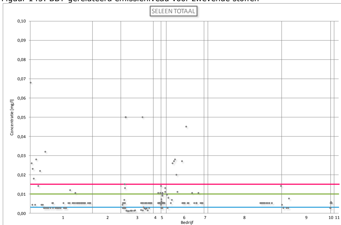
Figuur 145: BBT-gerelateerd emissieniveau voor zwevende stoffen
