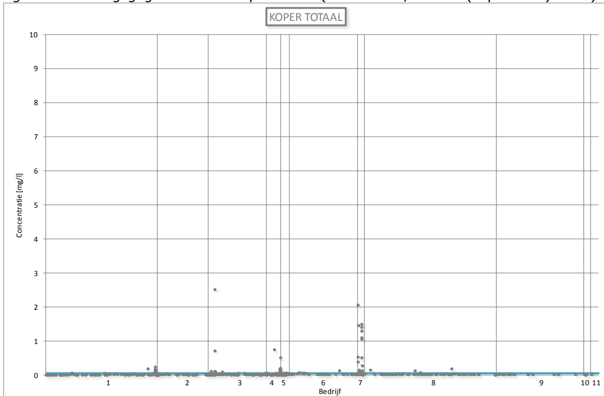
Figuur 32: Lozingsgegevens voor koper totaal (Vlaanderen, 2005 – (september) 2010)
