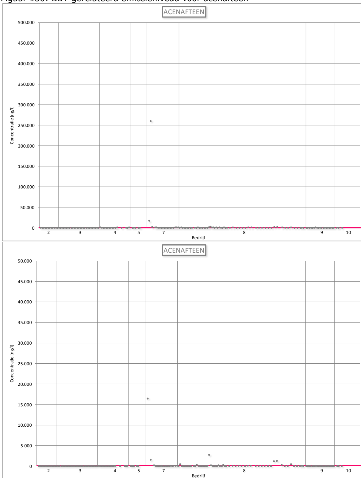
Figuur 150: BBT-gerelateerd emissieniveau voor acenafteen
