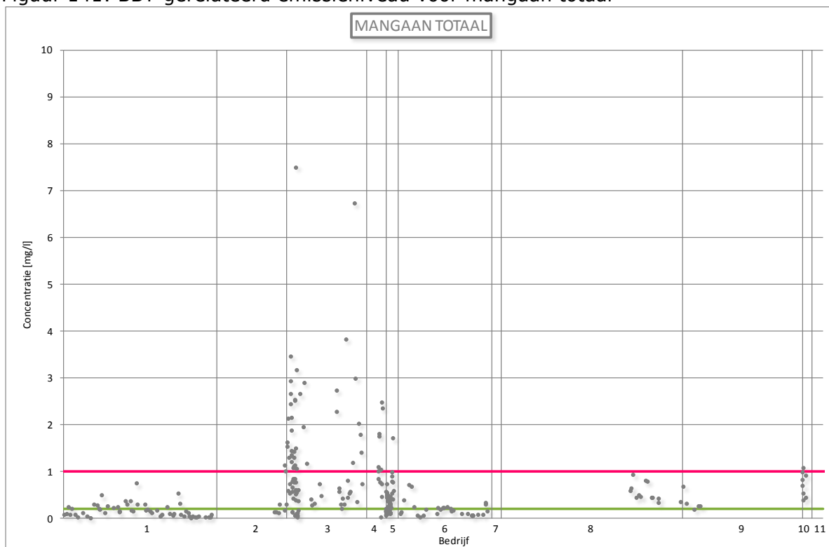
Figuur 141: BBT-gerelateerd emissieniveau voor mangaan totaal
