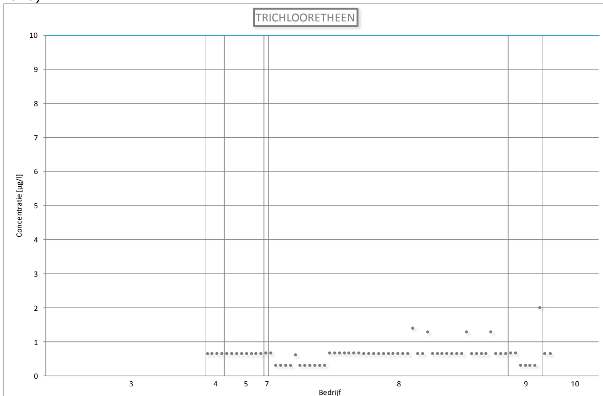
Figuur 101: Lozingsgegevens voor trichlooretheen (Vlaanderen, 2005 – (september) 2010)
