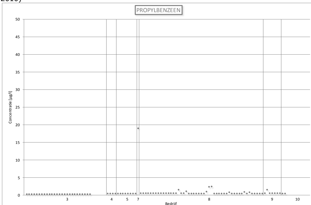
Figuur 89: Lozingsgegevens voor propylbenzeen (Vlaanderen, 2005 – (september) 2010)
