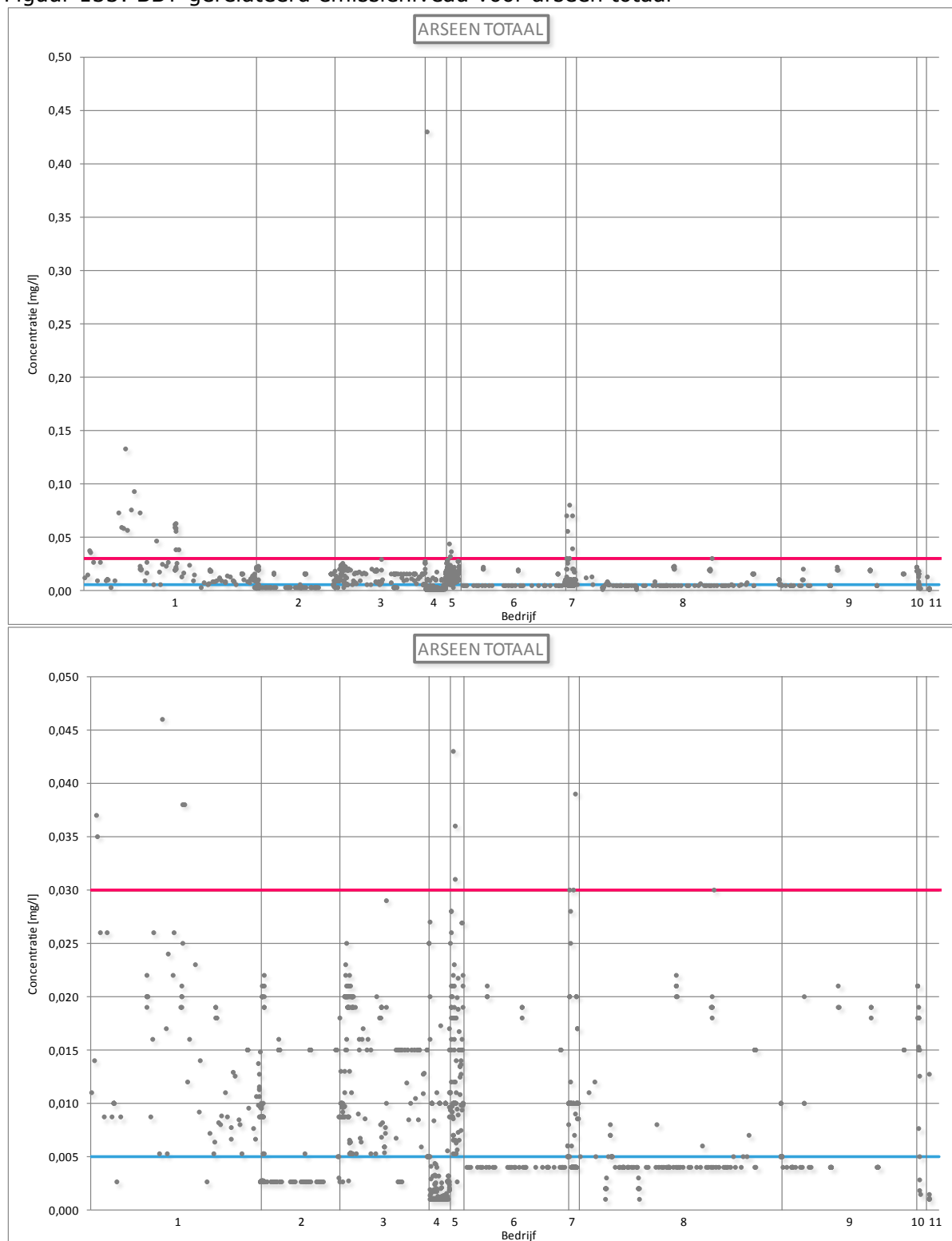
Figuur 133: BBT-gerelateerd emissieniveau voor arseen totaal
