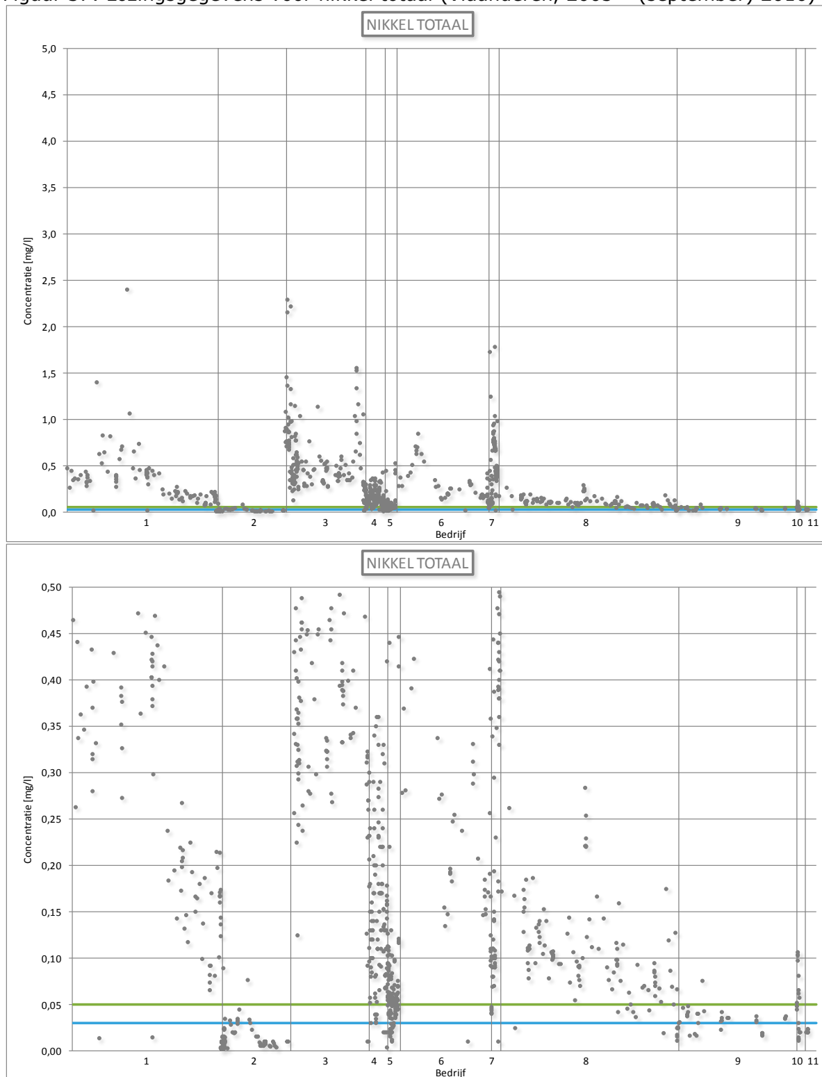
Figuur 37: Lozingsgegevens voor nikkel totaal (Vlaanderen, 2005 – (september) 2010)
