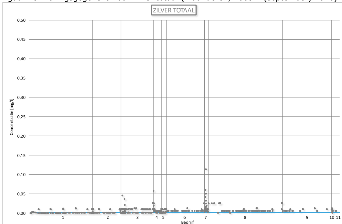
Figuur 23: Lozingsgegevens voor zilver totaal (Vlaanderen, 2005 – (september) 2010)
