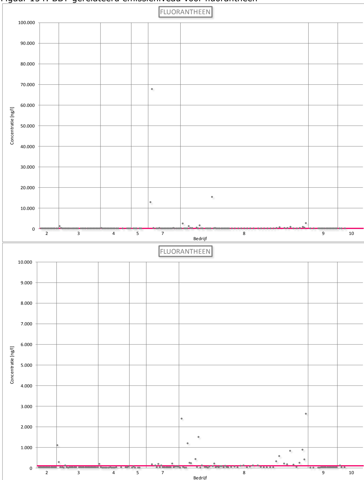
Figuur 154: BBT-gerelateerd emissieniveau voor fluorantheen
