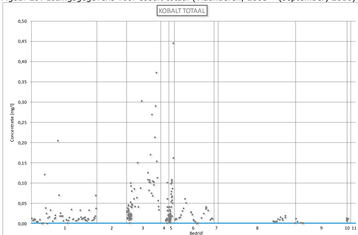
Figuur 29: Lozingsgegevens voor kobalt totaal (Vlaanderen, 2005 – (september) 2010)
