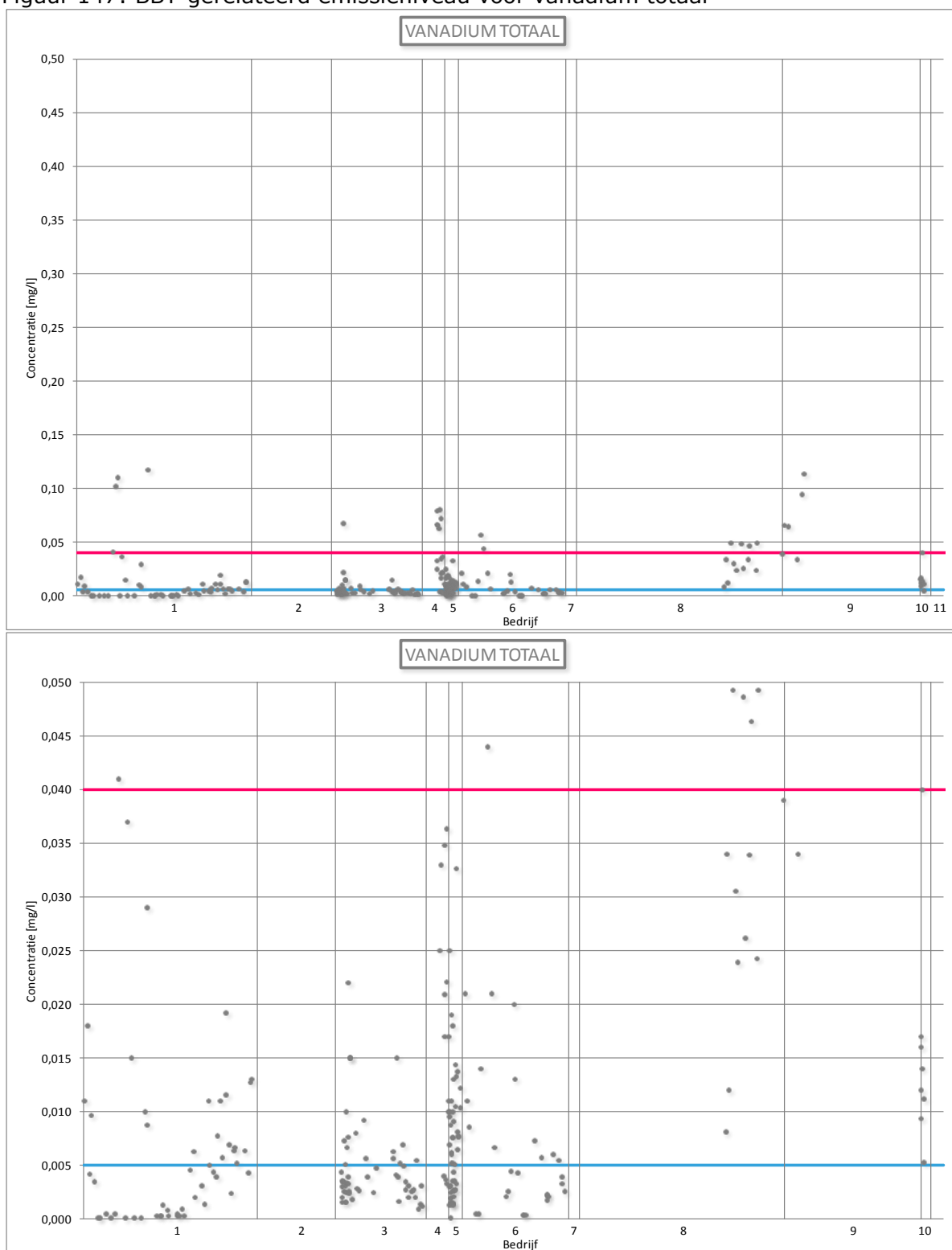
Figuur 147: BBT-gerelateerd emissieniveau voor vanadium totaal
