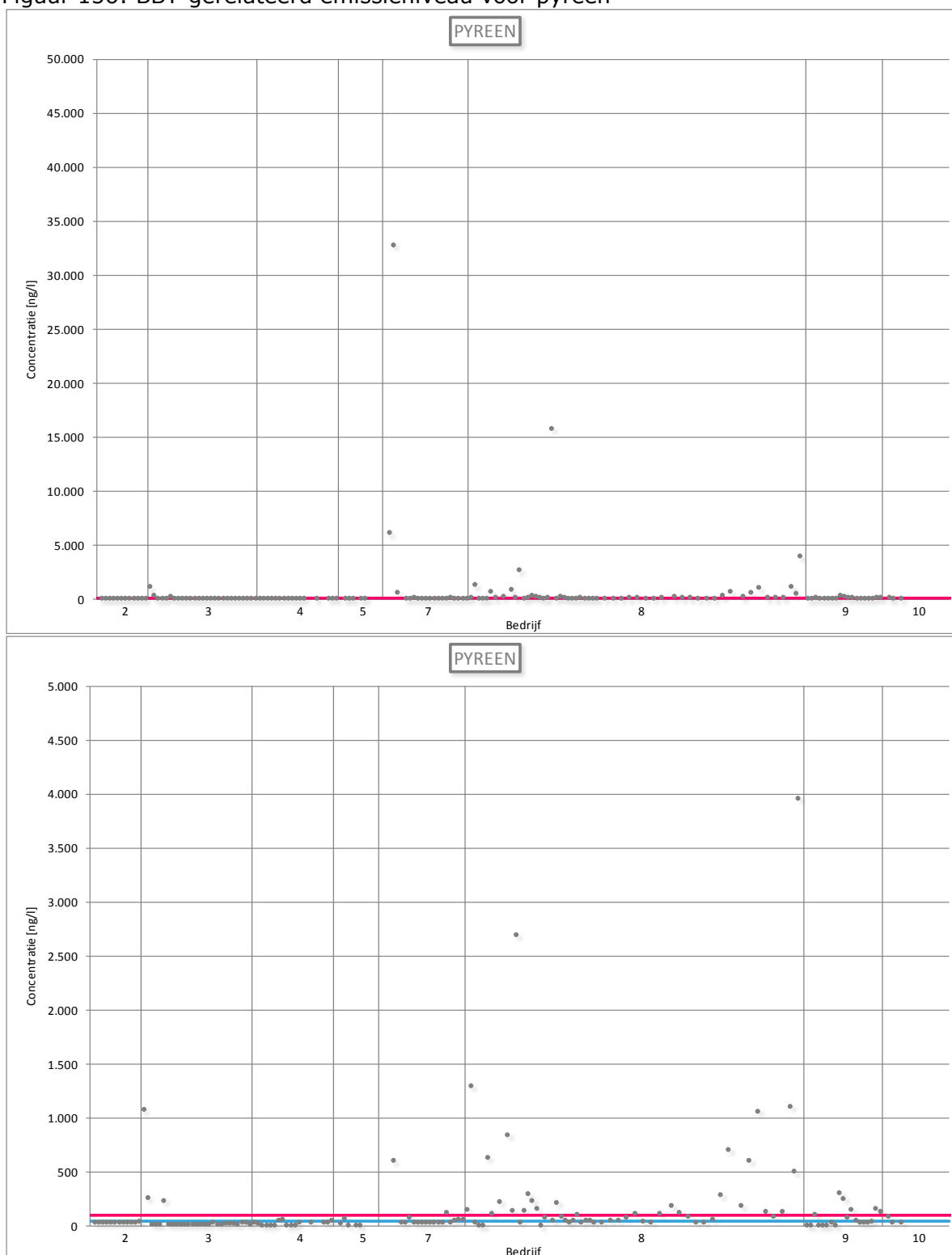
Figuur 156: BBT-gerelateerd emissieniveau voor pyreen
