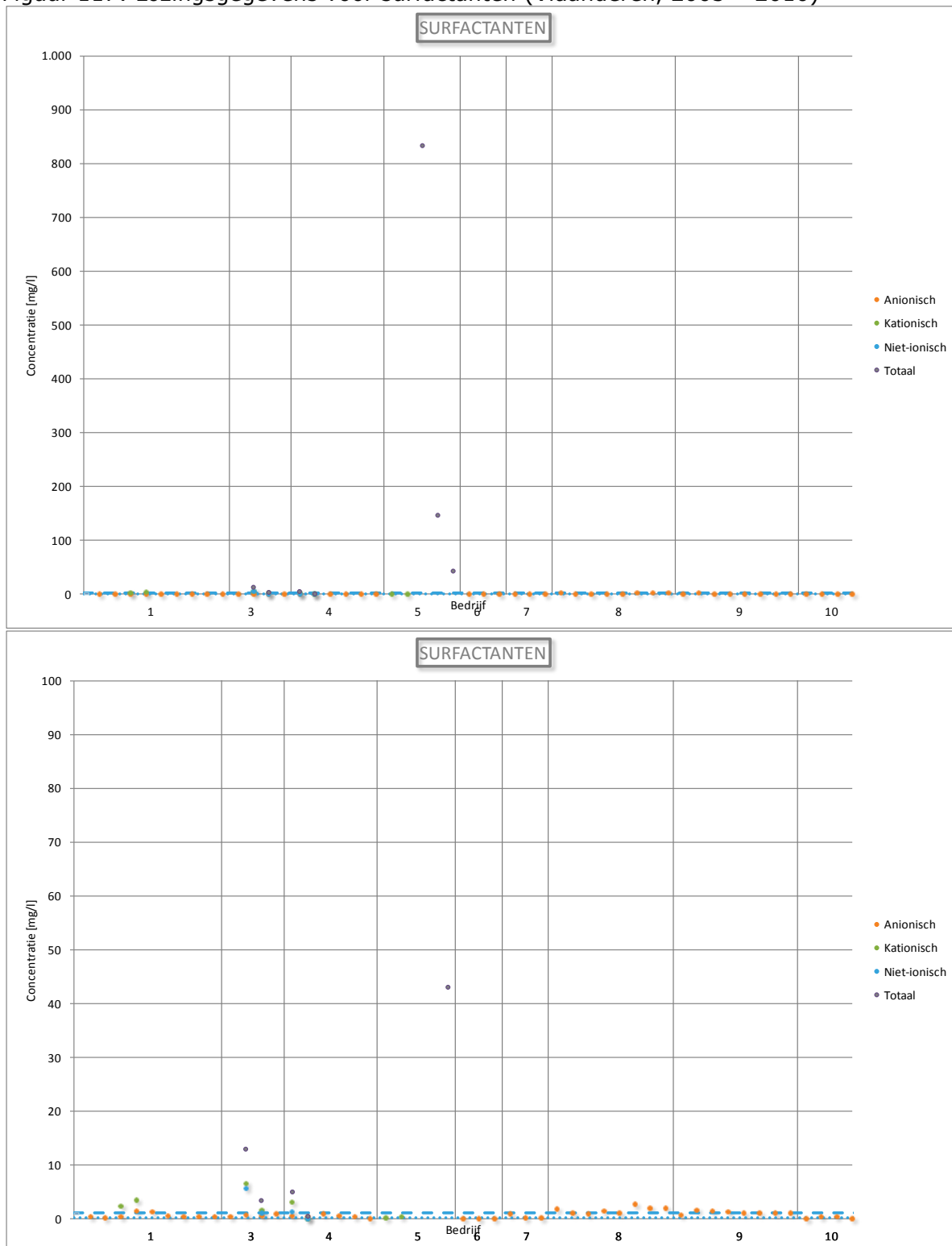
Figuur 117: Lozingsgegevens voor surfactanten (Vlaanderen, 2005 – 2010)
