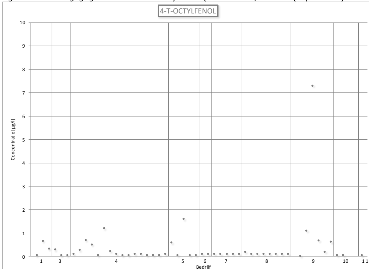
Figuur 85: Lozingsgegevens voor 4-t-octylfenol (Vlaanderen, 2005 – (september) 2010)
