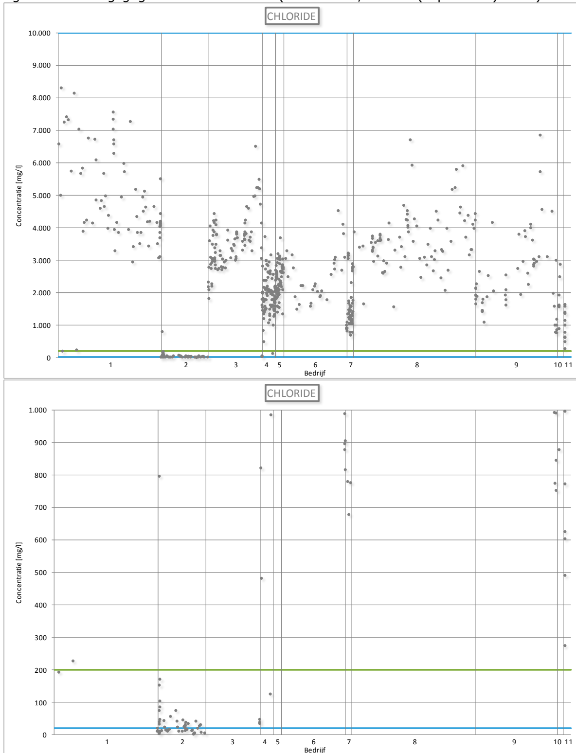
Figuur 12: Lozingsgegevens voor chloride (Vlaanderen, 2005 – (september) 2010)
