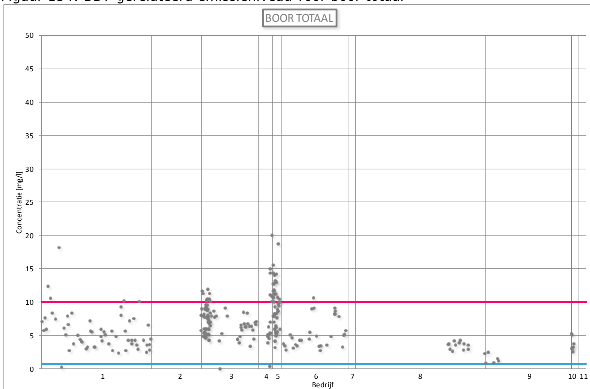
Figuur 134: BBT-gerelateerd emissieniveau voor boor totaal
