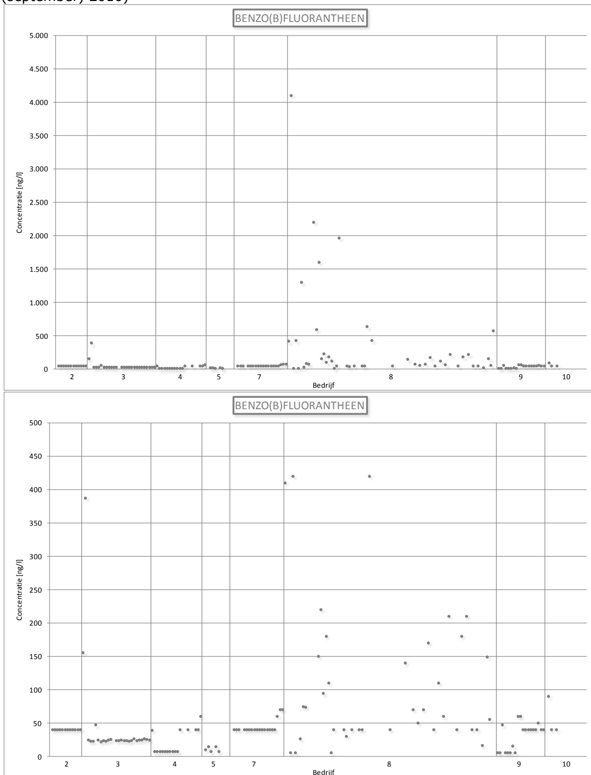
Figuur 51: Lozingsgegevens voor benzo(b)fluorantheen (Vlaanderen, 2005 – (september) 2010)
