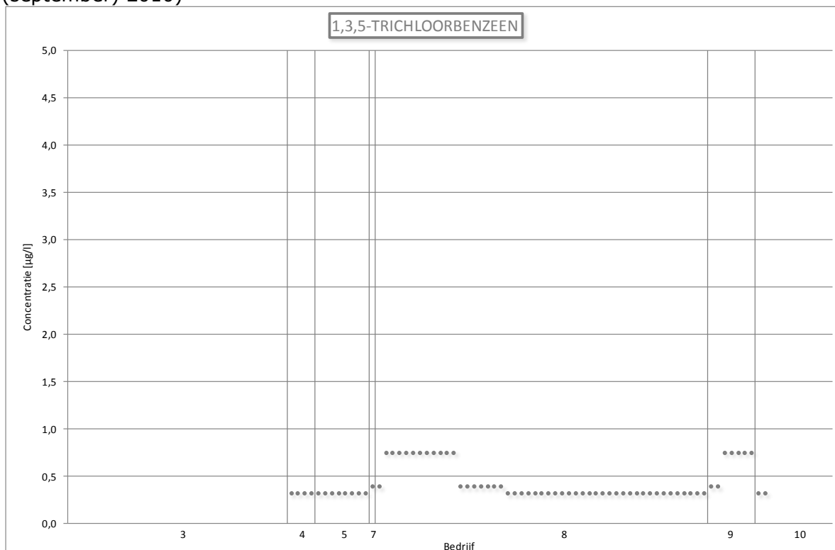
Figuur 110: Lozingsgegevens voor 1,3,5-trichloorbenzeen (Vlaanderen, 2005 – (september) 2010)
