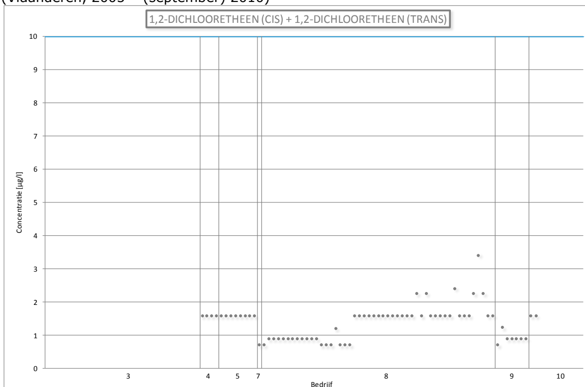
Figuur 95: Lozingsgegevens voor 1,2-dichlooretheen (cis) & 1,2-dichlooretheen (trans) (Vlaanderen, 2005 – (september) 2010)
