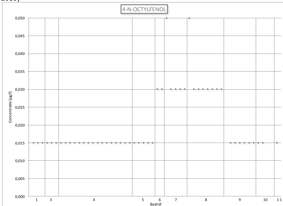
Figuur 82: Lozingsgegevens voor 4-n-octylfenol (Vlaanderen, 2005 – (september) 2010)
