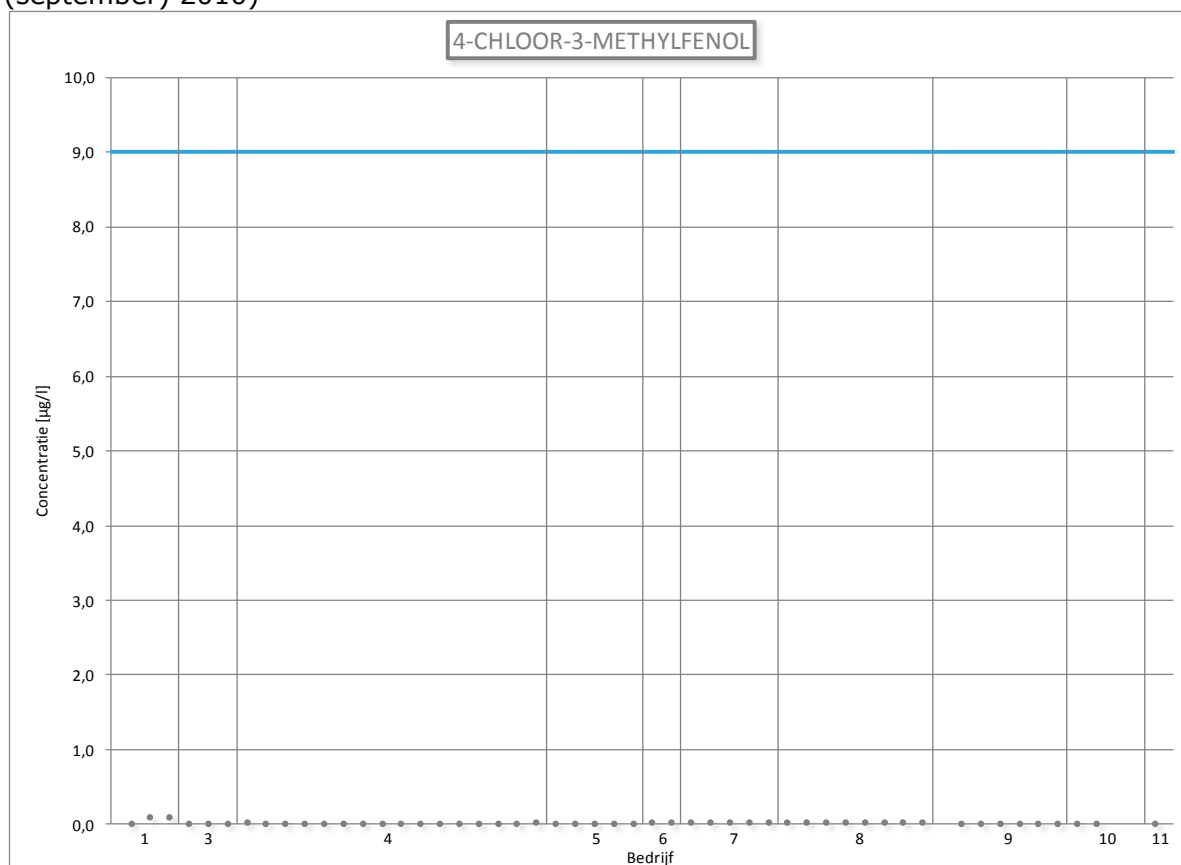
Figuur 80: Lozingsgegevens voor 4-chloor-3-methylfenol (Vlaanderen, 2005 – (september) 2010)
