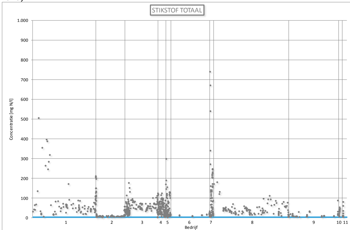
Figuur 16: Lozingsgegevens voor stikstof totaal (Vlaanderen, 2005 – (september) 2010)
