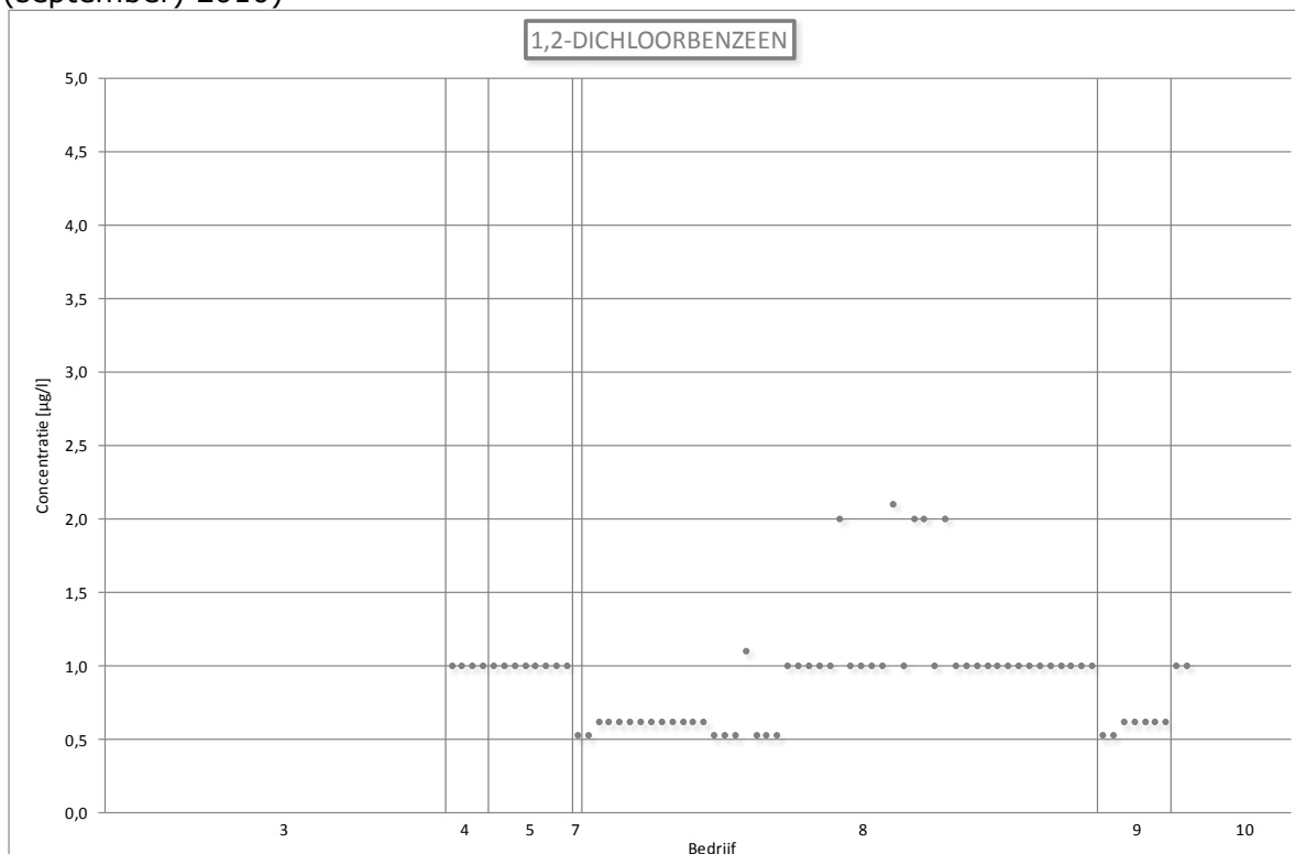
Figuur 104: Lozingsgegevens voor 1,2-dichloorbenzeen (Vlaanderen, 2005 – (september) 2010)
