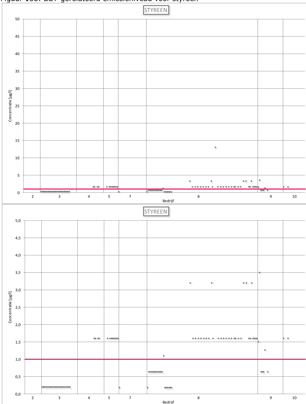
Figuur 158: BBT-gerelateerd emissieniveau voor styreen
