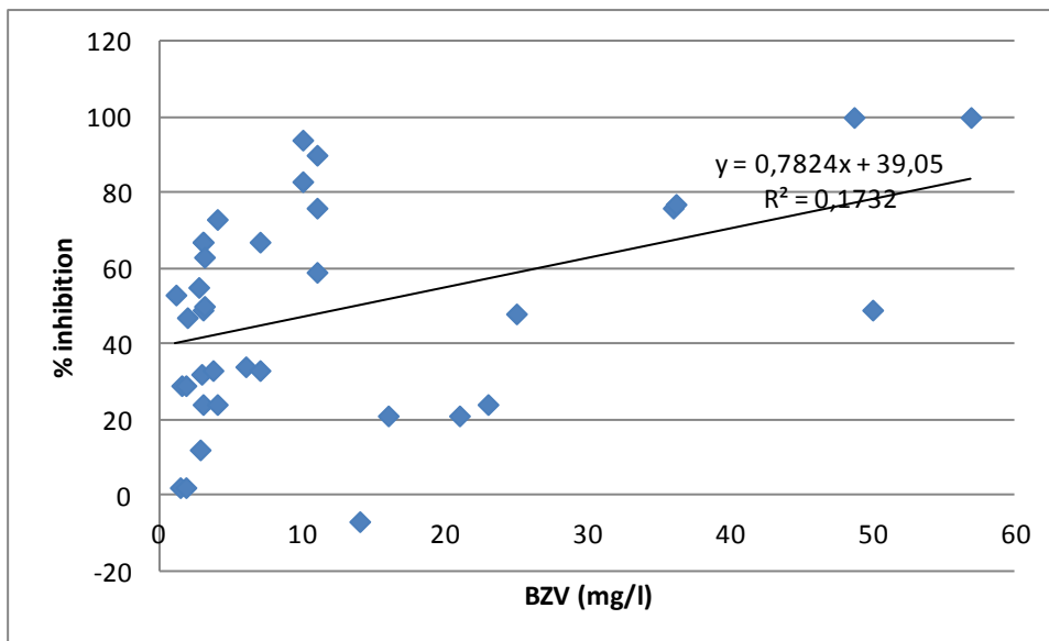
Figuur 122: Correlatie tussen toxiciteit en BZV
