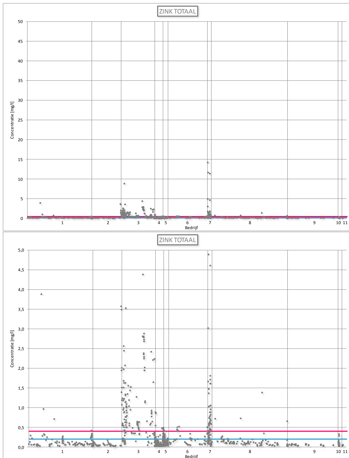
Figuur 148: BBT-gerelateerd emissieniveau voor zink totaal
