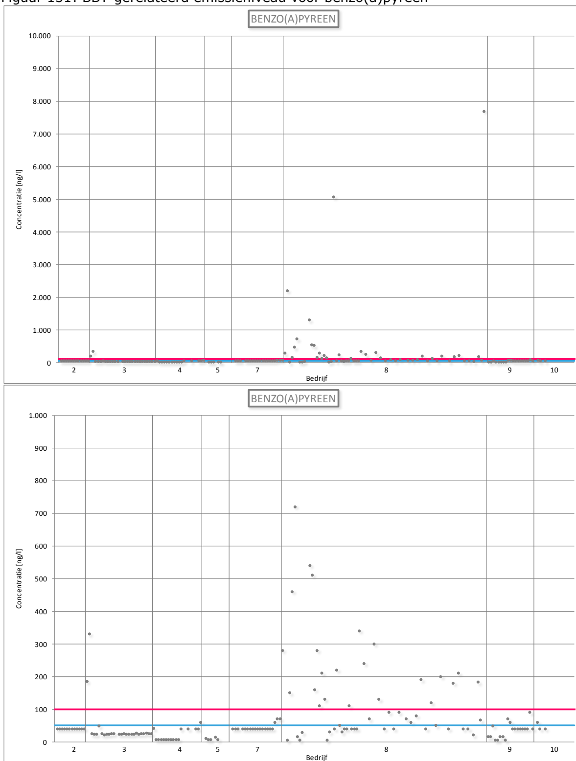
Figuur 151: BBT-gerelateerd emissieniveau voor benzo(a)pyreen
