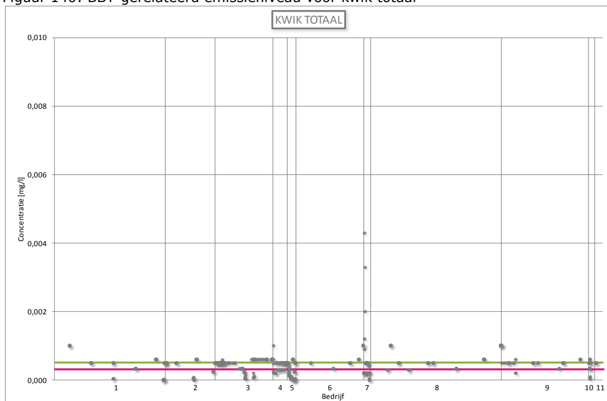
Figuur 140: BBT-gerelateerd emissieniveau voor kwik totaal
