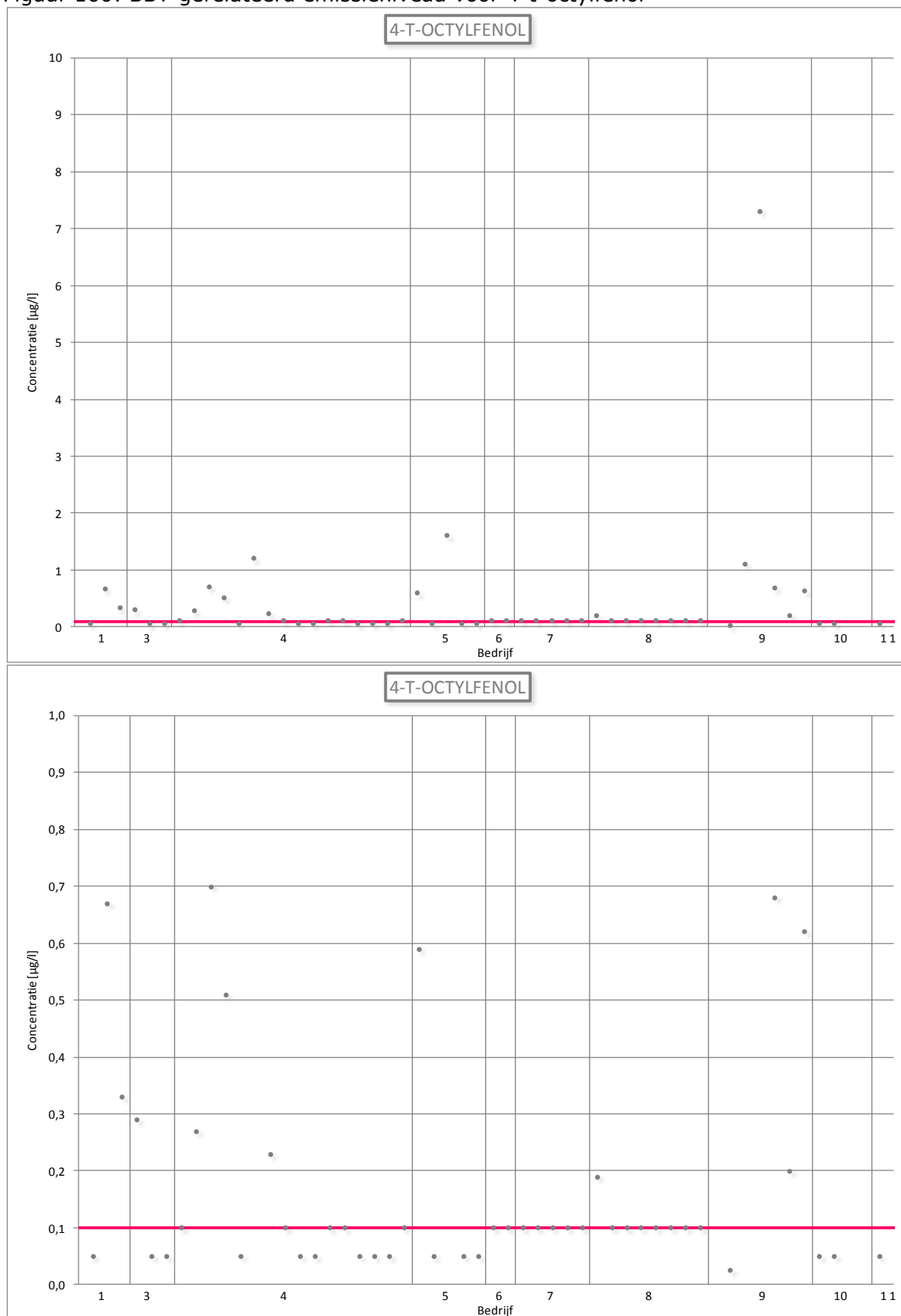
Figuur 160: BBT-gerelateerd emissieniveau voor 4-t-octylfenol
