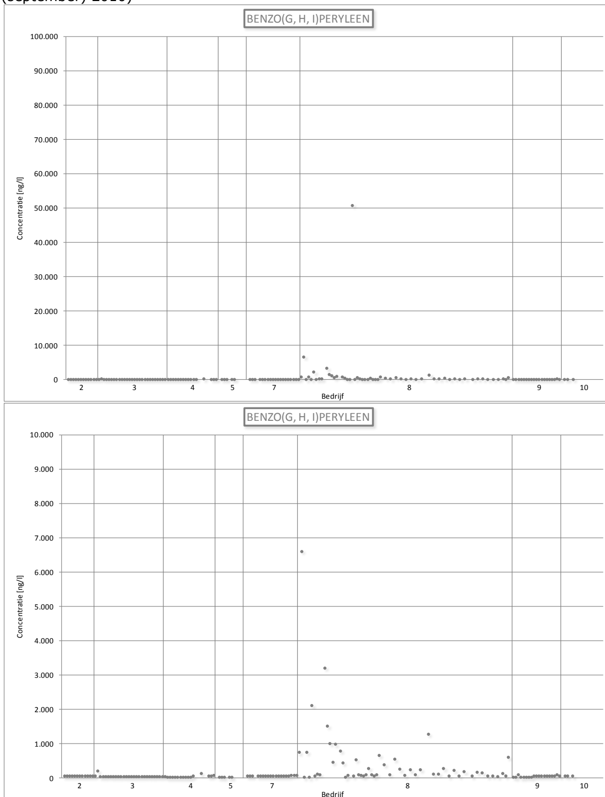
Figuur 54: Lozingsgegevens voor benzo(g,h,i)peryleen (Vlaanderen, 2005 – (september) 2010)
