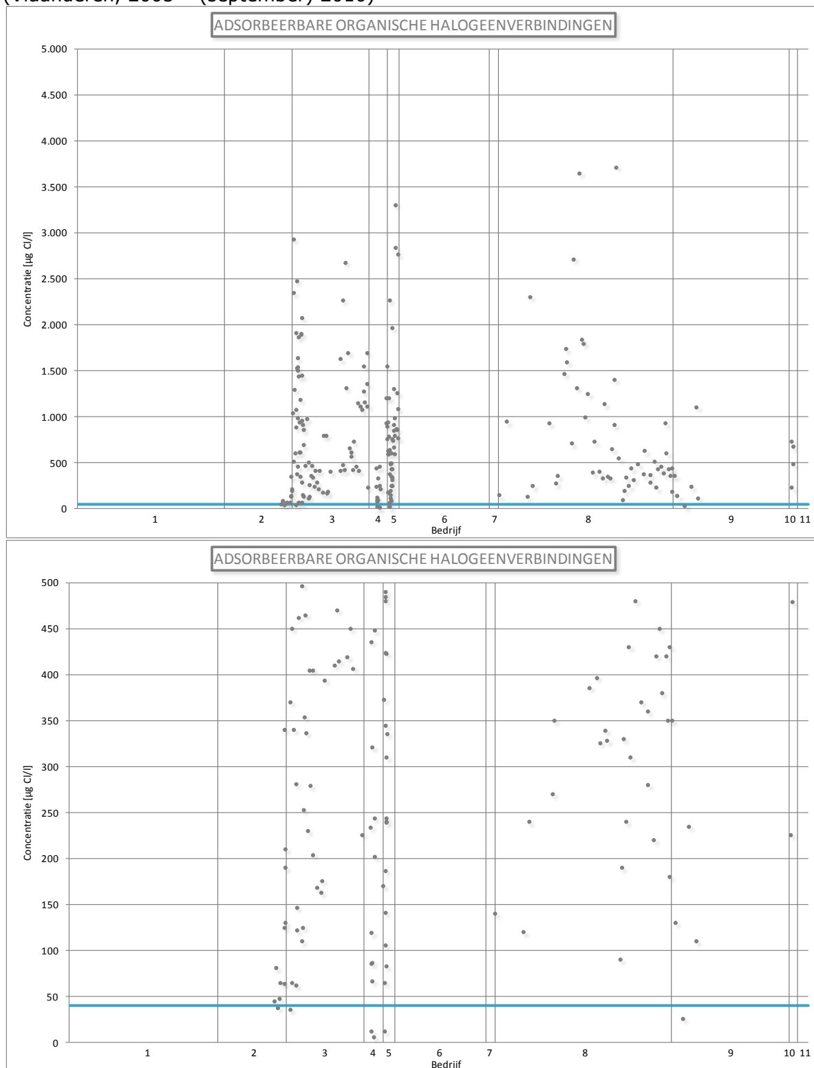
Figuur 45: Lozingsgegevens voor adsorbeerbare organische halogeenverbindingen (Vlaanderen, 2005 – (september) 2010)
