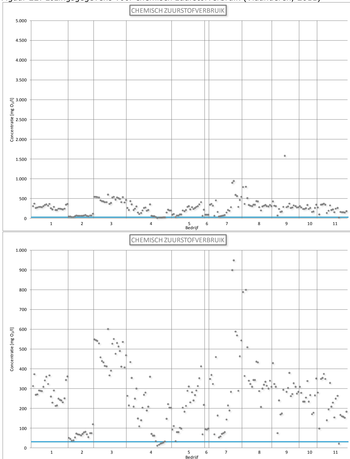
Figuur 22: Lozingsgegevens voor chemisch zuurstofverbruik (Vlaanderen, 2011)
