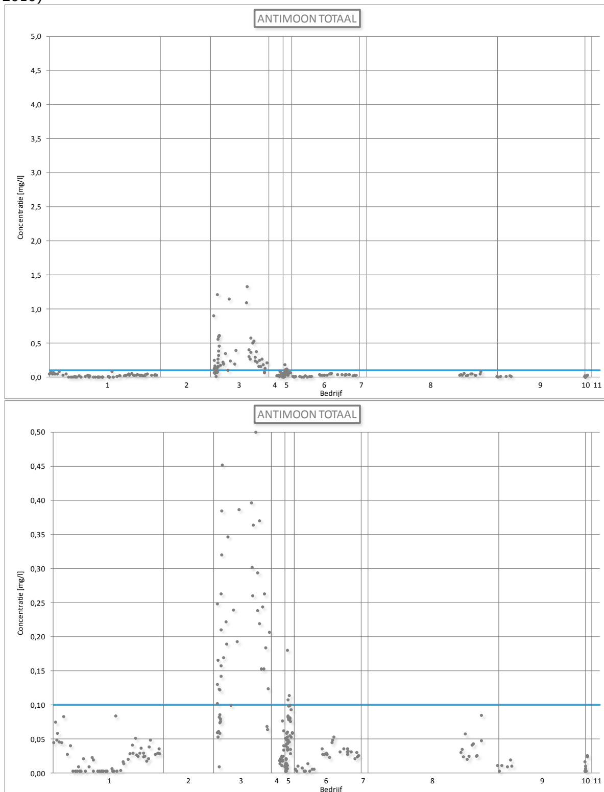
Figuur 39: Lozingsgegevens voor antimoon totaal (Vlaanderen, 2005 – (september) 2010)
