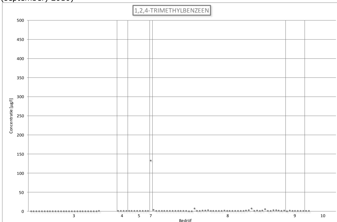
Figuur 87: Lozingsgegevens voor 1,2,4-trimethylbenzeen (Vlaanderen, 2005 – (september) 2010)
