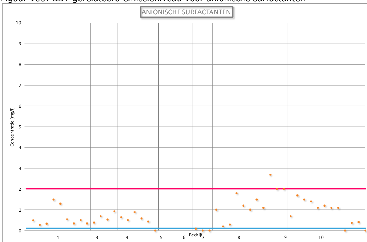
Figuur 163: BBT-gerelateerd emissieniveau voor anionische surfactanten
