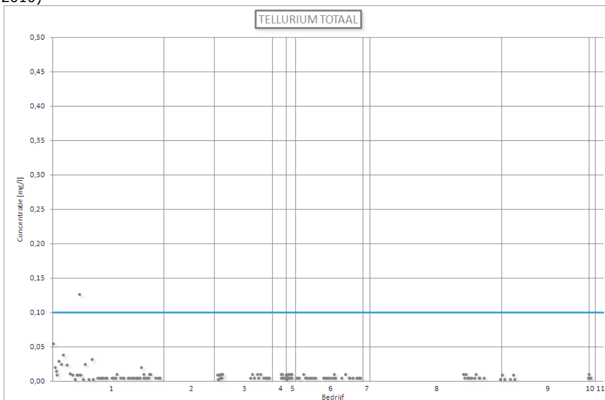
Figuur 41: Lozingsgegevens voor tellurium totaal (Vlaanderen, 2005 – (september) 2010)
