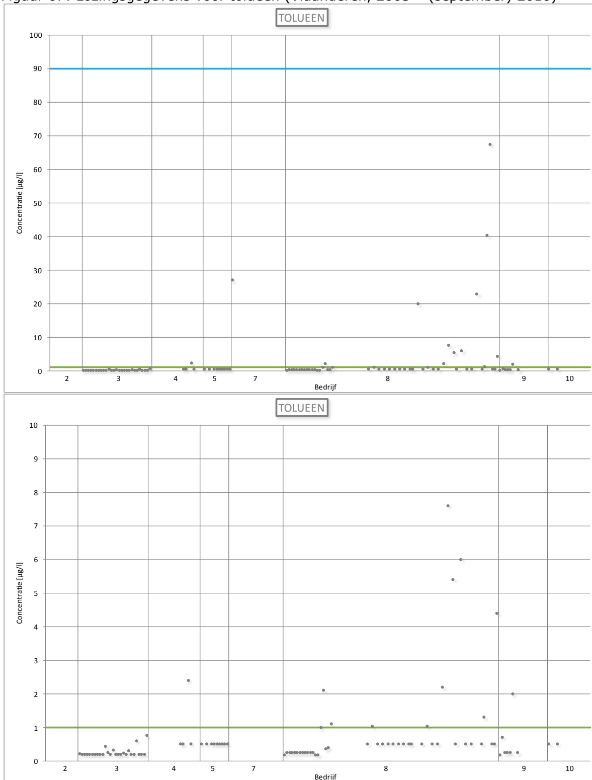
Figuur 67: Lozingsgegevens voor tolueen (Vlaanderen, 2005 – (september) 2010)
