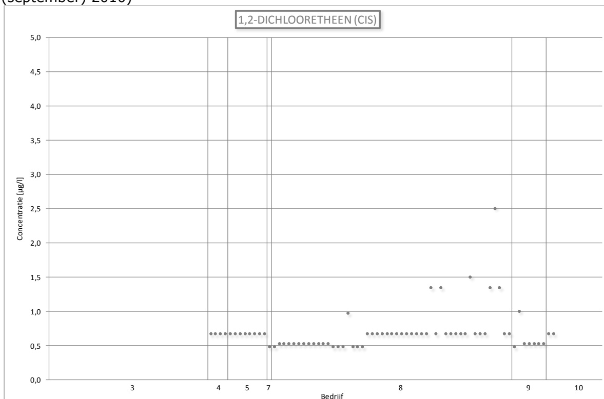
Figuur 93: Lozingsgegevens voor 1,2-dichlooretheen (cis) (Vlaanderen, 2005 – (september) 2010)
