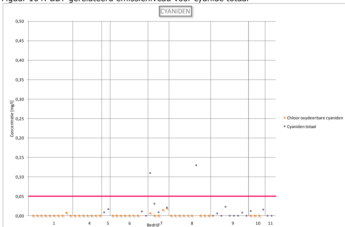
Figuur 164: BBT-gerelateerd emissieniveau voor cyanide totaal
