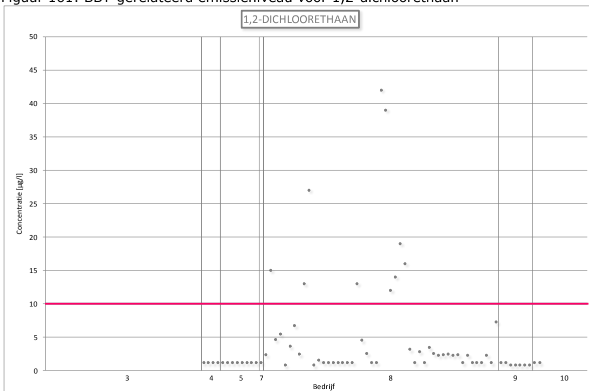
Figuur 161: BBT-gerelateerd emissieniveau voor 1,2-dichloorethaan
