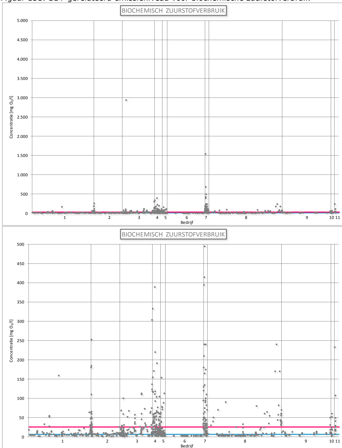
Figuur 131: BBT-gerelateerd emissieniveau voor biochemische zuurstofverbruik
