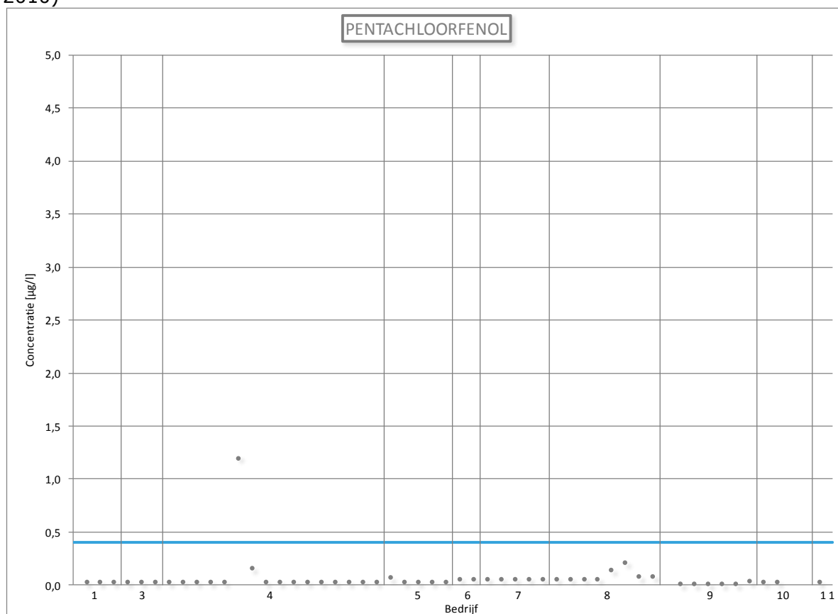
Figuur 79: Lozingsgegevens voor pentachloorfenol (Vlaanderen, 2005 – (september) 2010)
