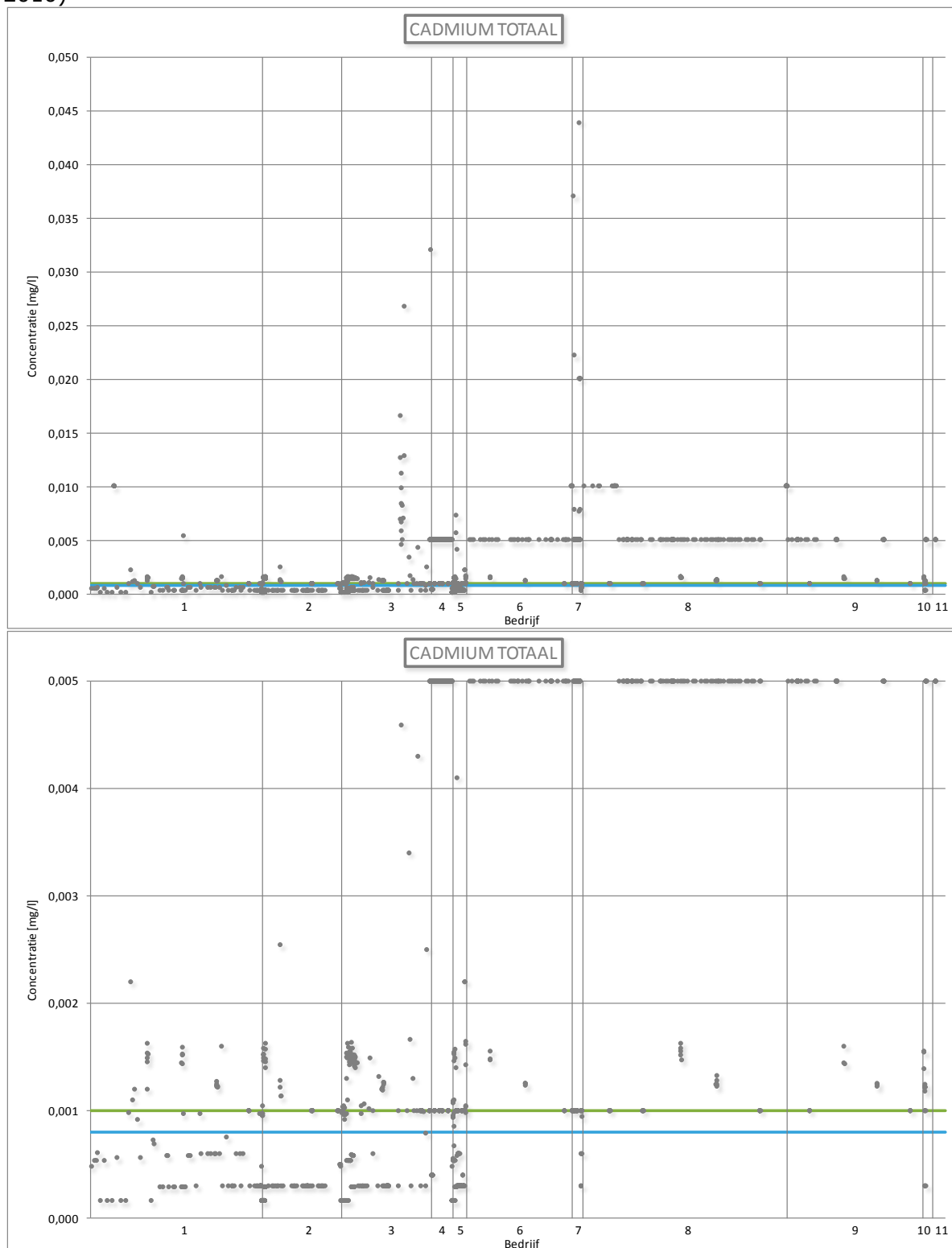
Figuur 28: Lozingsgegevens voor cadmium totaal (Vlaanderen, 2005 – (september) 2010)
