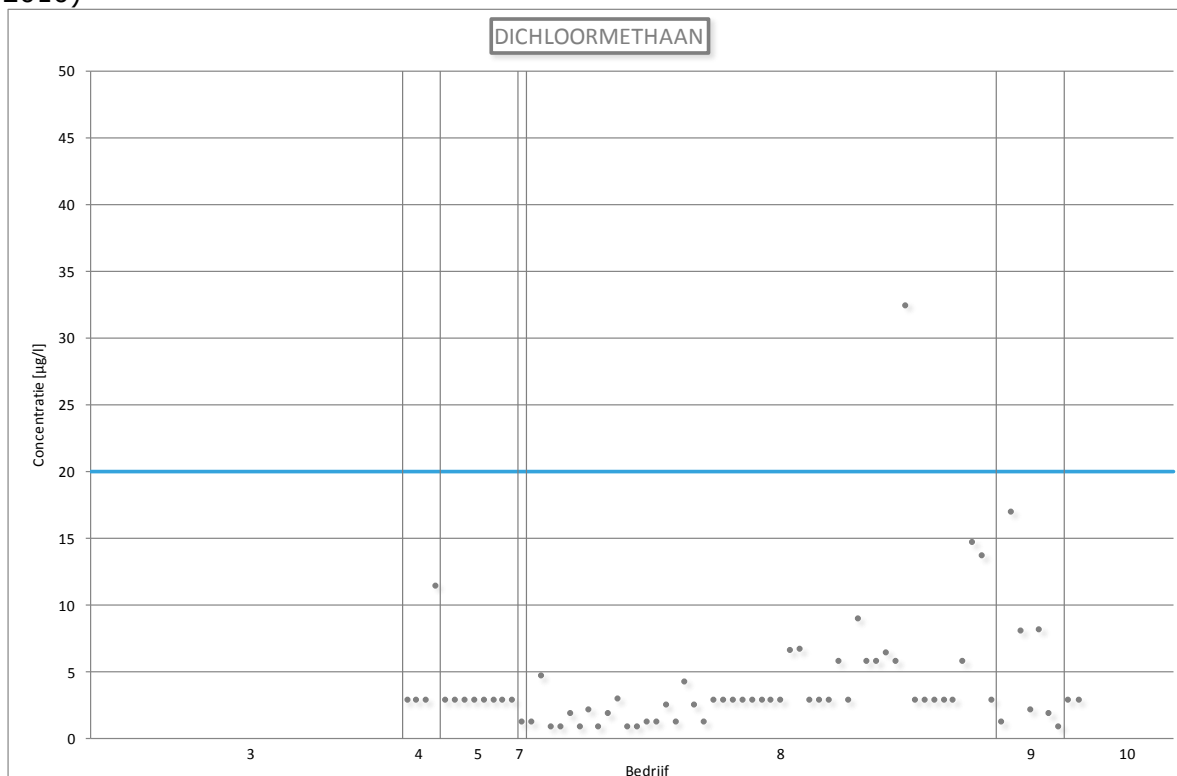
Figuur 98: Lozingsgegevens voor dichloormethaan (Vlaanderen, 2005 – (september) 2010)
