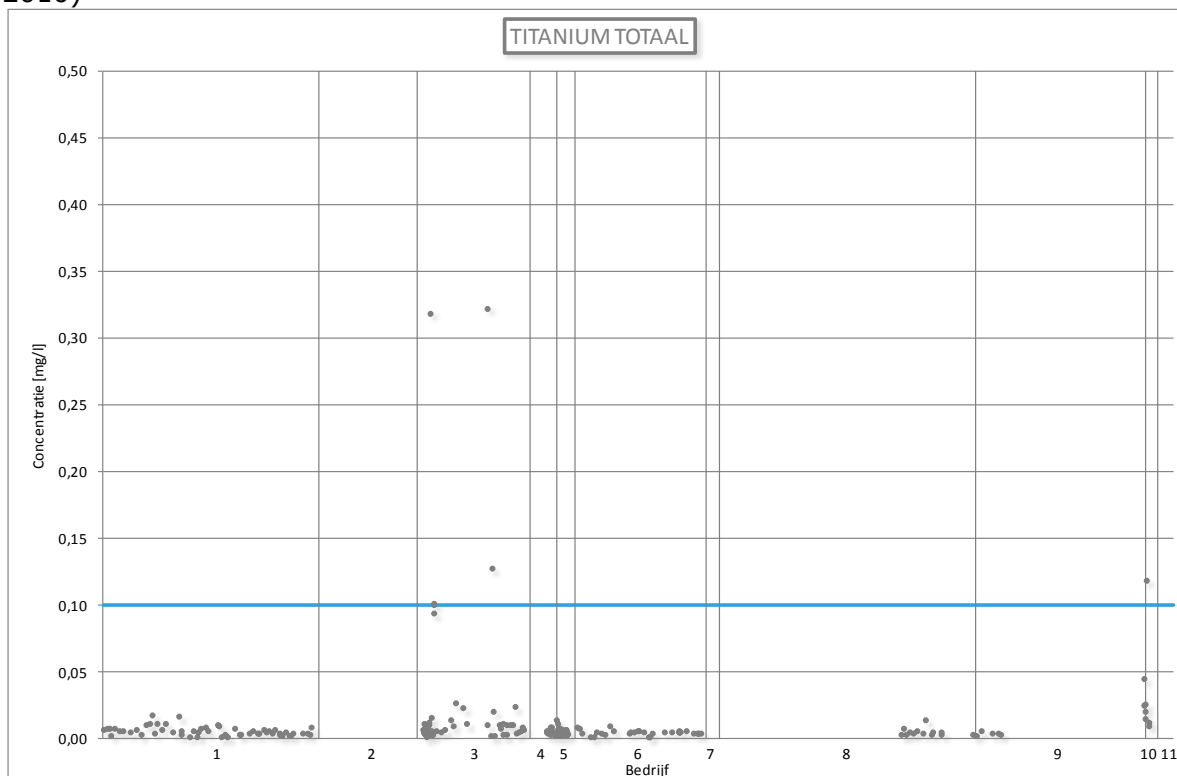
Figuur 42: Lozingsgegevens voor titanium totaal (Vlaanderen, 2005 – (september) 2010)
