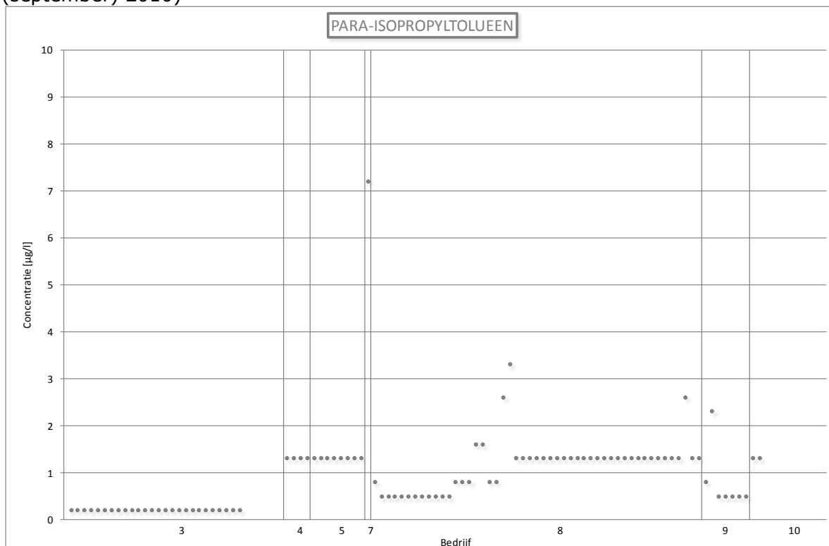
Figuur 86: Lozingsgegevens voor para-isopropytolueen (Vlaanderen, 2005 – (september) 2010)
