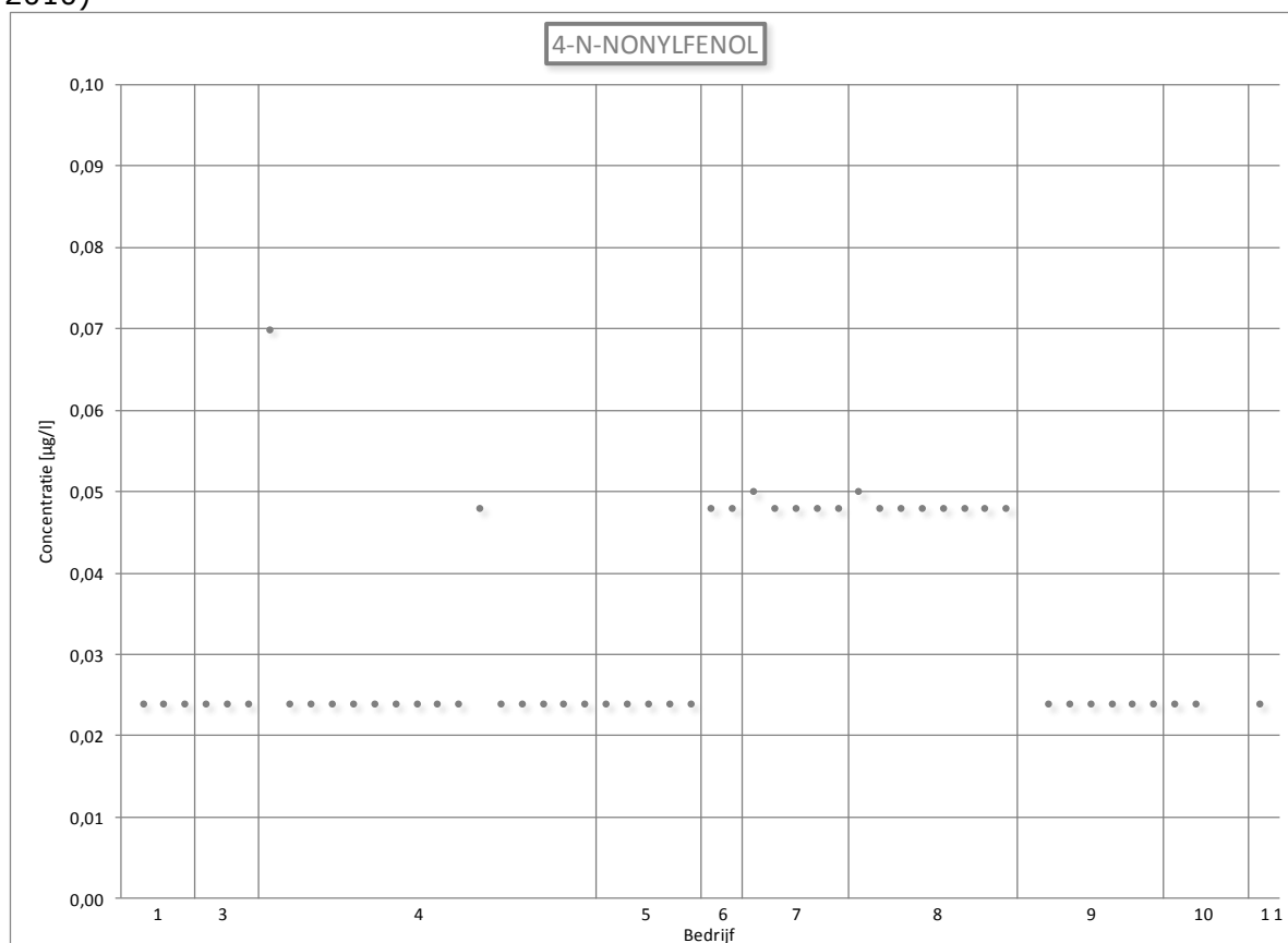
Figuur 83: Lozingsgegevens voor 4-n-nonylfenol (Vlaanderen, 2005 – (september) 2010)
