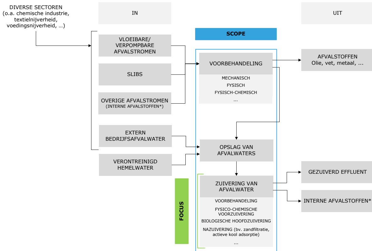
Figuur 1: Scope & focus van BBT-studie voor verwerking van externe bedrijfsafvalwaters & vloeibare/slibachtige bedrijfsafvalstromen Bron: BBT-kenniscentrum
