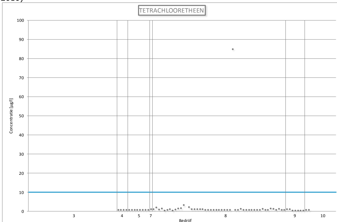
Figuur 99: Lozingsgegevens voor tetrachlooretheen (Vlaanderen, 2005 – (september) 2010)
