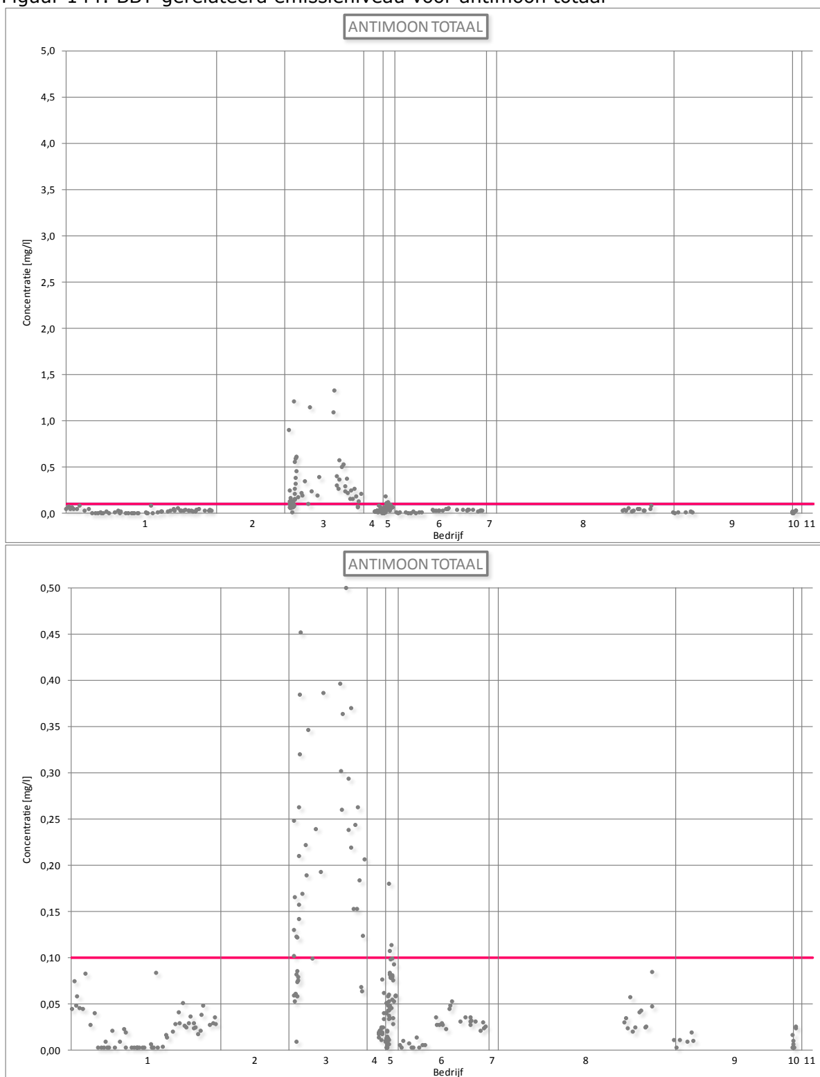
Figuur 144: BBT-gerelateerd emissieniveau voor antimoon totaal
