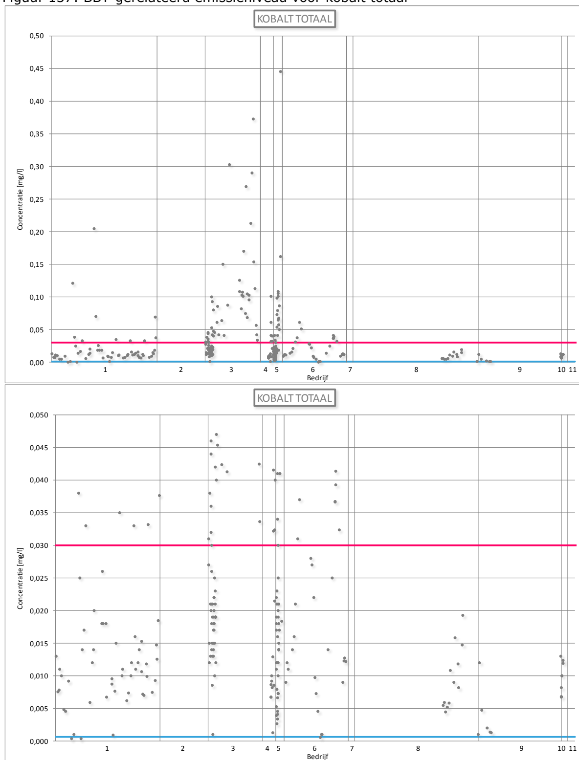
Figuur 137: BBT-gerelateerd emissieniveau voor kobalt totaal
