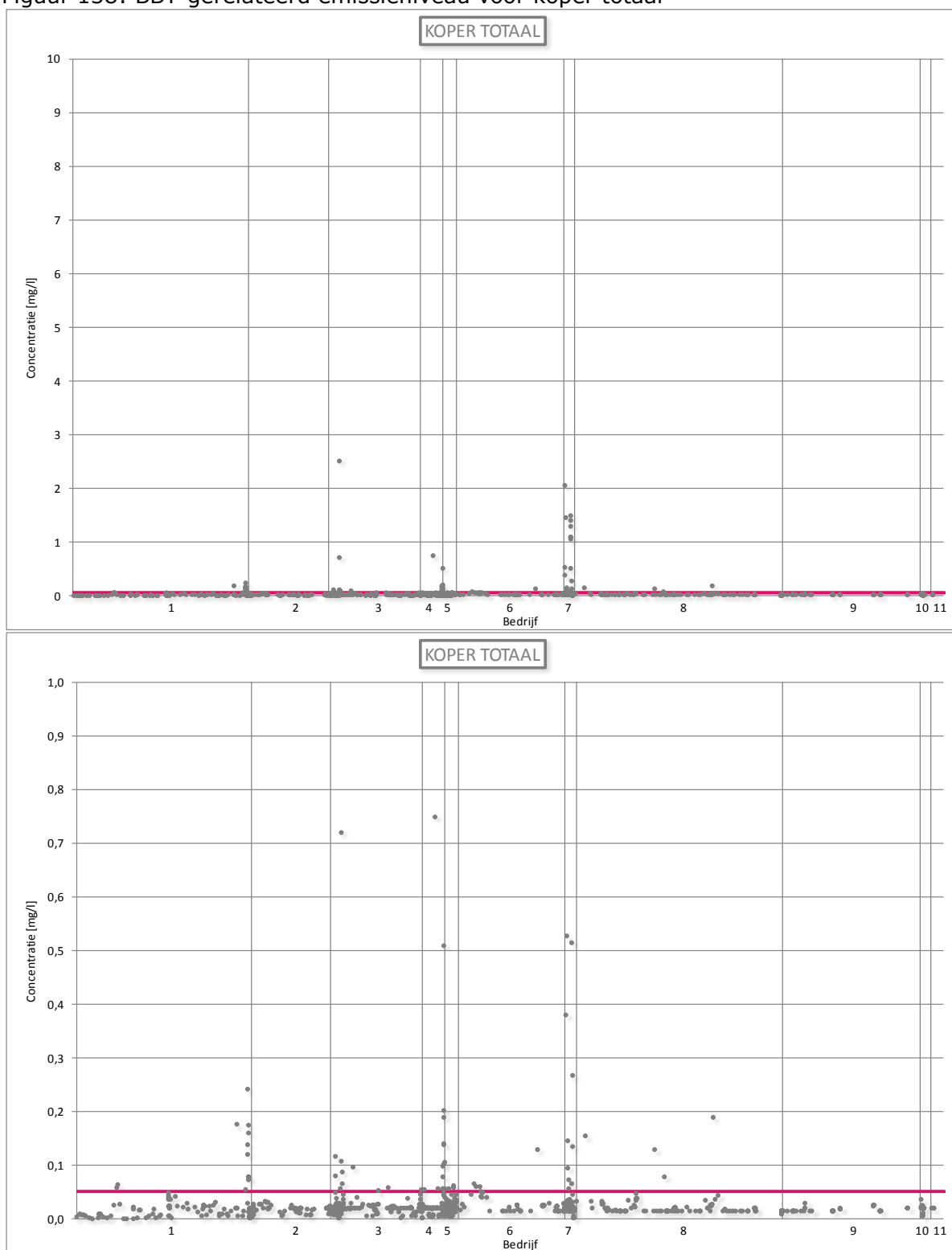
Figuur 138: BBT-gerelateerd emissieniveau voor koper totaal
