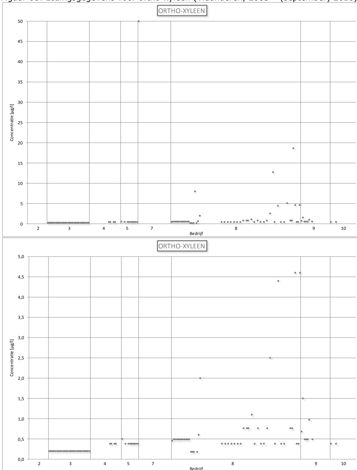
Figuur 68: Lozingsgegevens voor ortho-xyleen (Vlaanderen, 2005 – (september) 2010)
