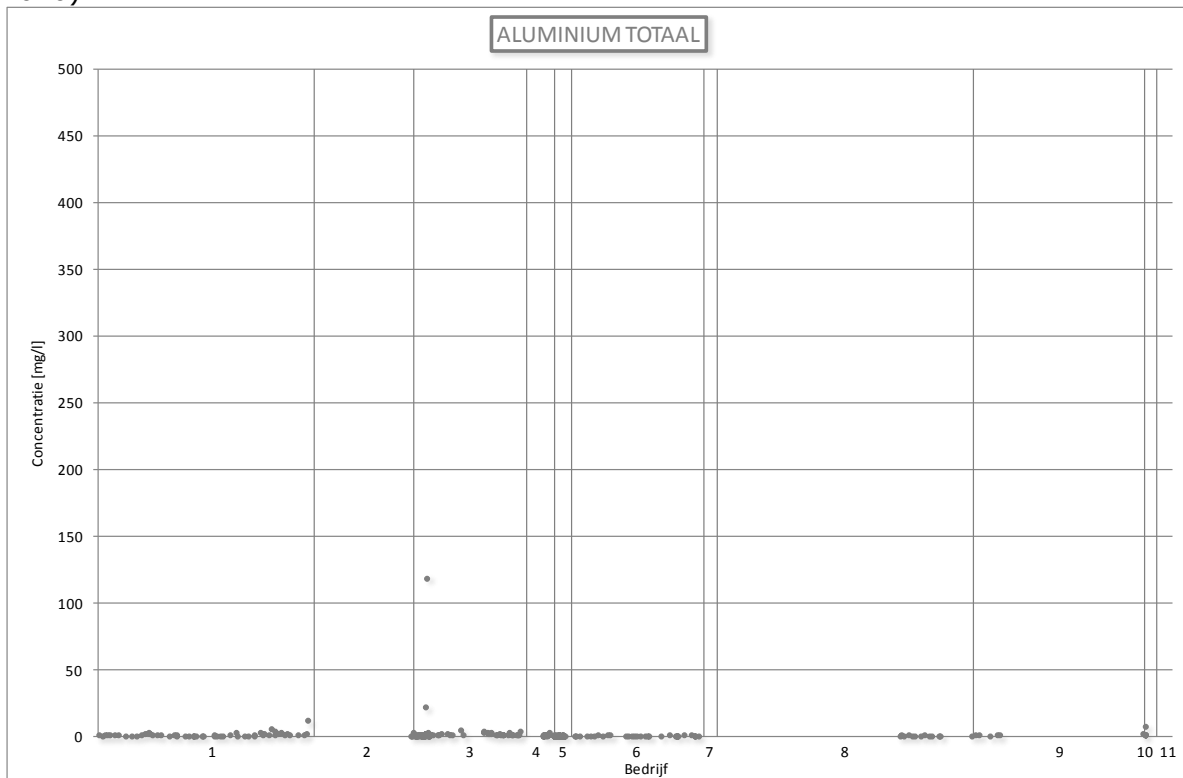
Figuur 24: Lozingsgegevens voor aluminium totaal (Vlaanderen, 2005 – (september) 2010)
