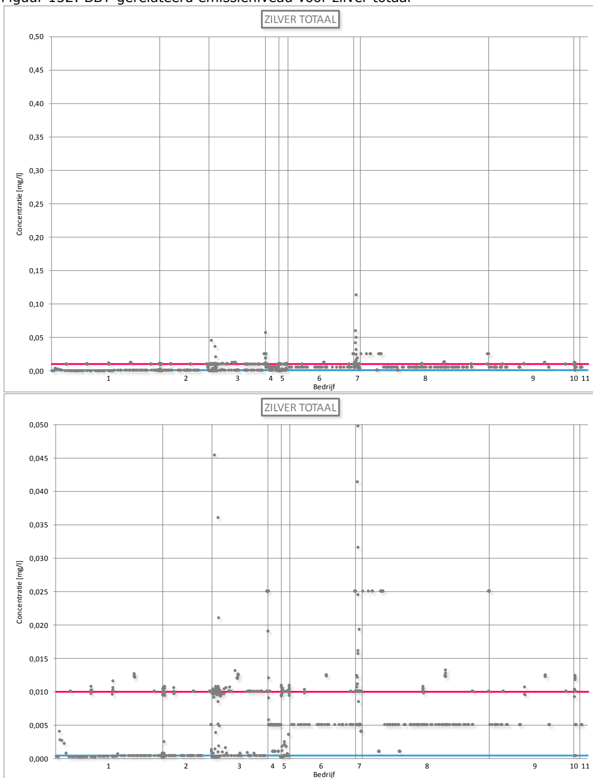
Figuur 132: BBT-gerelateerd emissieniveau voor zilver totaal
