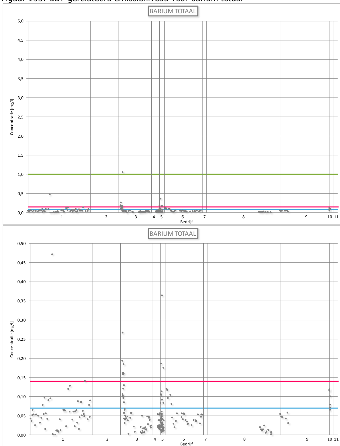
Figuur 135: BBT-gerelateerd emissieniveau voor barium totaal
