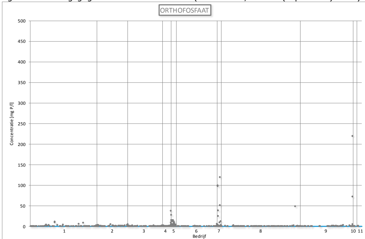
Figuur 11: Lozingsgegevens voor orthofosfaat (Vlaanderen, 2005 – (september) 2010)
