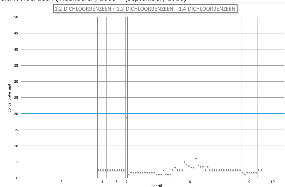
Figuur 107: Lozingsgegevens voor 1,2-dichloorbenzeen & 1,3-dichloorbenzeen & 1,4-dichloorbenzeen (Vlaanderen, 2005 – (september) 2010)
