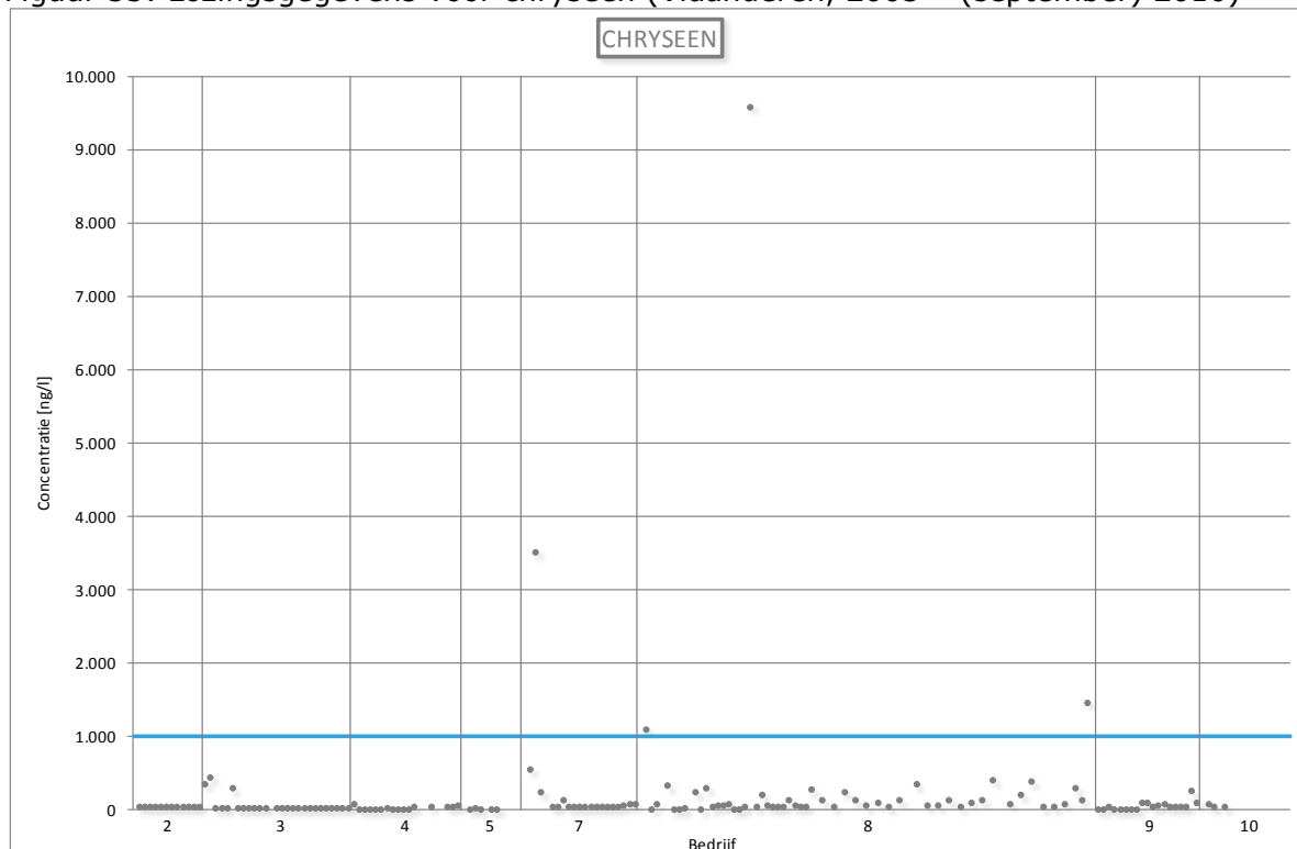
Figuur 55: Lozingsgegevens voor chryseen (Vlaanderen, 2005 – (september) 2010)
