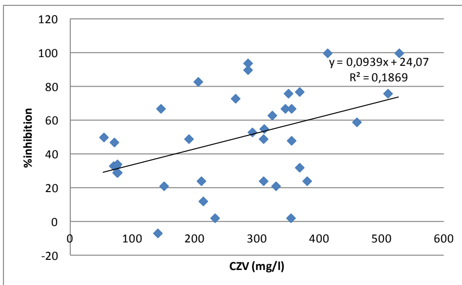
Figuur 123: Correlatie tussen toxiciteit en CZV
