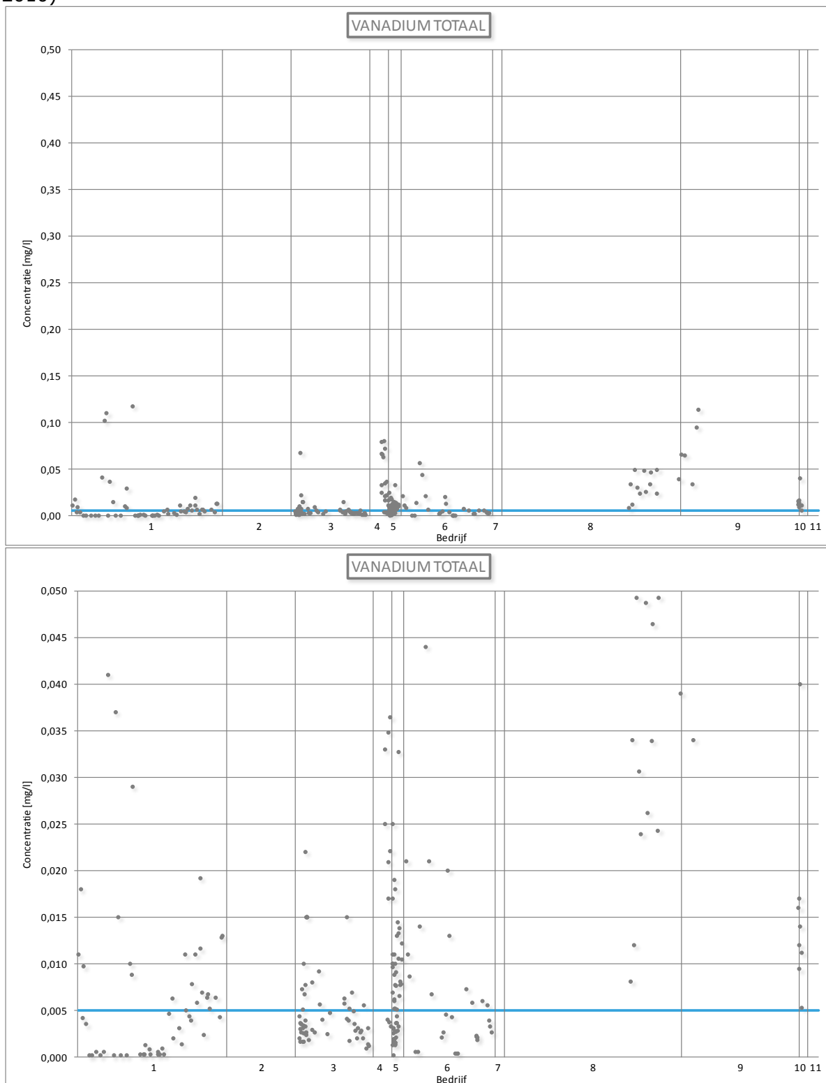
Figuur 43: Lozingsgegevens voor vanadium totaal (Vlaanderen, 2005 – (september) 2010)
