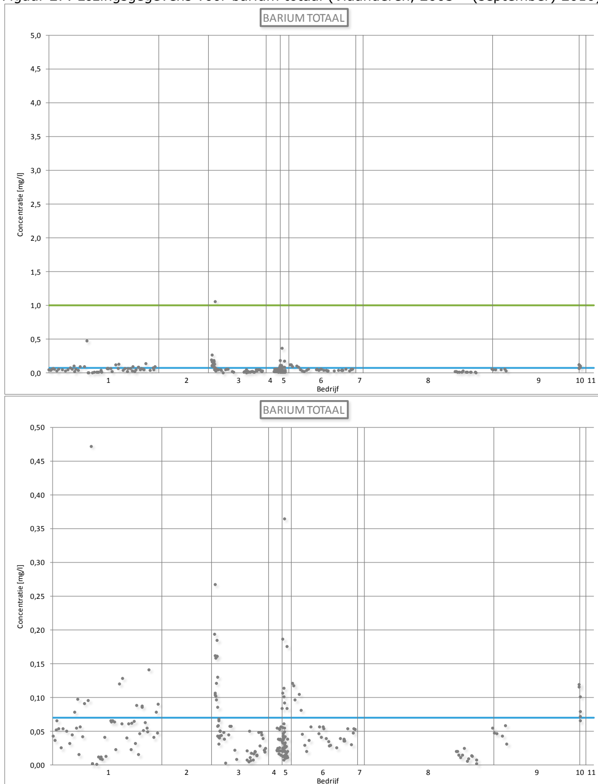
Figuur 27: Lozingsgegevens voor barium totaal (Vlaanderen, 2005 – (september) 2010)
