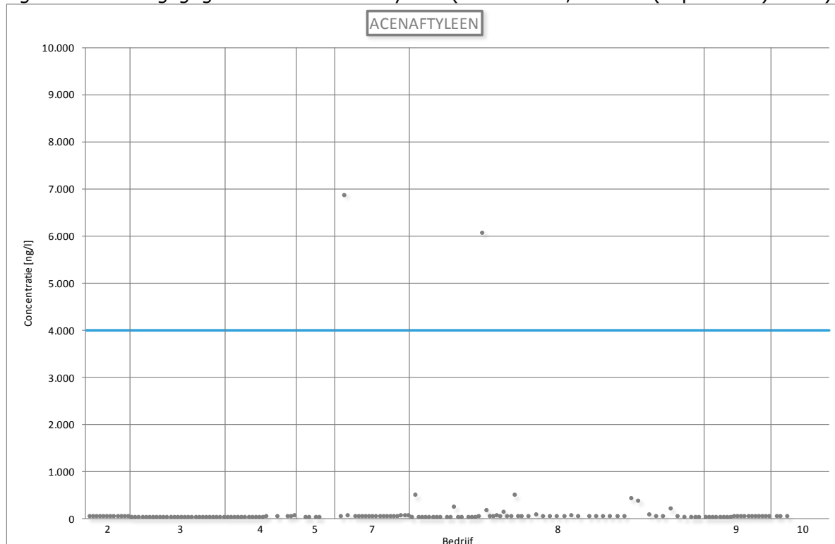
Figuur 47: Lozingsgegevens voor acenaftyleen (Vlaanderen, 2005 – (september) 2010)
