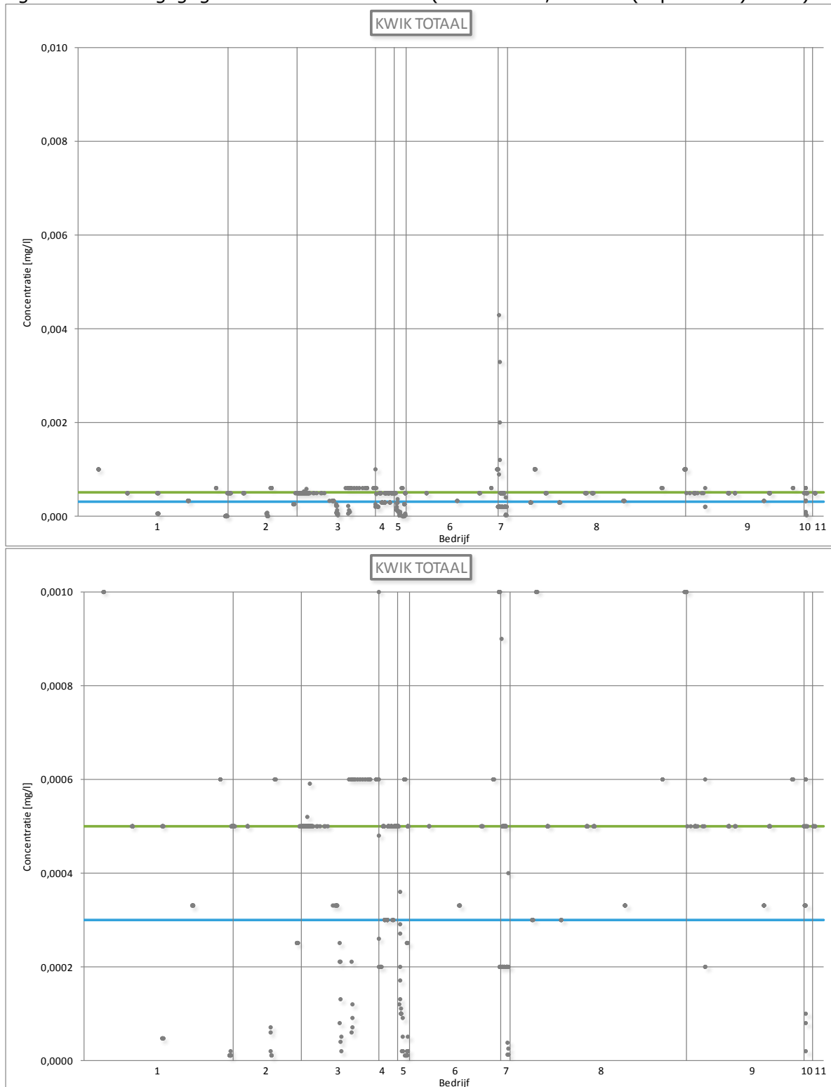
Figuur 34: Lozingsgegevens voor kwik totaal (Vlaanderen, 2005 – (september) 2010)
