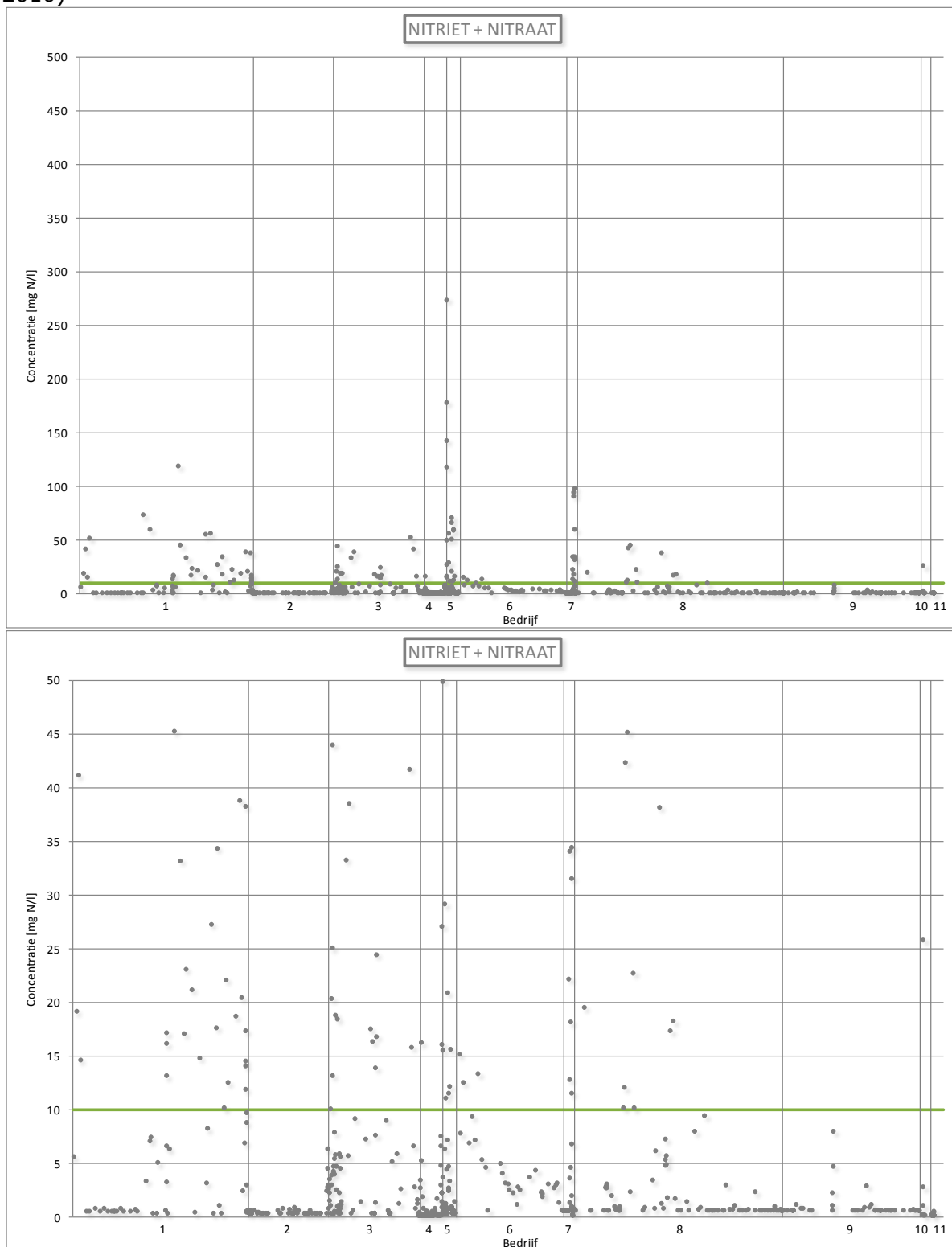
Figuur 10: Lozingsgegevens voor nitriet & nitraat (Vlaanderen, 2005 – (september) 2010)
