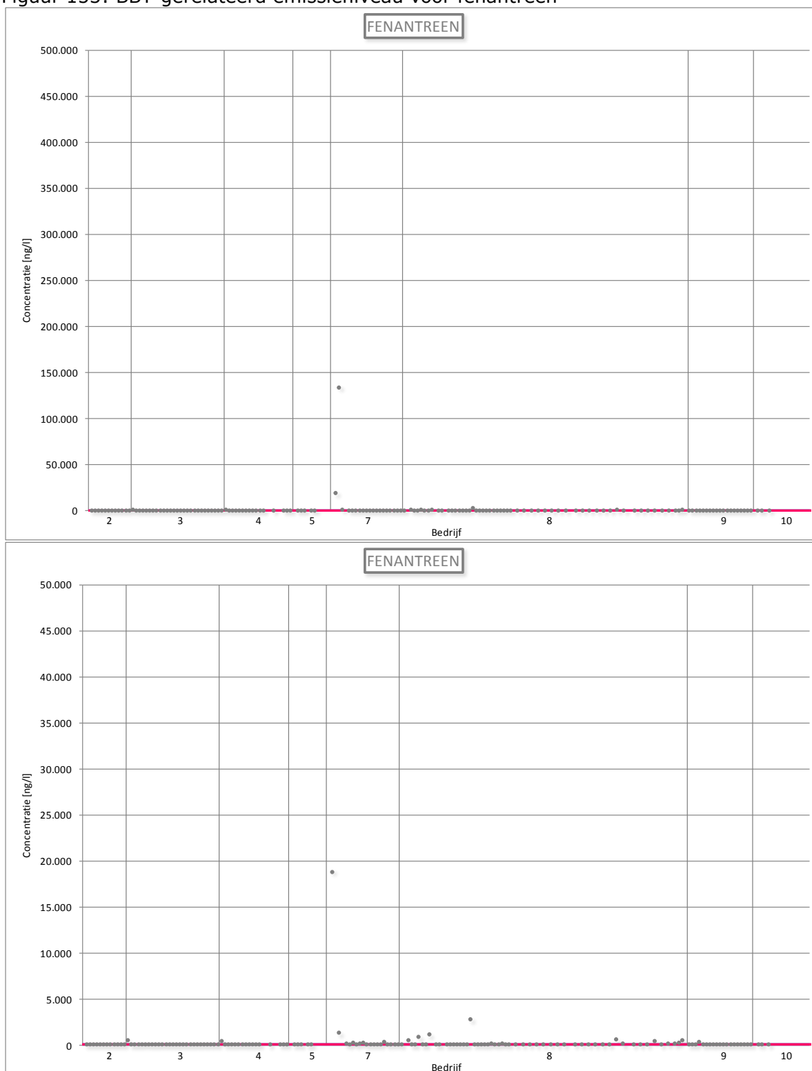
Figuur 153: BBT-gerelateerd emissieniveau voor fenantreen
