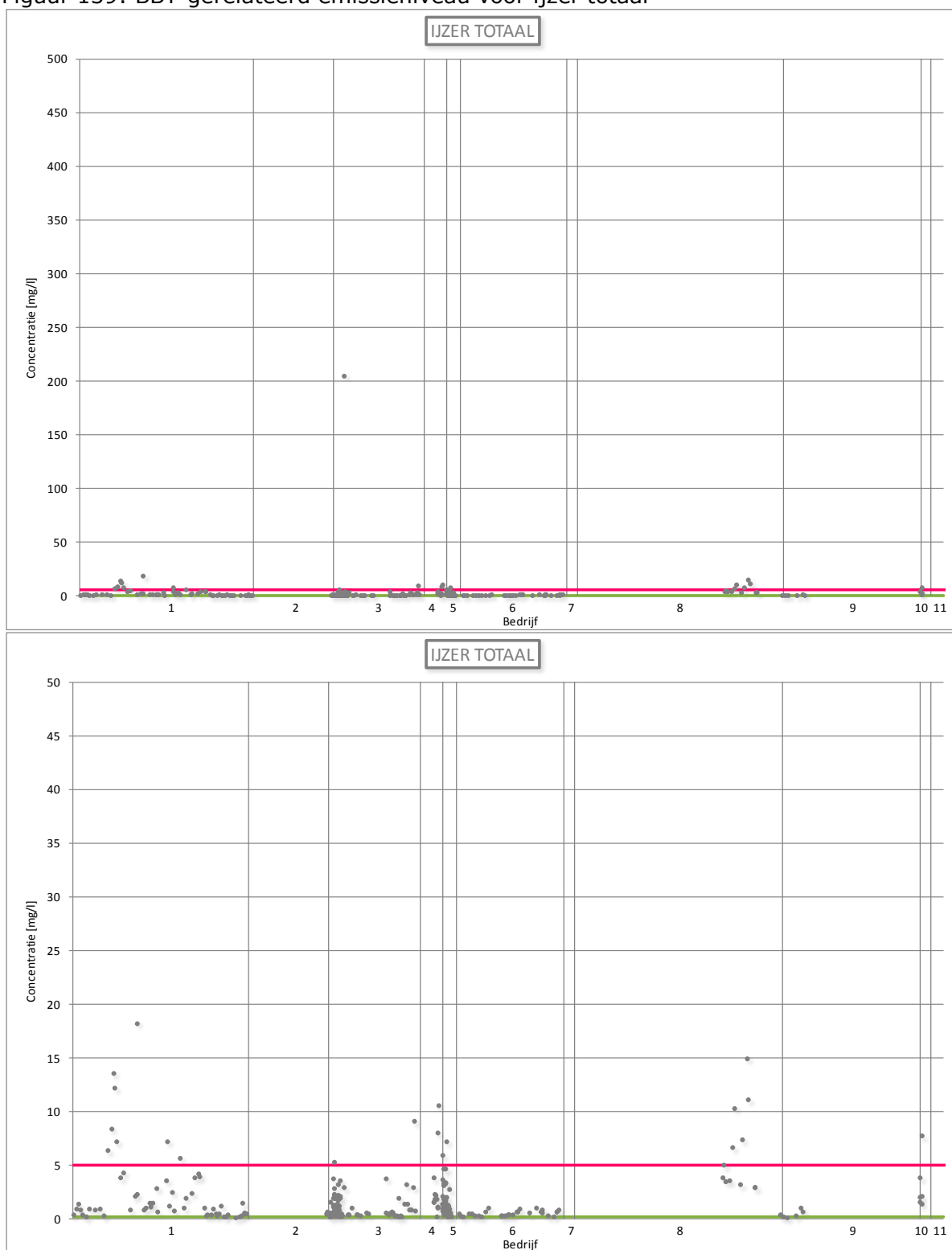
Figuur 139: BBT-gerelateerd emissieniveau voor ijzer totaal
