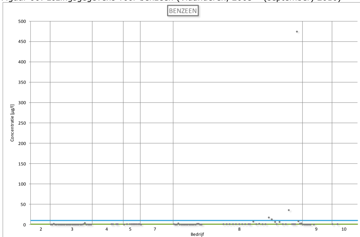
Figuur 66: Lozingsgegevens voor benzeen (Vlaanderen, 2005 – (september) 2010)
