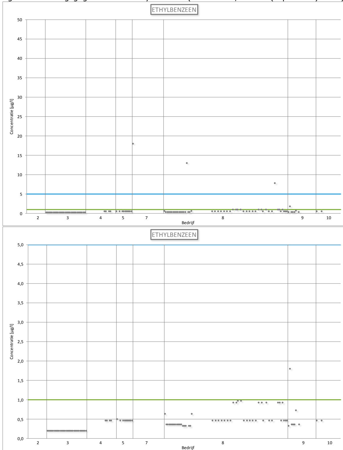
Figuur 71: Lozingsgegevens voor ethylbenzeen (Vlaanderen, 2005 – (september) 2010)
