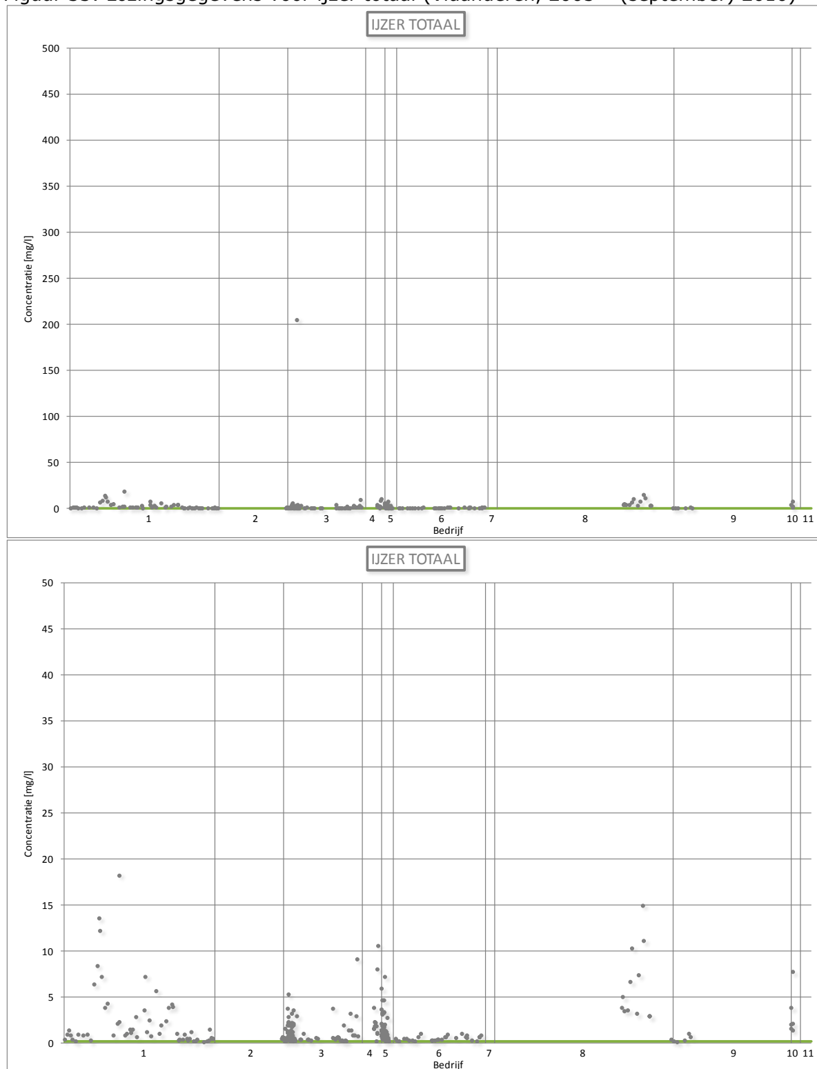
Figuur 33: Lozingsgegevens voor ijzer totaal (Vlaanderen, 2005 – (september) 2010)
