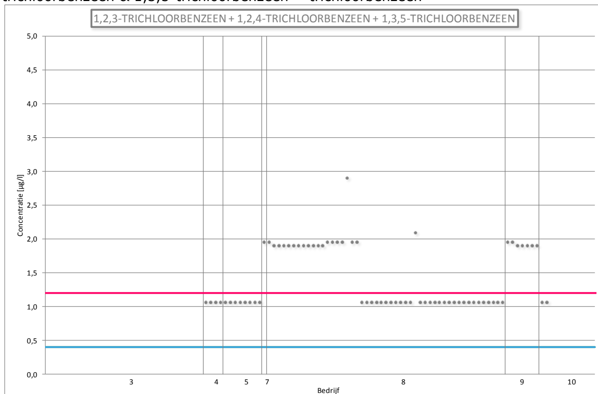
Figuur 162: BBT-gerelateerd emissieniveau voor 1,2,3-trichloorbenzeen & 1,2,4-trichloorbenzeen & 1,3,5-trichloorbenzeen = trichloorbenzeen
