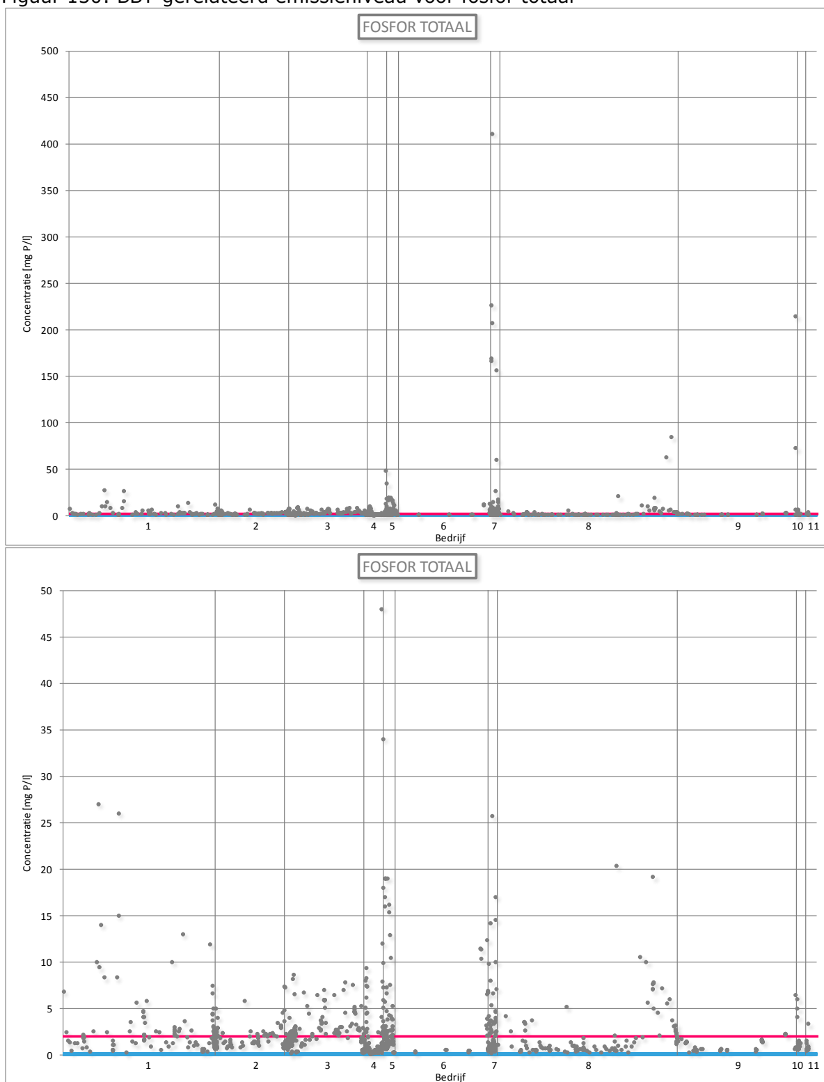
Figuur 130: BBT-gerelateerd emissieniveau voor fosfor totaal
