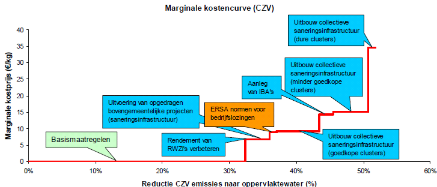
Figuur 120: Marginale kostencurve voor reductie van CZV naar oppervlaktewater
