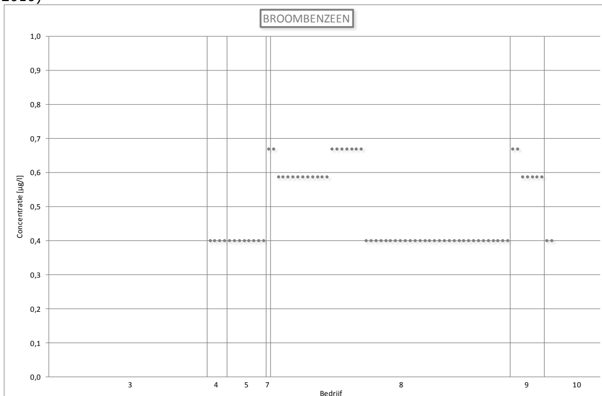
Figuur 102: Lozingsgegevens voor broombenzeen (Vlaanderen, 2005 – (september) 2010)
