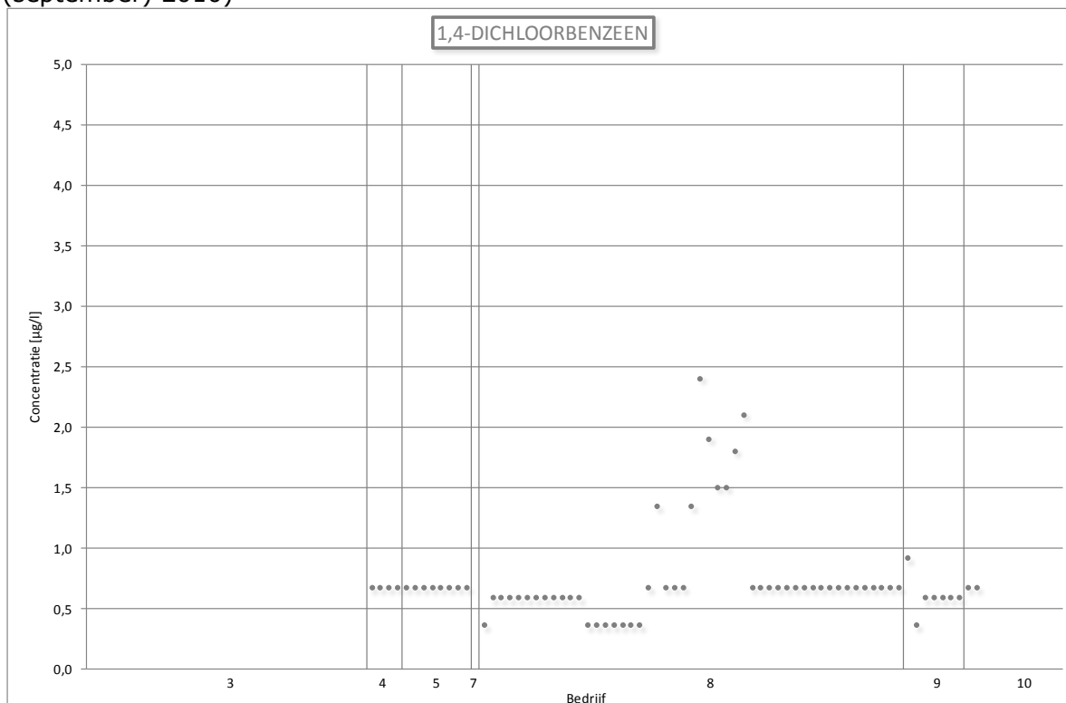
Figuur 106: Lozingsgegevens voor 1,4-dichloorbenzeen (Vlaanderen, 2005 – (september) 2010)
