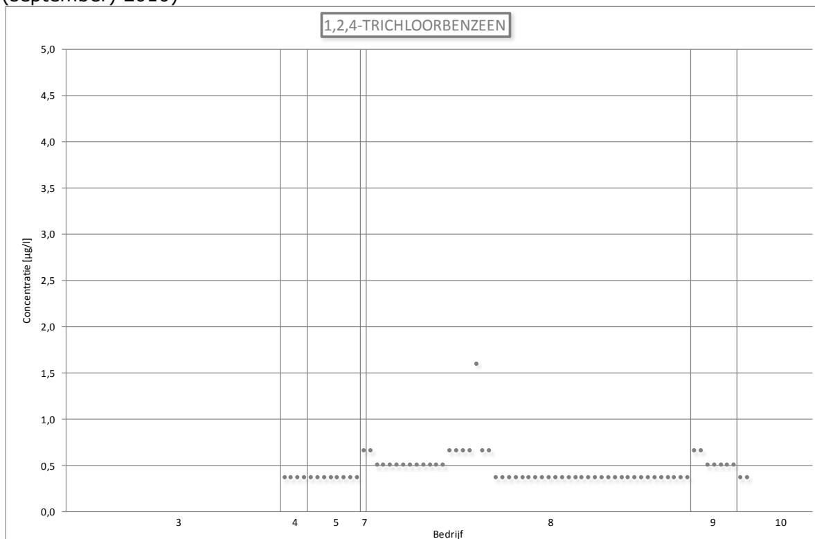
Figuur 109: Lozingsgegevens voor 1,2,4-trichloorbenzeen (Vlaanderen, 2005 – (september) 2010)
