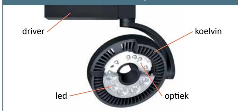
figuur 14 : opbouw van een verlichtingstoestel op basis van led met onder andere koelvinnen, leds, driver en optiek
