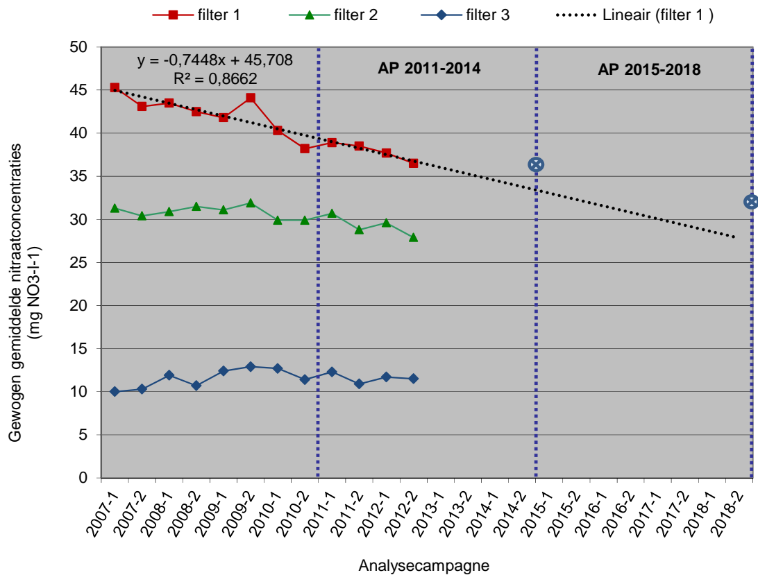
Figuur 52 Evolutie van de gewogen gemiddelde nitraatconcentraties ter hoogte van de drie filters in het freatische grondwatermeetnet vanaf 2007 met trendinterpolatie naar de volgende actieplanperiodes (AP).
