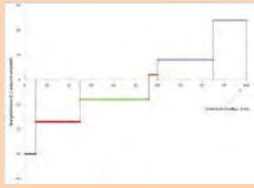
Marginale kostencurve
