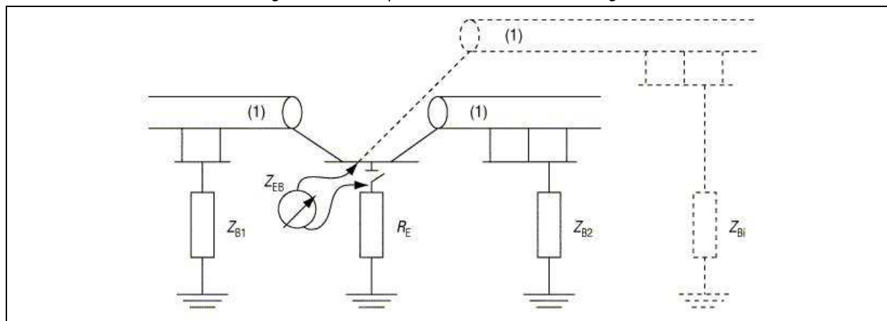
Figuur 2.10. Lusimpedantie van een aardverbinding Z_{EB}
