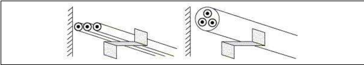
Figuur 5.6. Plaatsingswijzen van elektrische leidingen – Haken
