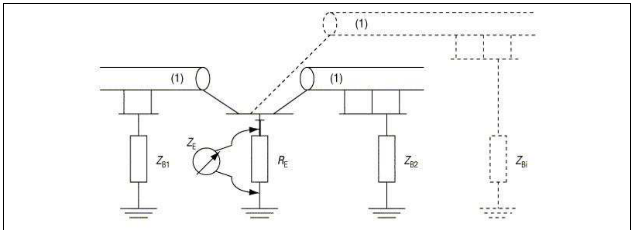
Figuur 2.8. Aardingsimpedantie Z_E
