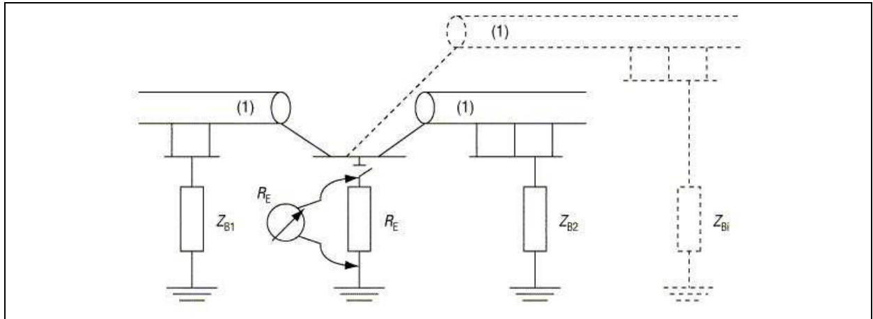
Figuur 2.7. Aardingsweerstand R_E
