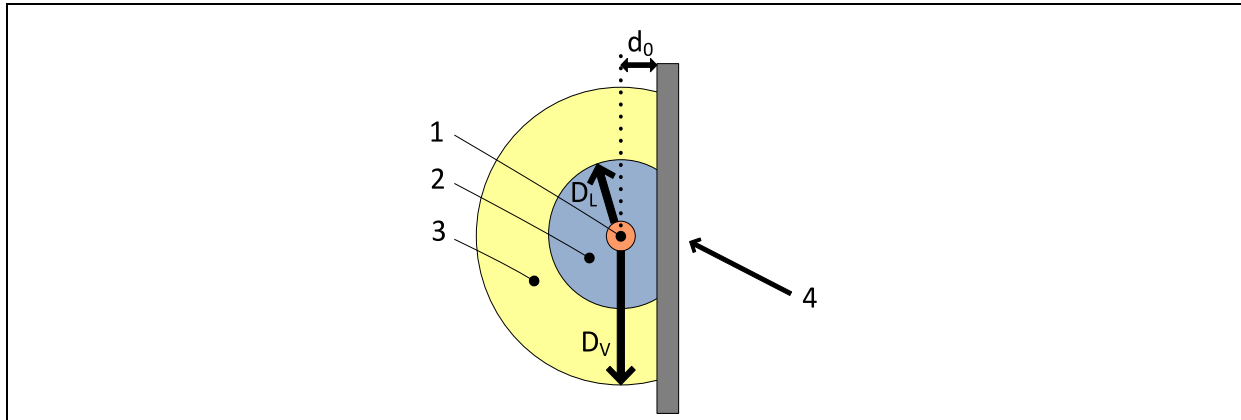
Figuur 2.22. Voorstelling van de zone onder spanning en de nabijheidszone met gearde, metalen bescherminrichting
