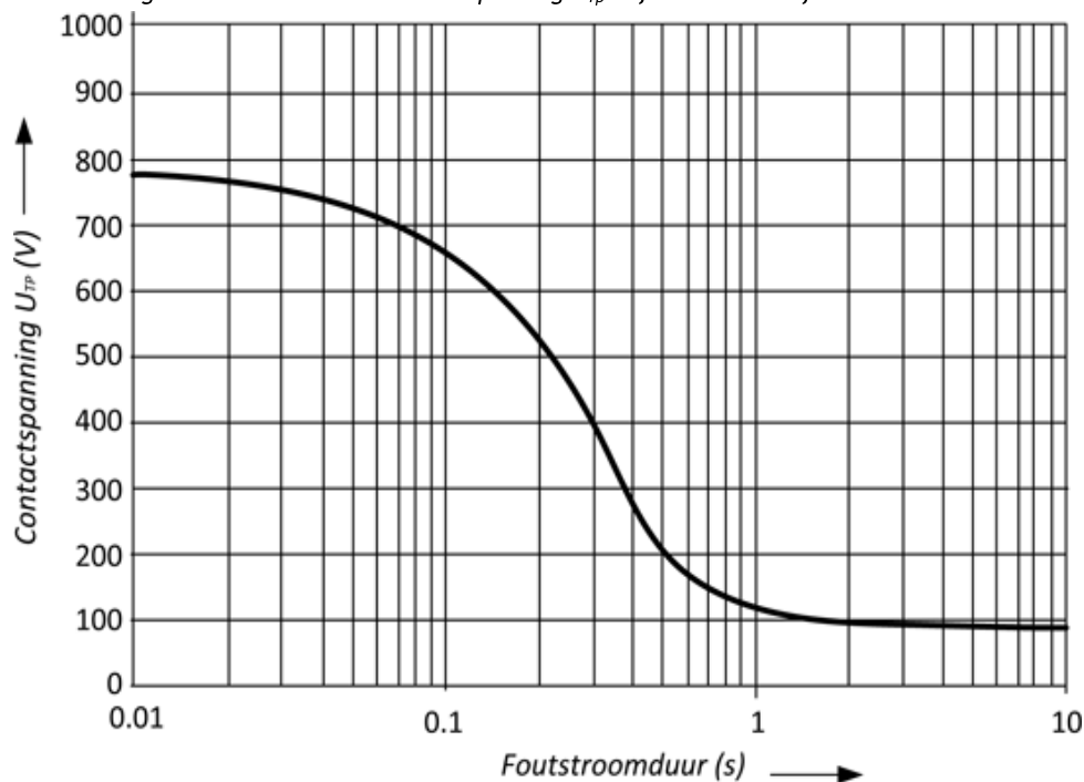
Figuur 2.1. Toelaatbare contactspanning U_{Tp} in functie van de foutstroomduur
