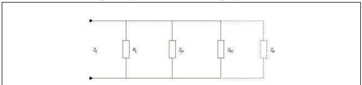
Figuur 2.9. Equivalent schema van de aardingsimpedantie Z_E
