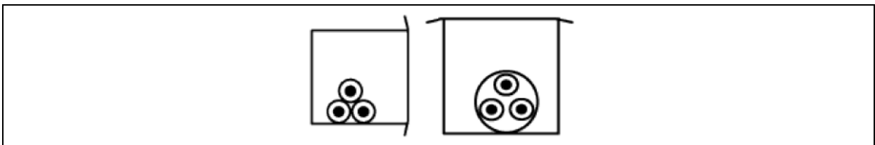
Figuur 2.16. Plaatsingswijze «kabelbaan»
