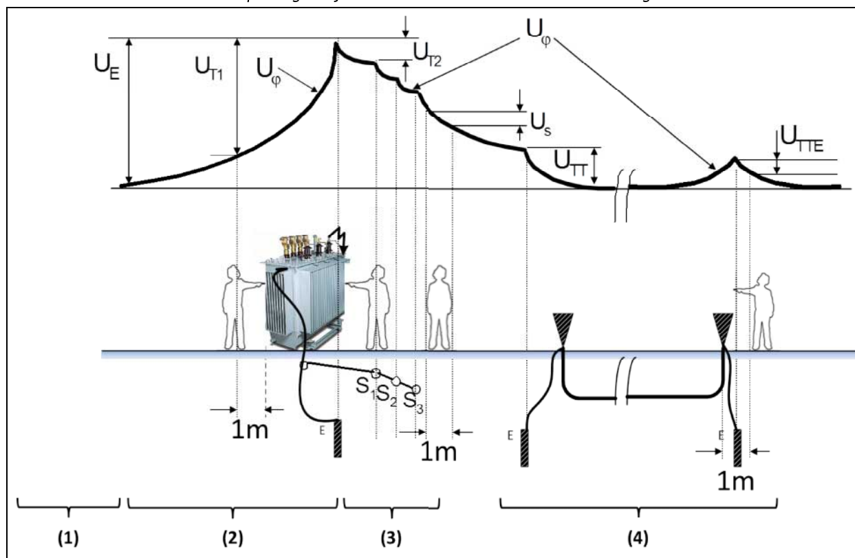
Figuur 2.6. Voorbeeld van verandering van aardbodemspansing en van spanningen bij het vloeien van stroom in de aardverbindingen
