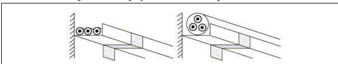
Figuur 5.5. Plaatsingswijzen van elektrische leidingen – Kabelrekken
