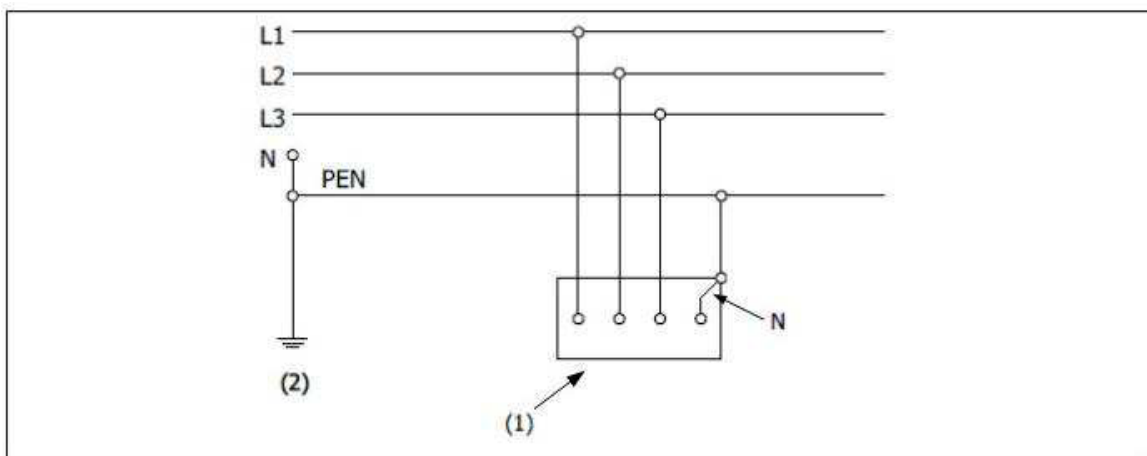
Figuur 2.2. TN-C-systeem
