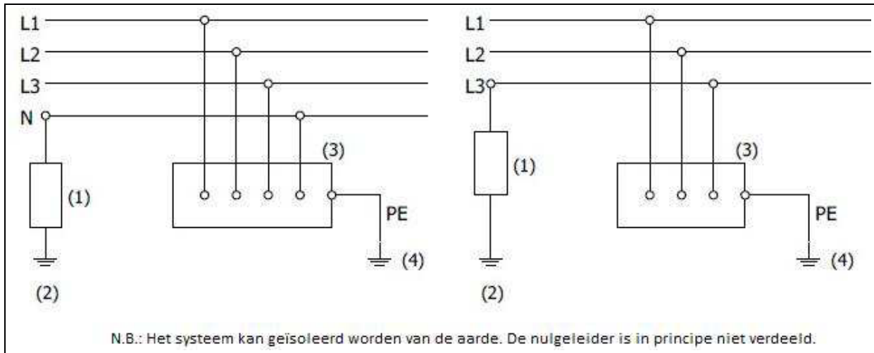
Figuur 2.5. IT-systeem
