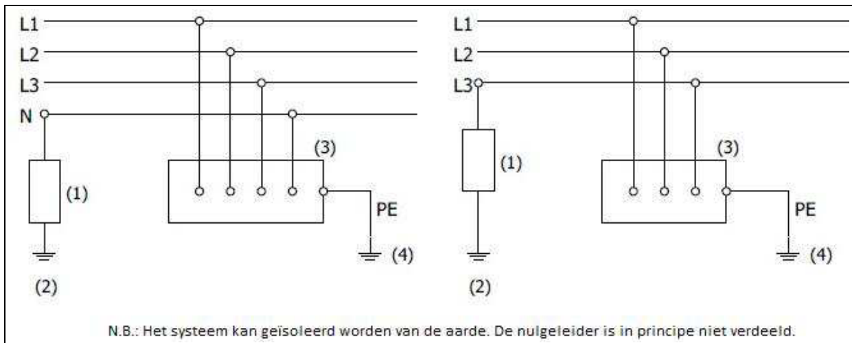
Figuur 3.5. IT-net
