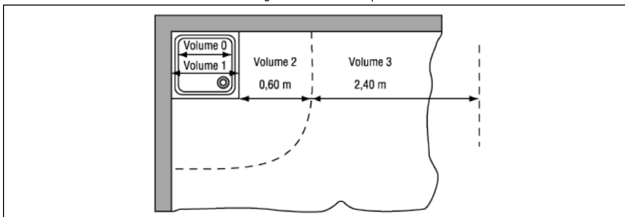
Figuur 7.3. Stortbadkuip
