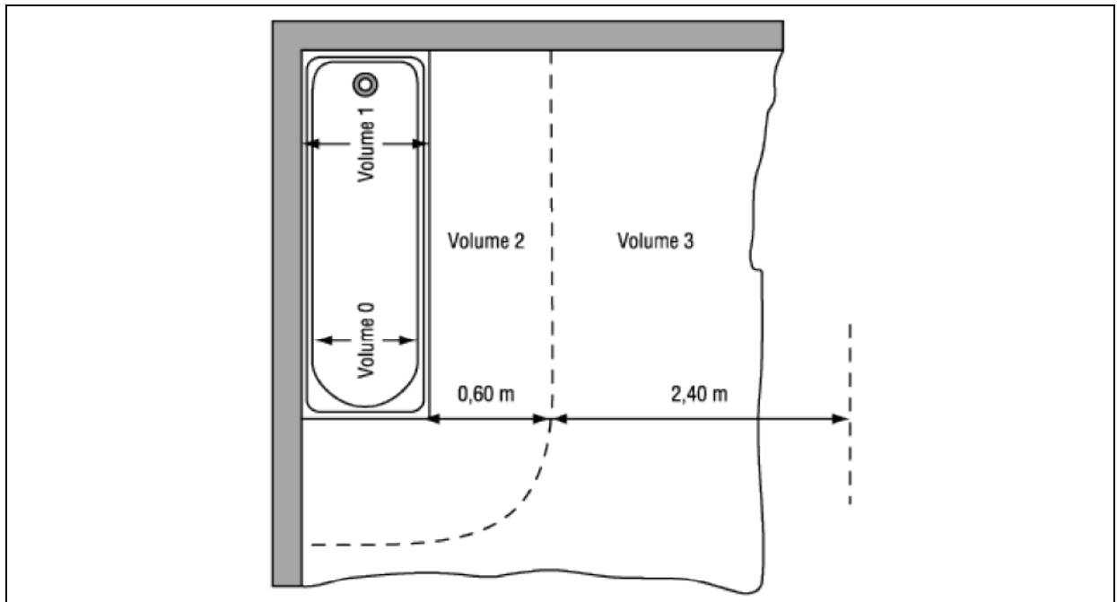
Figuur 7.1. Badkuip
