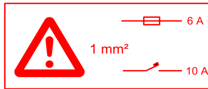
Figuur 8.1. Aanduiding van een stroombaan met een doorsnede kleiner dan 1,5 \text{ mm}^2
