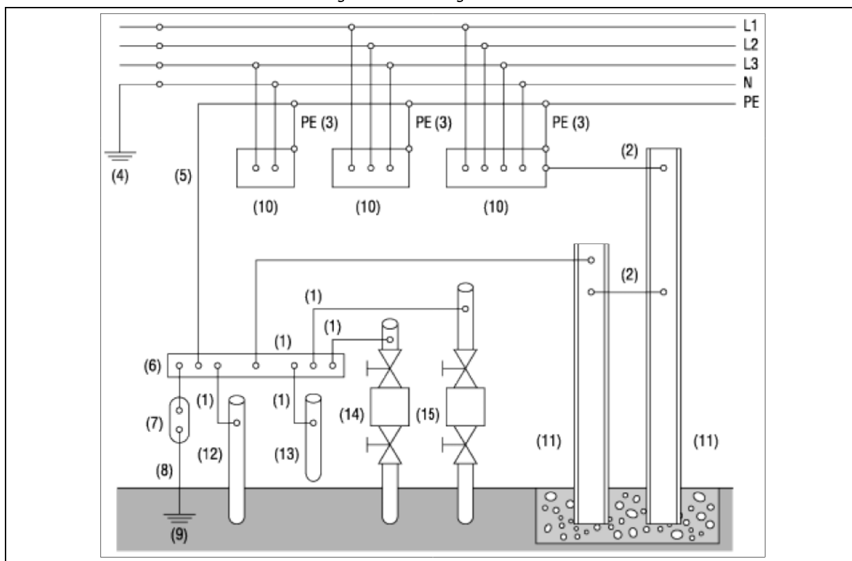
Figuur 2.10. Aardingsinstallatie
