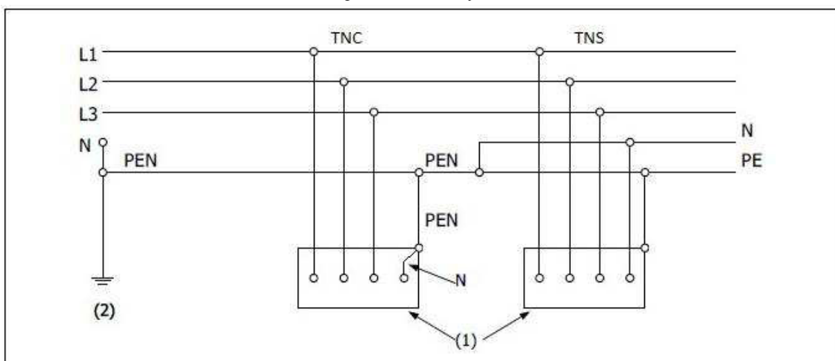
Figuur 2.3. TN-C-S-systeem
