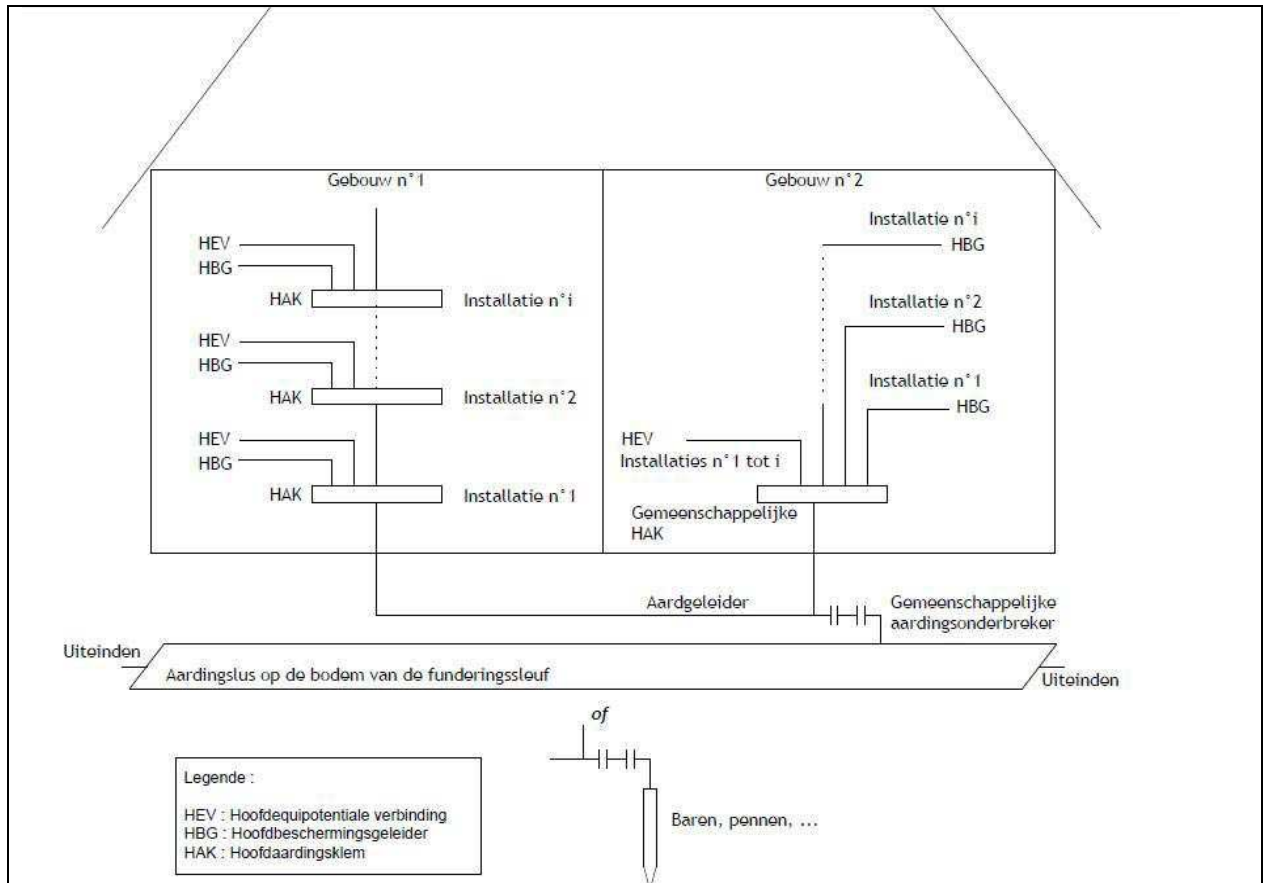
Figuur 5.32. Principeschema van de gemeenschappelijke aardverbinding (Gevalen bedoeld in punt c.1. 1 ste en 2 de alinea)
