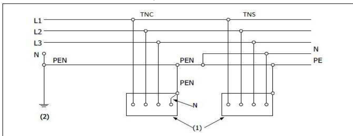
Figuur 3.3. TN-C-S-net
