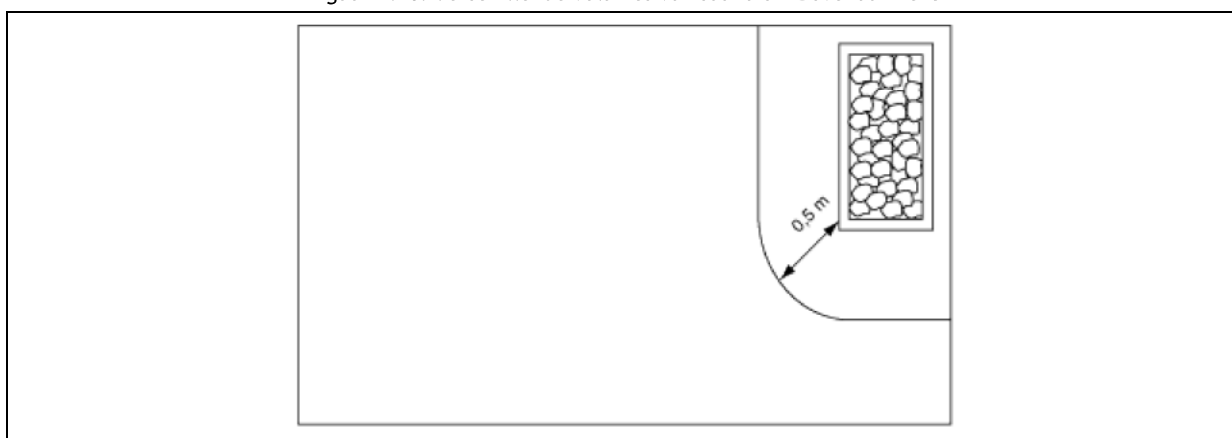
Figuur 7.16. Verschillende volumes van sauna's – Boveenaanzicht
