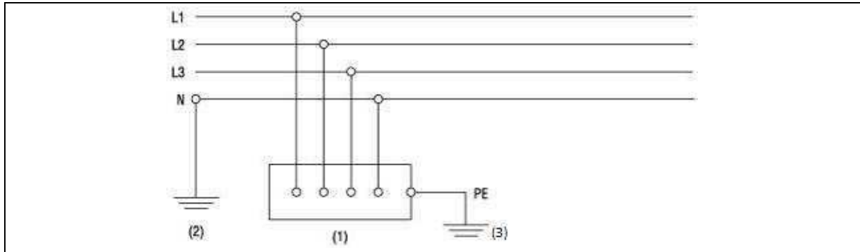
Figuur 3.4. TT-net
