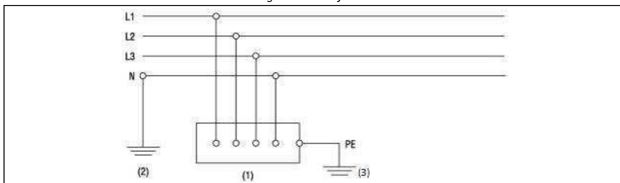
Figuur 2.4. TT-systeem
