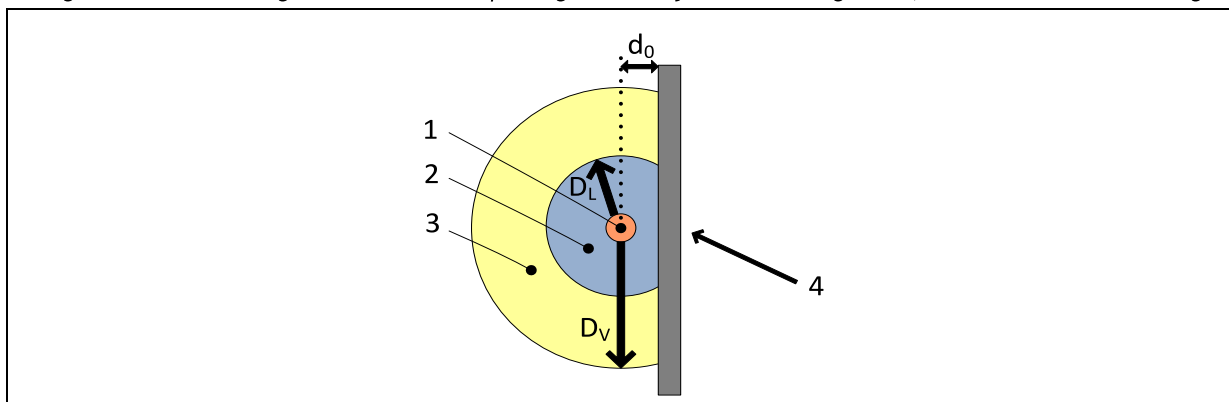
Figuur 2.23. Voorstelling van de zone onder spanning en de nabijheidszone met gearde, metalen bescherming
