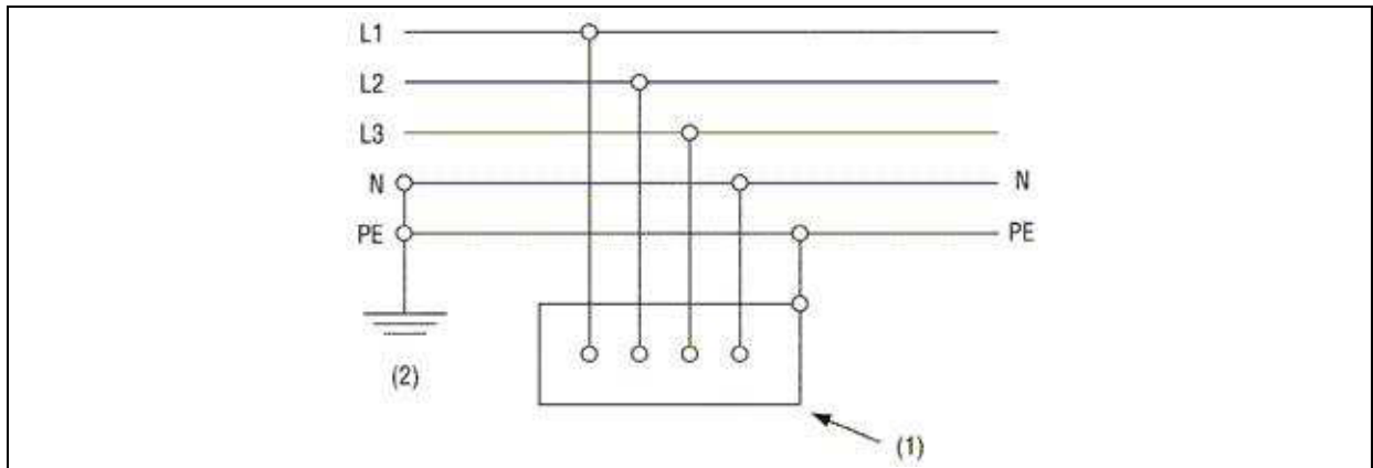
Figuur 2.1. TN-S-systeem
