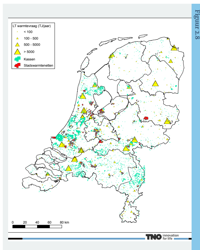
Figuur 2.8 Lage temperatuur (LT) warmtevraag. Bron: RVO WarmteAtlas (warmtenetten en LT-industrie), Top10 Vector (kassen).
