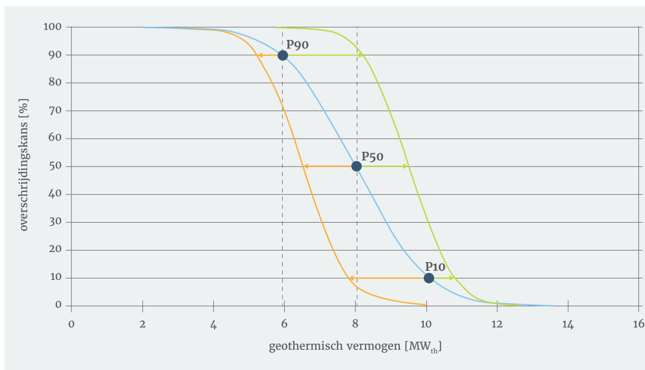
Figuur 3.9 Verandering van de verwachtingscurve van het vermogen van een doublet als gevolg van toegenomen ondergrondgegevens en kennis. Blauwe curve: vóór exploratie. Rood: na exploratie met negatief resultaat – het verwachte vermogen neemt af. Groen: na aanboren met positief resultaat – het verwachte vermogen neemt toe. De onzekerheid is afgenomen wat zichtbaar is in een steilere curve.
