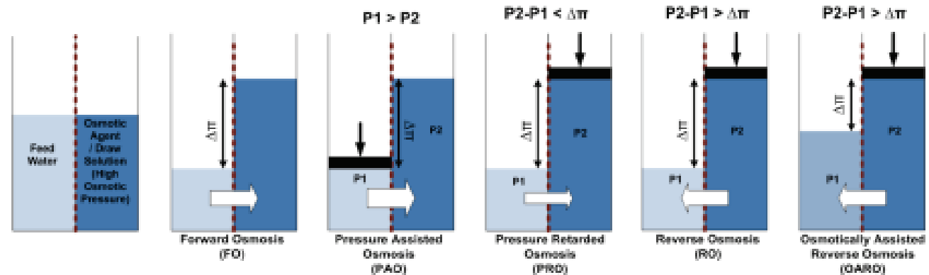
Figuur 2: Schematische weergave van osmotische processen
