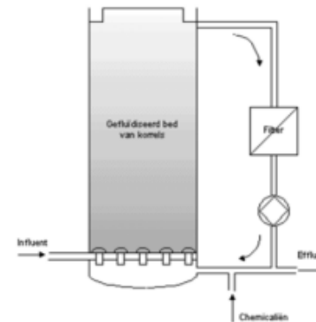
Figuur 9: Schematische weergave van vacuümverdamping WASS-Pelletkristallisatie/Korrelreactor
