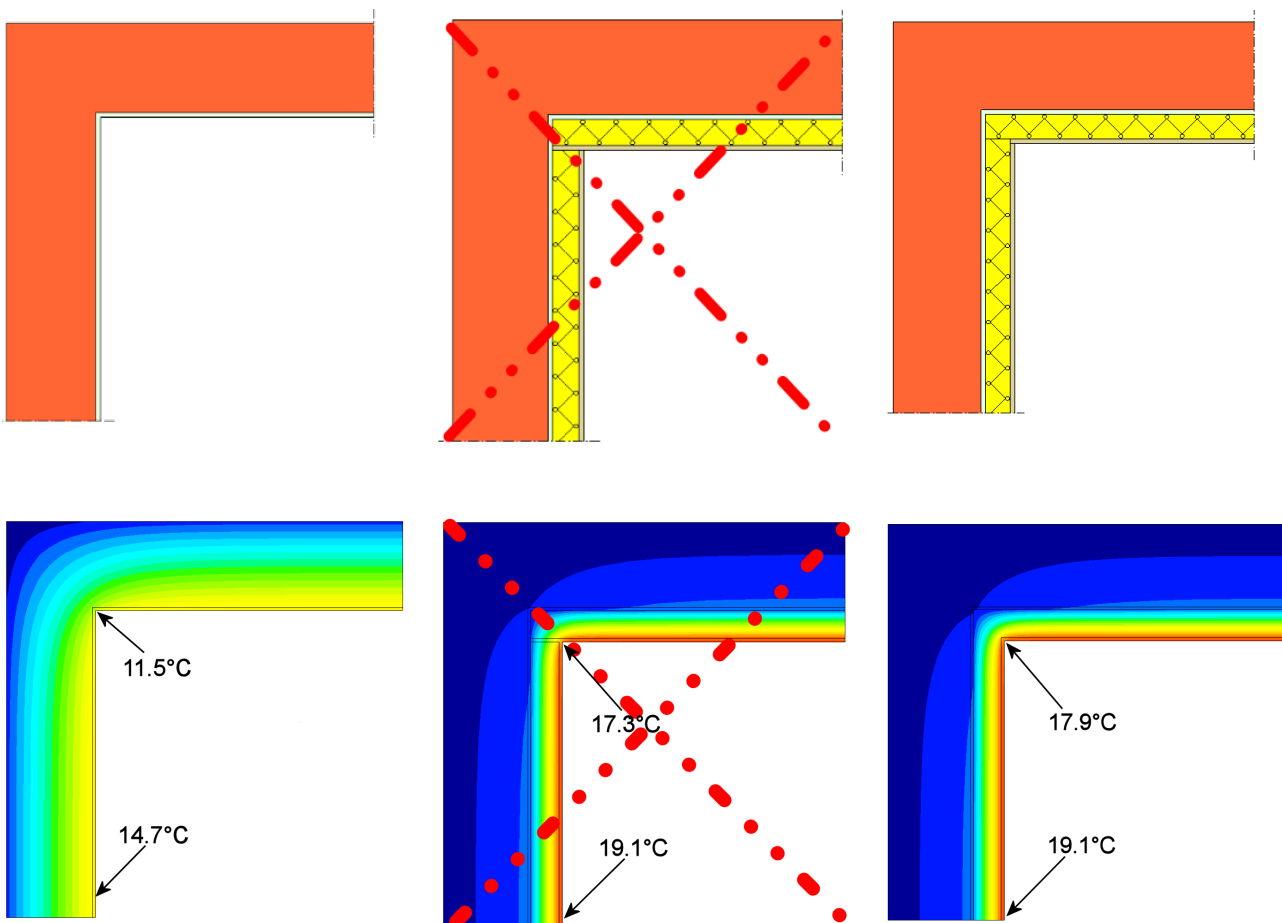
Figuur 39: Aansluiting van de isolatie op de plaats van een buitenhoek: de oorspronkelijke wand (links), de afgeraden opbouw met doorlopende binnenaafwerking (midden), en de aanbevolen opbouw zonder doorlopende binnenaafwerking (rechts).
