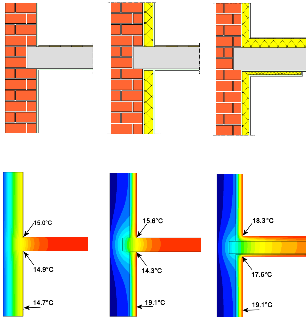
Figuur 42: Flankerende isolatie aan de bovenkant van de vloer, die leidt tot een verlaging van de oppervlaktetemperatuur in de hoek aan de onderkant.
