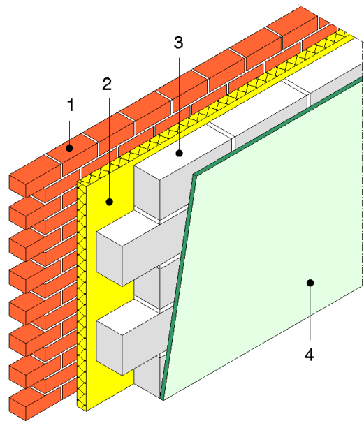
1. Metselwerk (buitenspouwblad); 2. Thermische isolatie; 3. Binnenspouwblad; 4. Binnenafwerking
