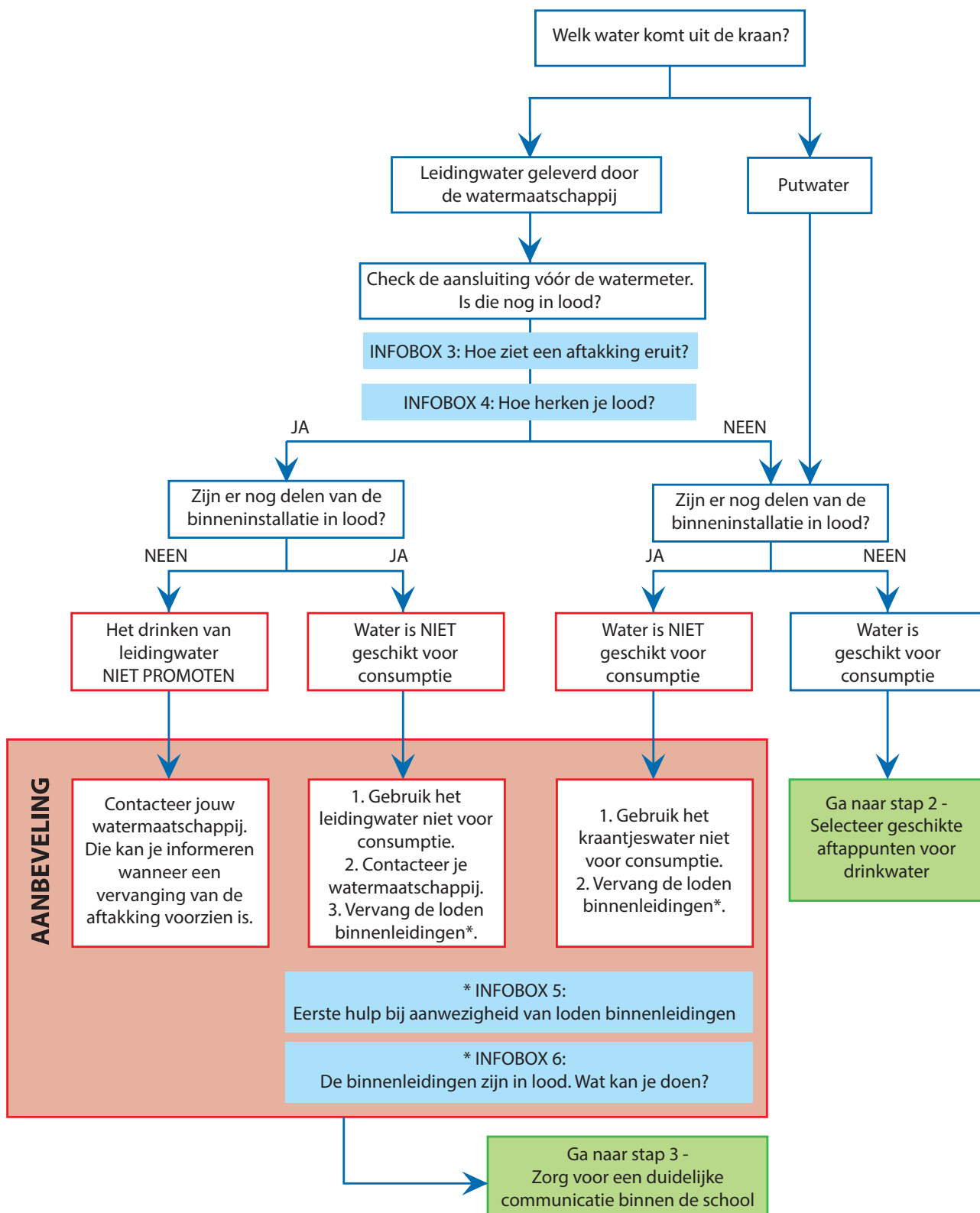
Figuur 2: Stroomschema loodvrije leidingen
